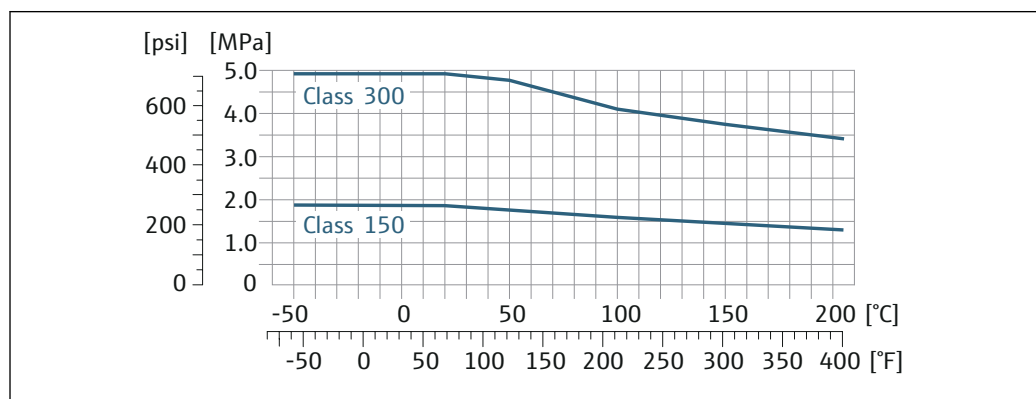
図 27 フランジ材質：1.4539 (SUS 890L 相当)；ラップジョイントフランジ (非接液)：1.4404 (SUS 316 または 316L 相当)
