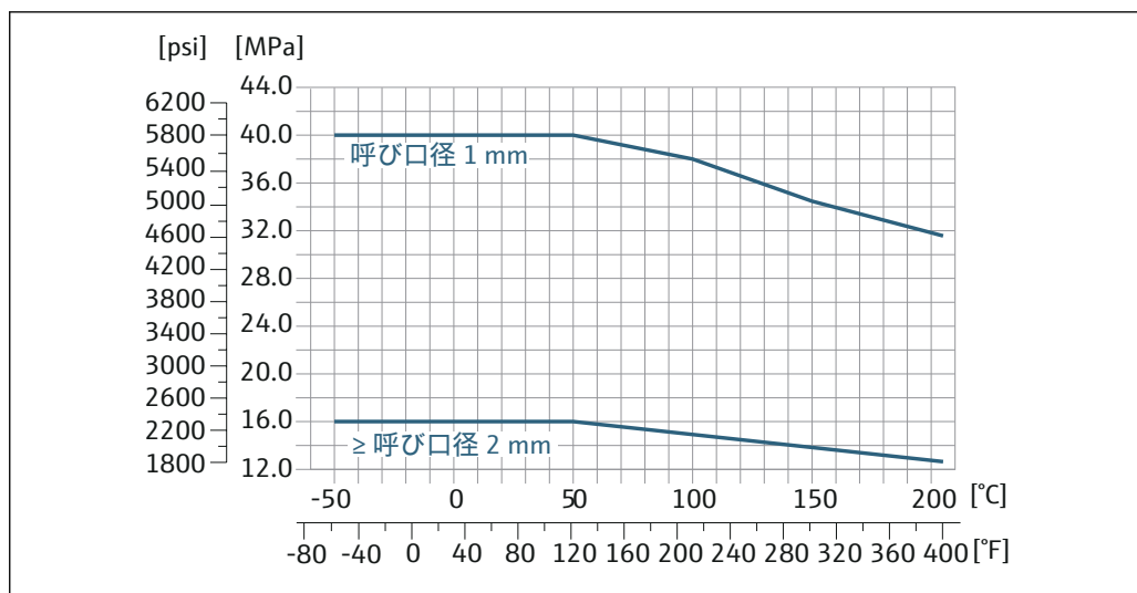
図 29 4-VCO-4 カップリング : 1.4539 (SUS 890L 相当) ; 8-VCO-4 カップリング : 1.4539 (SUS 890L 相当) ; NPTF ネジ込み式アダプタ : 1.4539 (SUS 890L 相当)
