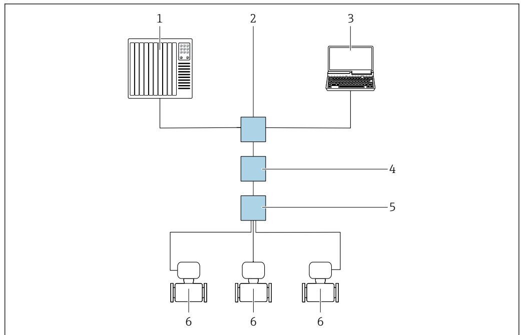
図 52 APL ネットワーク経由のリモート操作用オプション
