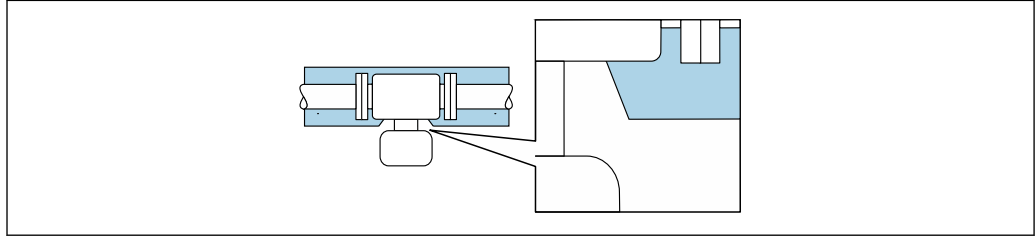
図 30 伸長ネックを覆わない断熱
