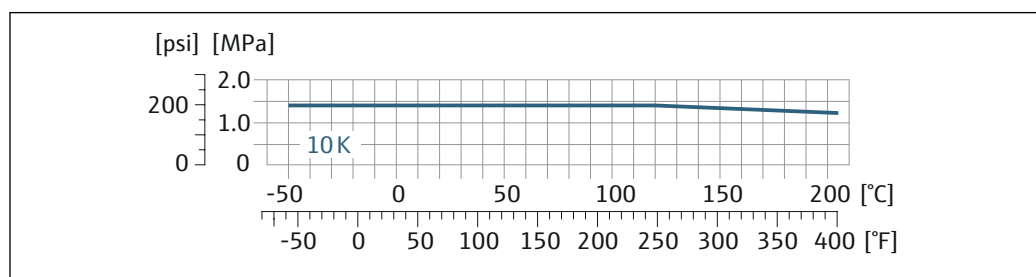
図 28 フランジ材質：1.4539 (SUS 890L 相当)；ラップジョイントフランジ (非接液)：1.4404 (SUS 316 または 316L 相当)
