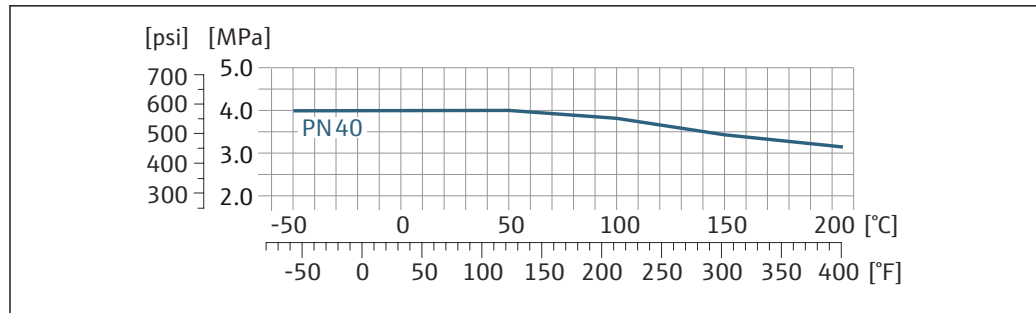
図 26 フランジ材質：1.4539 (SUS 890L 相当)、アロイ C22；ラップジョイントフランジ (非接液)：1.4404 (SUS 316 または 316L 相当)
