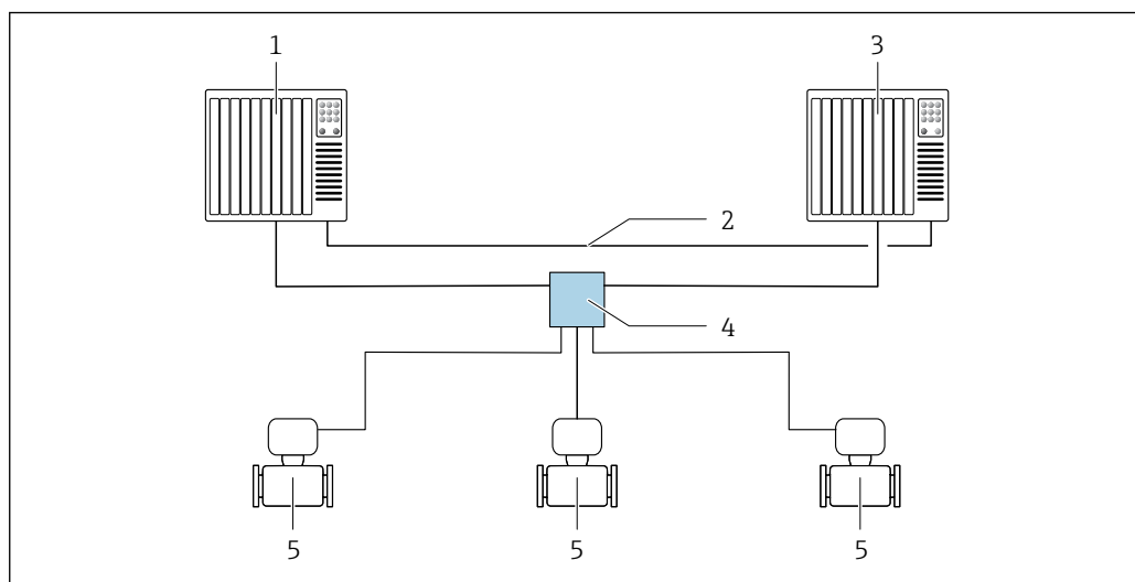
▣ 25 Przykład układu systemu redundantnego (S2): topologia gwiazdy
