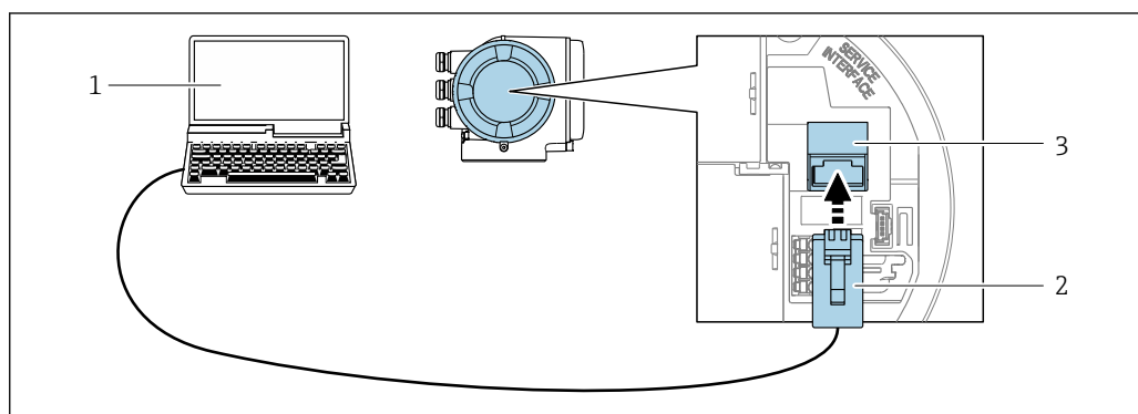
23 Podłączenie poprzez interfejs serwisowy (CDI-RJ45)
