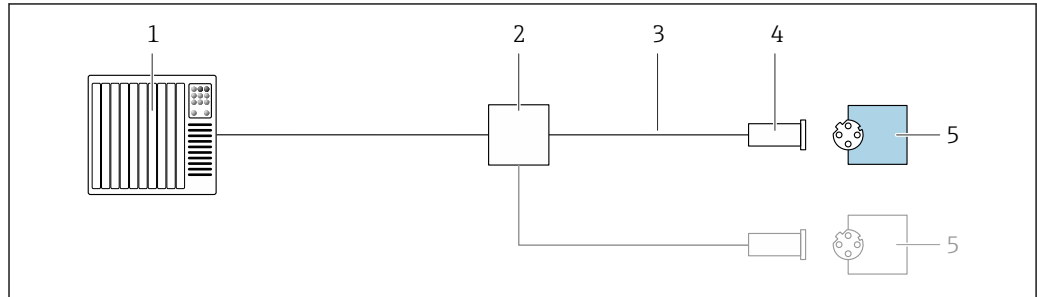
16 Przykład połączenia wersji PROFINET
