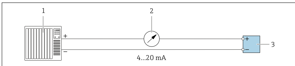
18 Przykład podłączenia wyjścia prądowego 4-20 mA (aktywnego)
