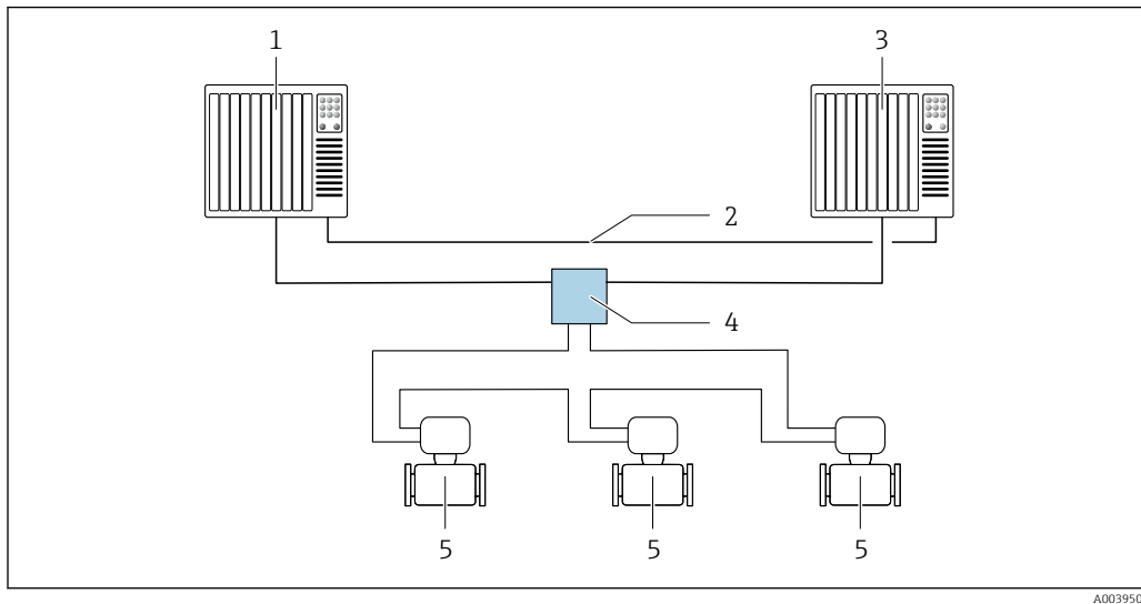
33 Przykład układu systemu redundanтного (S2): topologia pierścieniowa
