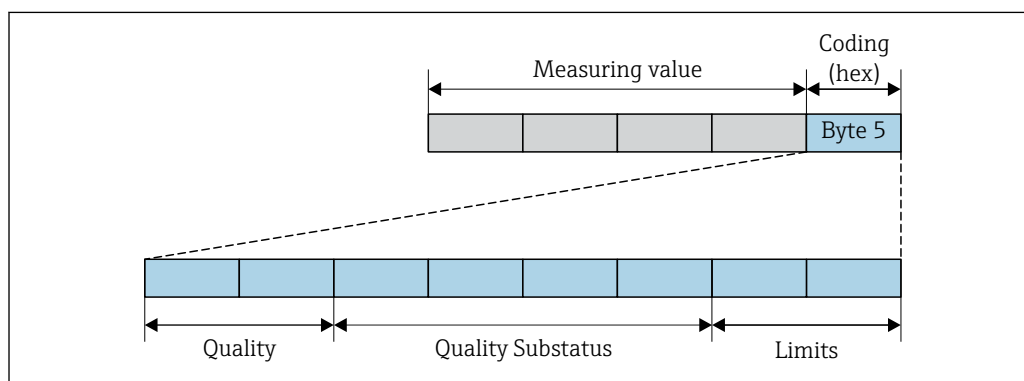
39 Struktura bajtu statusu
