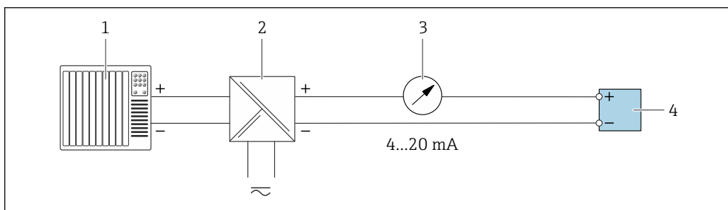
19 Przykład podłączenia wyjścia prądowego 4-20 mA (pasywnego)
