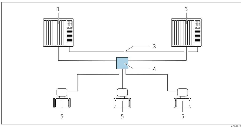
34 Przykład układu systemu redundanтного (S2): topologia gwiazdy
