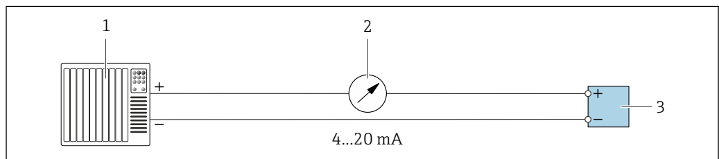
12 Przykład podłączenia wyjścia prądowego 4-20 mA (aktywnego)
