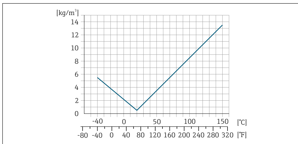
35 Kalibracja gęstości w warunkach procesowych, np. w temperaturze +20°C (+68°F)
