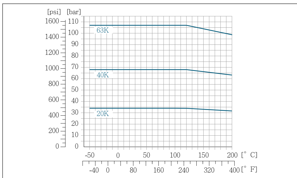
31 Avec matériau de bride : 1.4404 (316/316L) ou Alloy C22, 2.4602 (UNS N06022)
