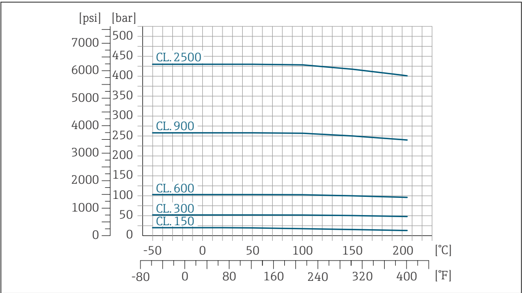
29 Avec matériau de bride : Alloy C22, 2.4602 (UNS N06022)
