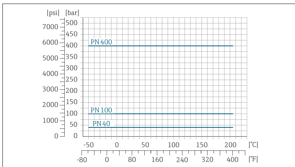
26 Avec matériau de bride : Alloy C22, 2.4602 (UNS N06022)
