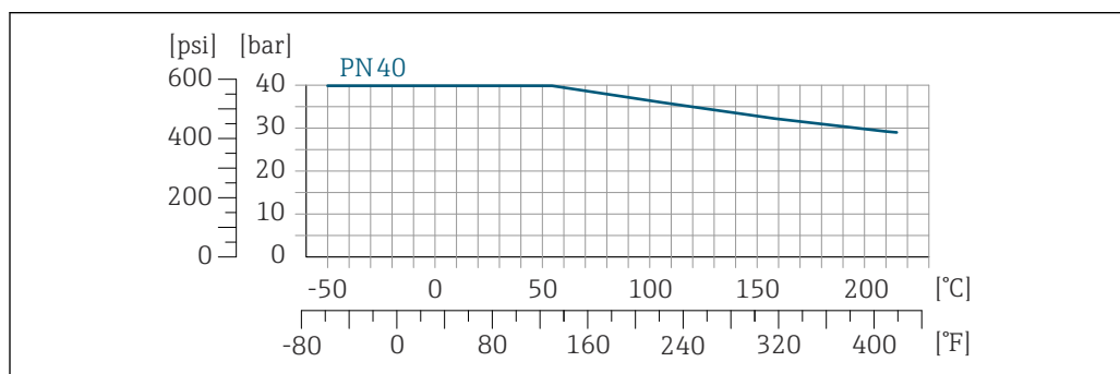
27 Bride tournante avec matériau de bride : 1.4301 (F304), parties en contact avec le produit Alloy C22: 2.4602 (UNS N06022)
