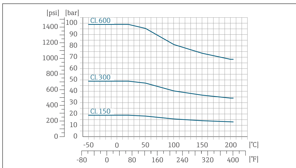
30 Bride tournante avec matériau de bride : 1.4301 (F304), parties en contact avec le produit Alloy C22: 2.4602 (UNS N06022)
