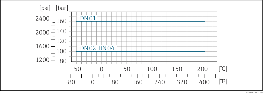
33 Avec matériau de bride 1.4404 (316/316L)
