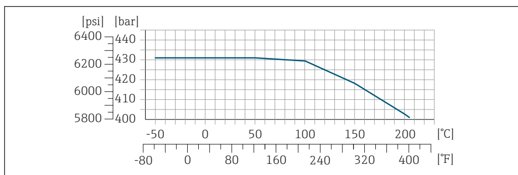
35 Avec matériau de bride : Alloy C22, 2.4602 (UNS N06022) ; caractéristique de commande "Mat. tube mesure, surface en contact", option HB
