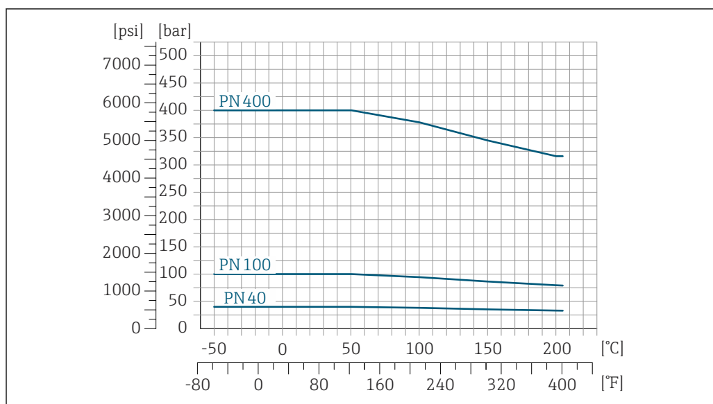
25 Avec matériau de bride 1.4404 (316/316L)
