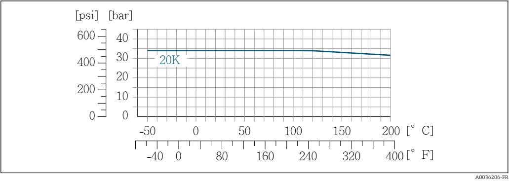
32 Bride tournante avec matériau de bride : 1.4301 (F304), parties en contact avec le produit Alloy C22: 2.4602 (UNS N06022)
