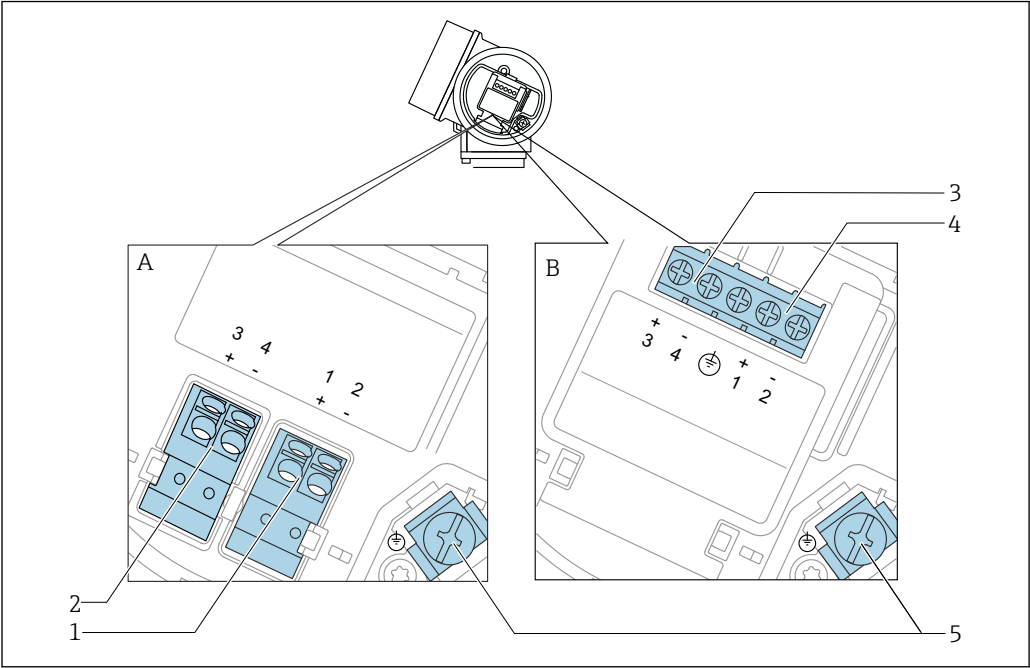
15 接线端子分配：两线制；4...20 mA HART，开关量输出
