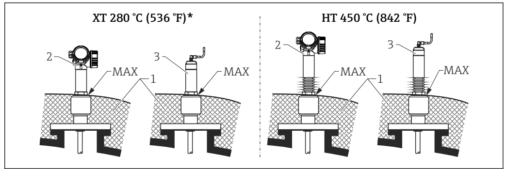
10 法兰过程连接 - 增温型 (XT) 和高温型 (HT) 仪表
