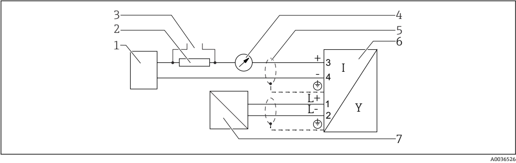
图 20 接线端子分配：四线制；4...20 mA HART (10.4 ... 48 V DC )
