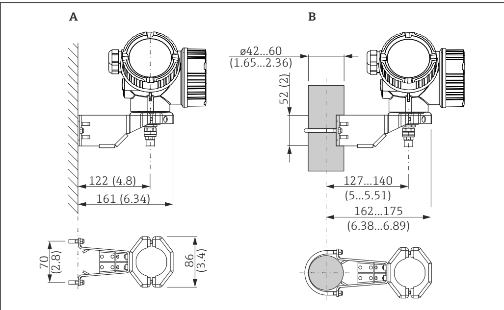
图 11 使用安装架安装电子腔外壳。测量单位 mm (in)
