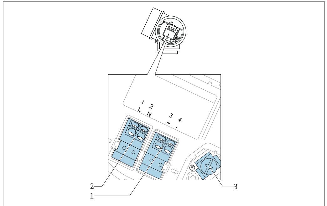
图 21 接线端子分配: 四线制; 4...20 mA HART (90 ... 253 V AC )
