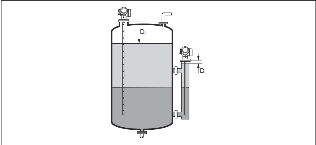
55 界面测量时的距离
