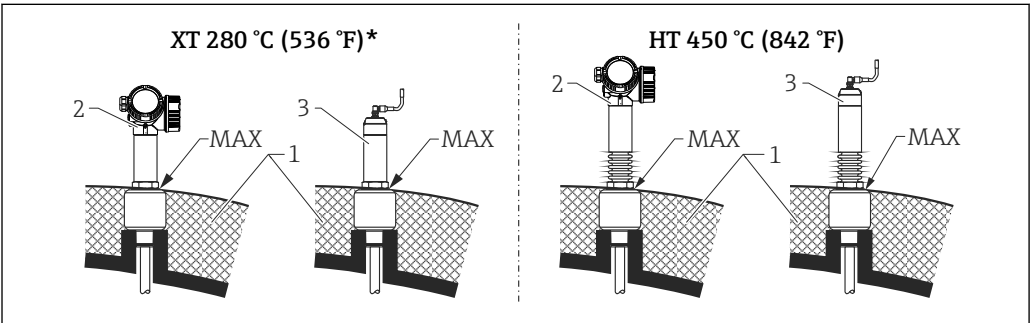
9 螺纹过程连接 - 增温型 (XT) 和高温型 (HT) 仪表
