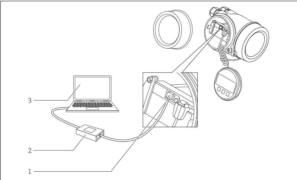
图 34 DeviceCare/FieldCare, 使用服务接口 (CDI)
