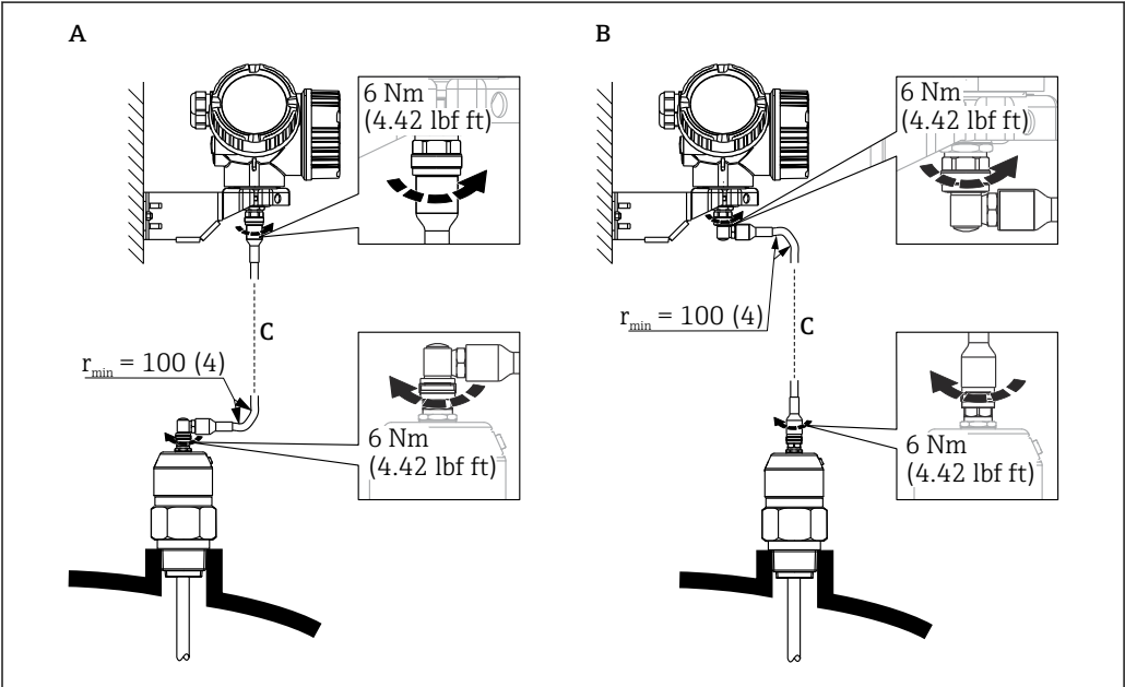
12 连接连接电缆。通过以下方式连接电缆：。测量单位 mm (in)
