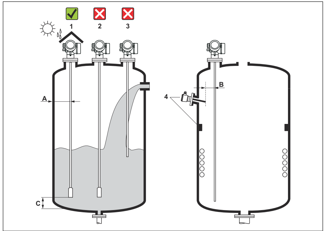
图 4 Levelflex 的安装条件
