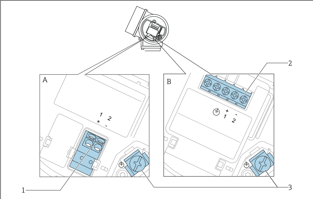
图 13 接线端子分配: 两线制; 4...20 mA HART
