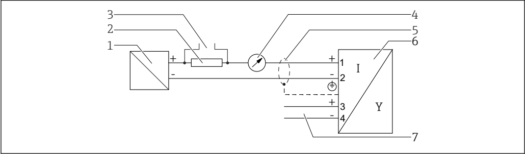
16 接线图：两线制；4...20 mA HART，开关量输出
