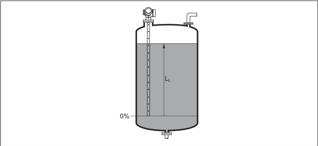
52 液位测量时的液位
