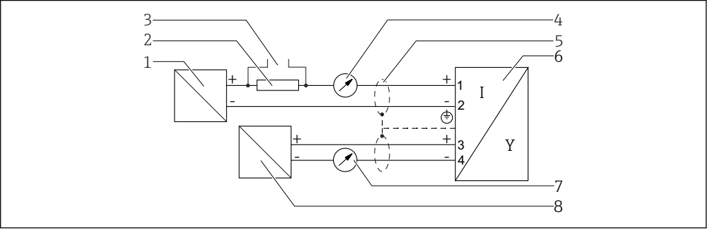
18 接线图: 两线制; 4...20 mA HART, 4...20 mA
