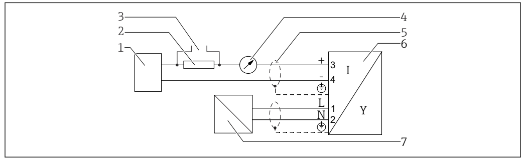
22 接线端子分配: 四线制; 4...20 mA HART (90 ... 253 V AC )
