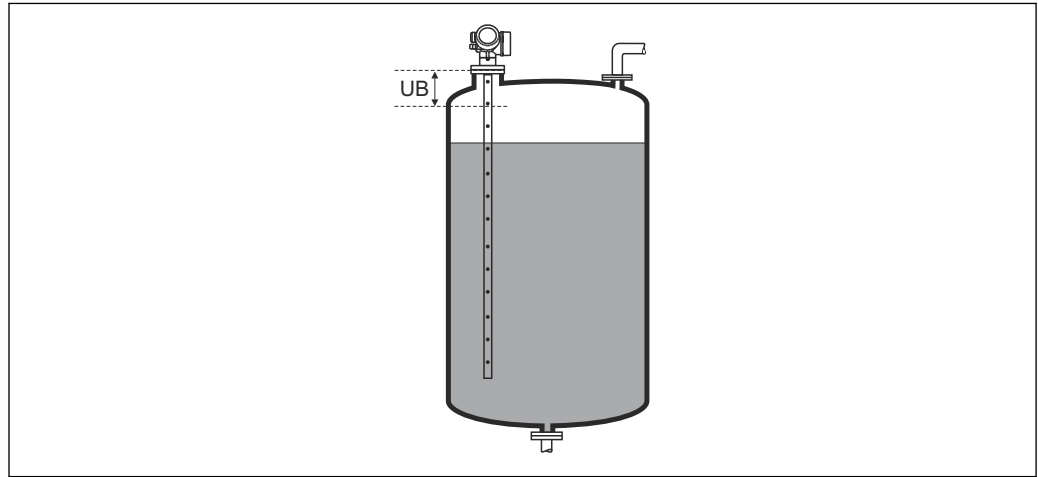
图 59 液位测量的盲区距离 (UB)
