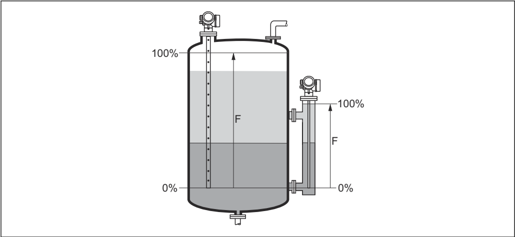
51 界面测量时的满标 (F)
