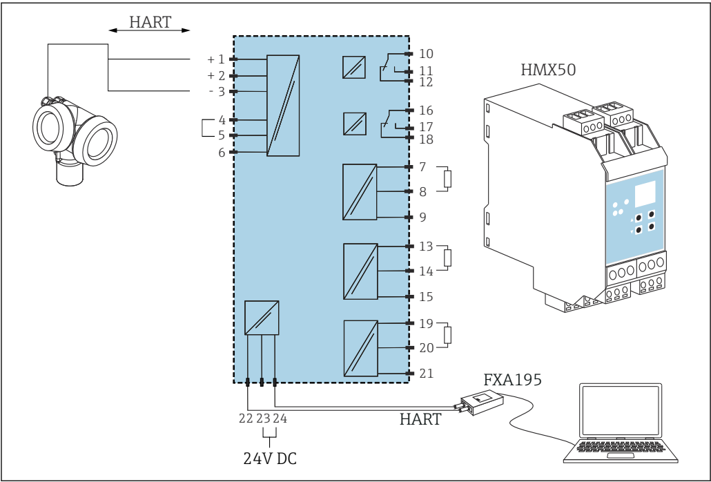
图 25 HART 回路转换器 HMX50 的接线图 (图例：无源两线制设备，连接电流输出，用作电源)
