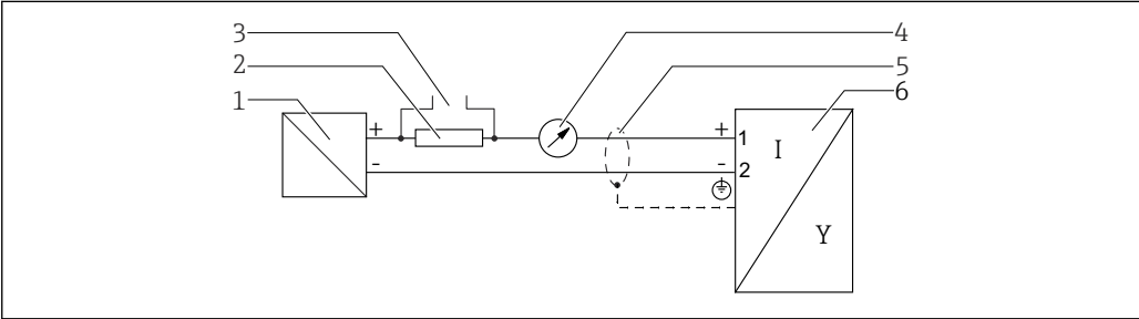
图 14 接线图: 两线制; 4...20 mA HART
