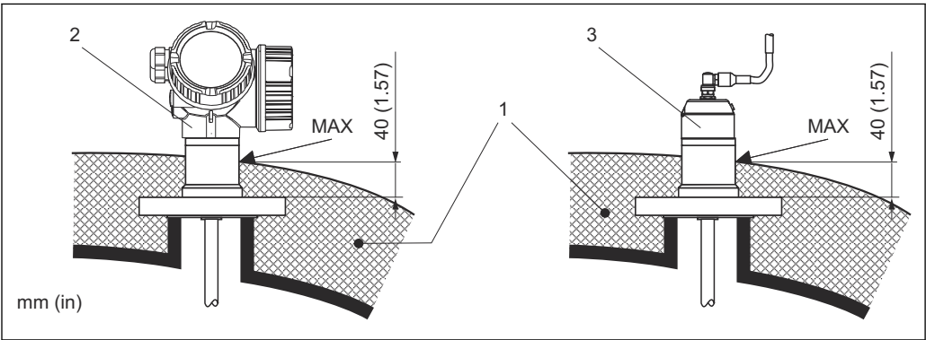
8 法兰过程连接
