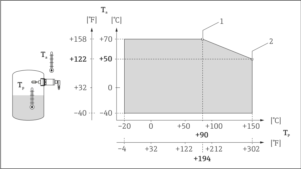
18 Courbe pour capteur 150 °C (302 °F)
