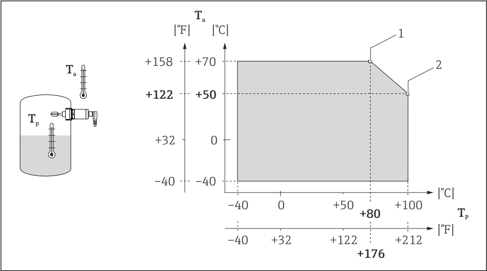
17 Courbe pour capteur 100 °C (212 °F)
