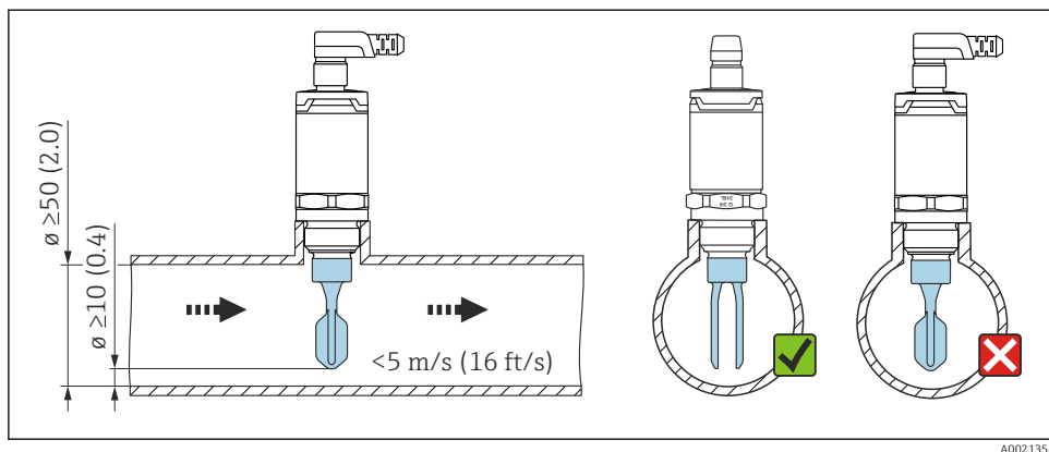
8 Position des lames vibrantes dans les conduites. Unité de mesure mm (in)
