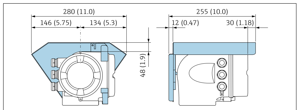
30 Capot de protection pour Proline 500 ; unité de mesure mm (in)
