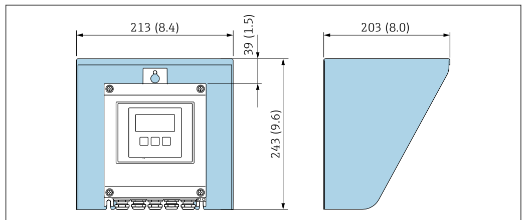
29 Capot de protection climatique pour Proline 500 – numérique ; unité de mesure mm (in)
