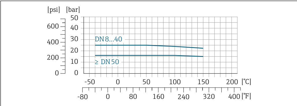
35 Avec matériau de bride 1.4404 (316/316L)
