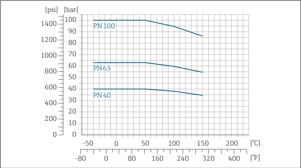
32 Avec matériau de bride 1.4404 (F316/F316L)
