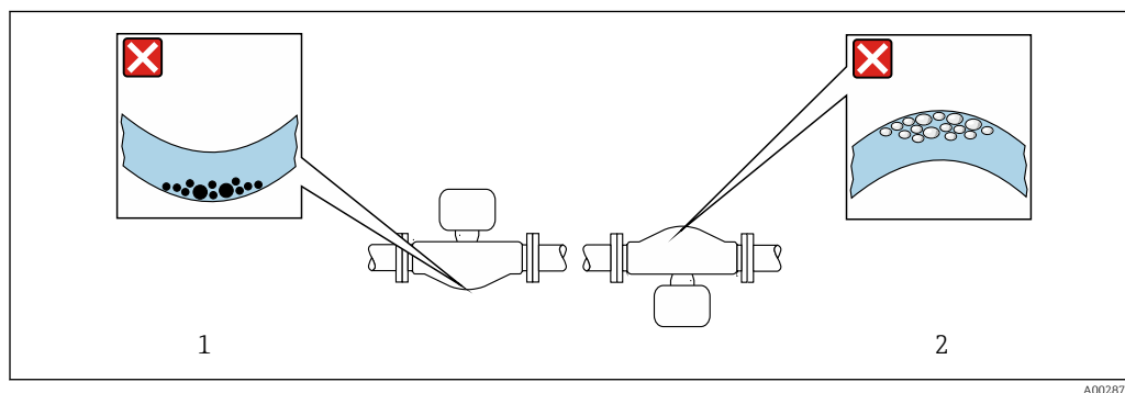
24 Position du capteur avec tube de mesure coudé
