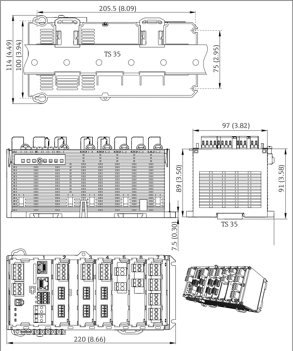
31 Dimensions en mm (inch)
