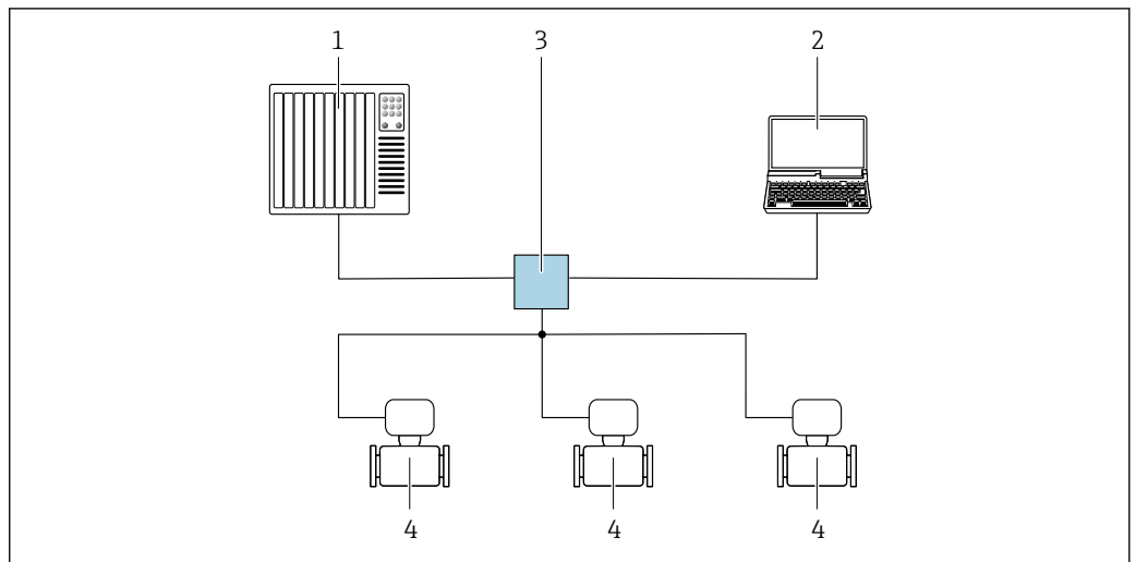
54 Opções para operação remota através da rede PROFIBUS: topologia estrela
