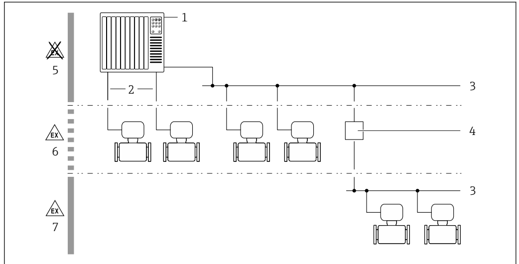
1 Possibilidades para integração de medidores em um sistema
