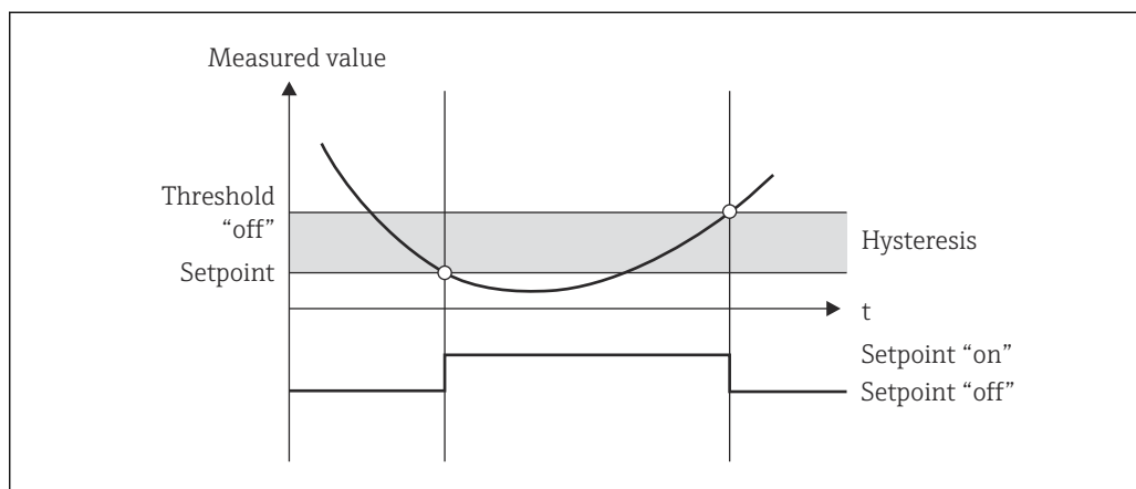
9 Режим работы Min
