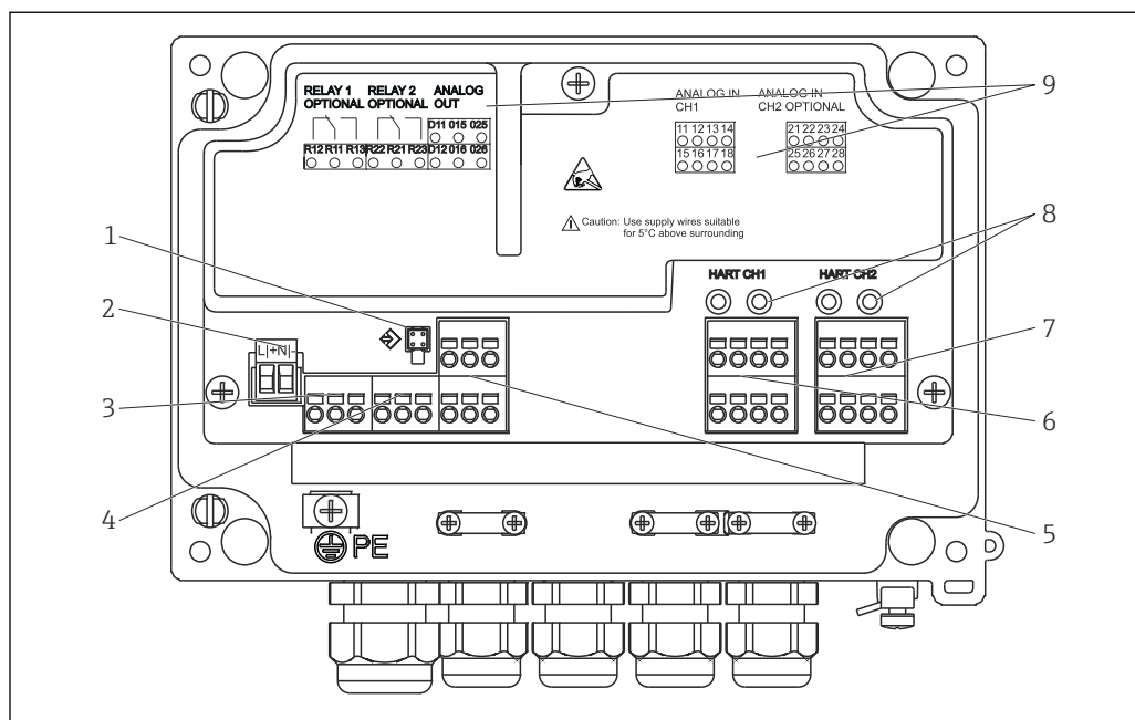
18 Вид изнутри и назначение клемм индикатора процесса
