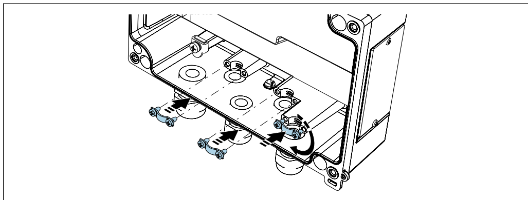
6 Соединение для заземления экрана
