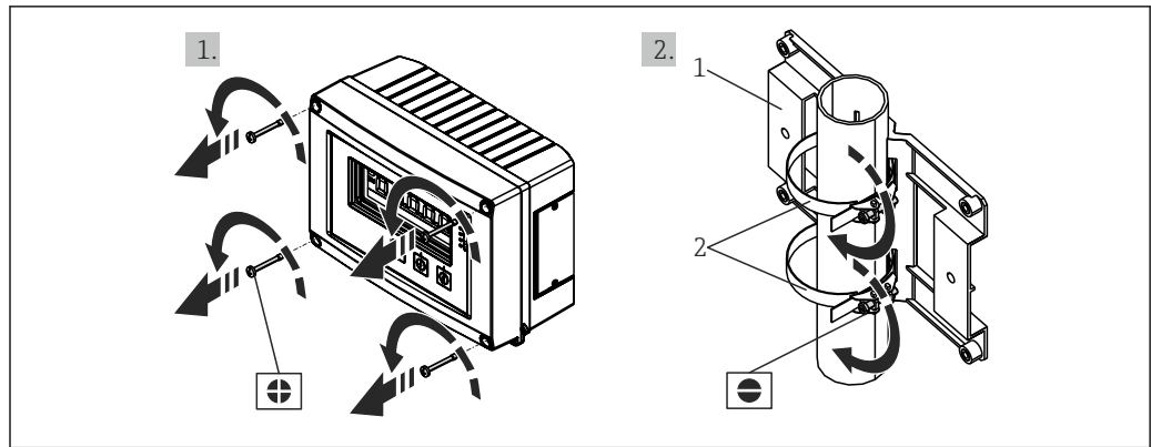
2 Монтаж полевого индикатора на трубопроводе
