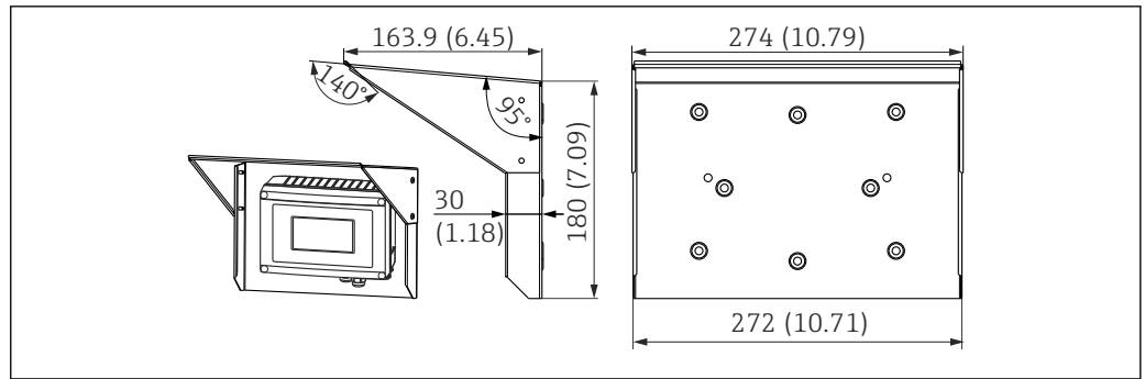
21 Размеры в мм (дюймах)
