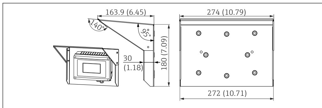
17 Размеры в мм (дюймах)
