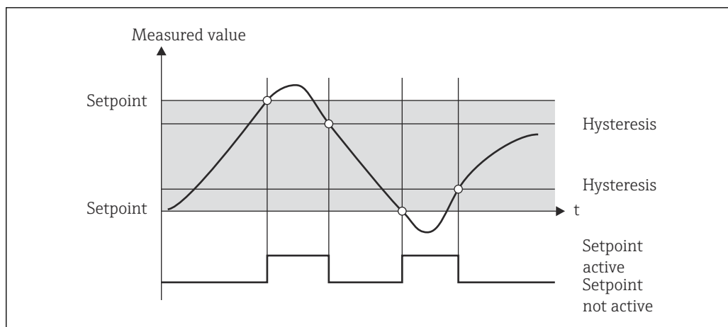
13 Режим работы InBand
