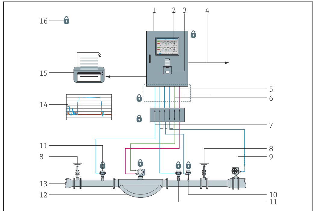
2 Systemaufbau des Bunker-Messsystems
