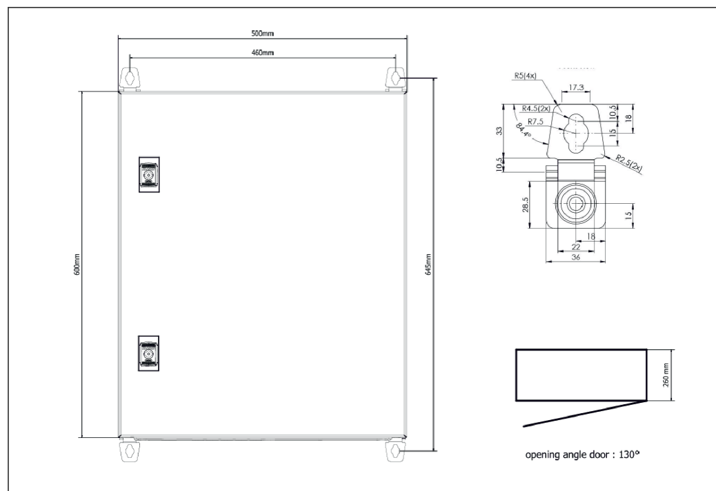
4 SPS (Steuereinheit) in einem Schaltschrank
