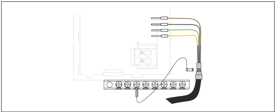
17 Morsettiera
