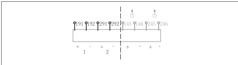
22 Assegnazione degli ingressi binari 1 e 2
