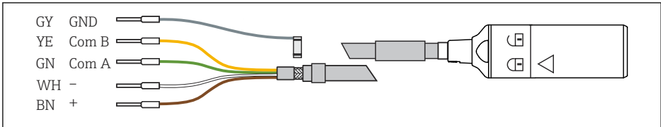
16 Esempio di cavo dati Memosens CYK10
