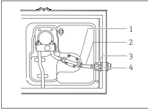
12 Tubo di aspirazione collegato lateralmente (stato alla consegna)
