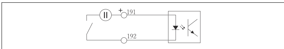
23 Ingresso binario con generatore di tensione esterno
