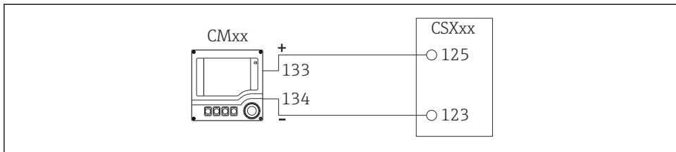
20 Con trasmettitore a 2 fili, ad es. Liquiline M CM42
