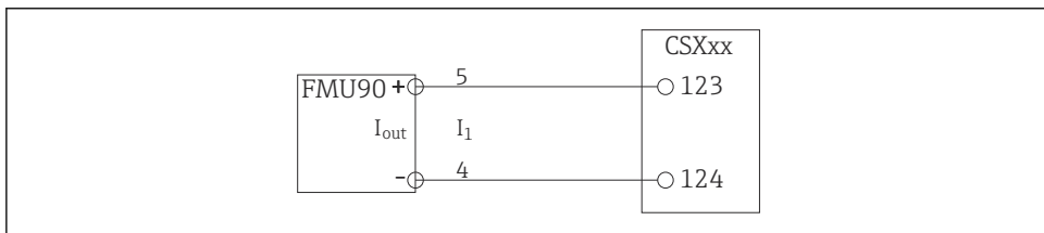
21 Con trasmettitore a 4 fili, ad es. Prosonic S FMU90
