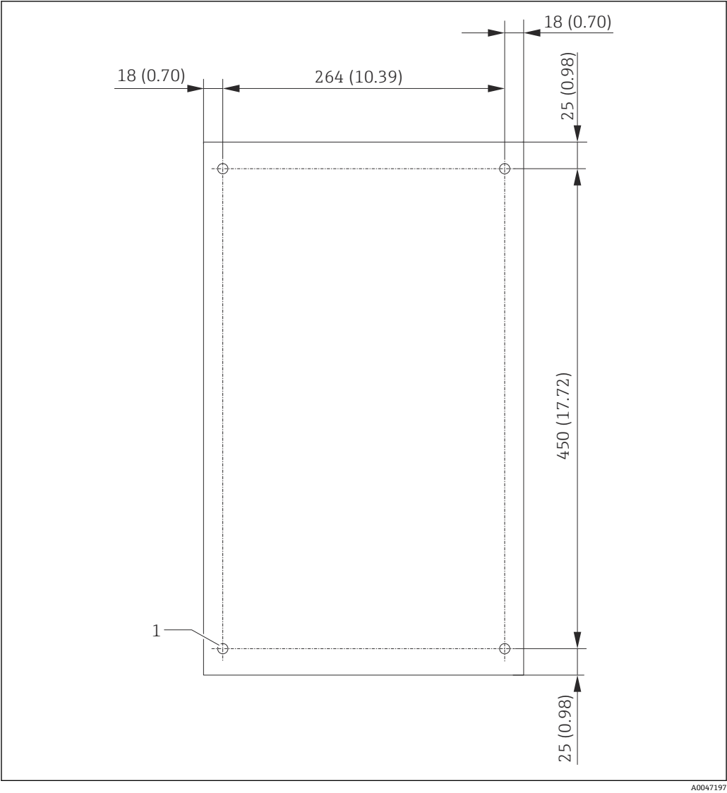
图 2 仪表外壳后视图 1 拉铆螺母
