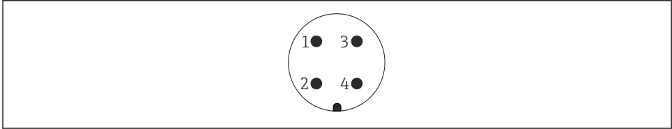
5 Affectation des broches du connecteur 7/8"
