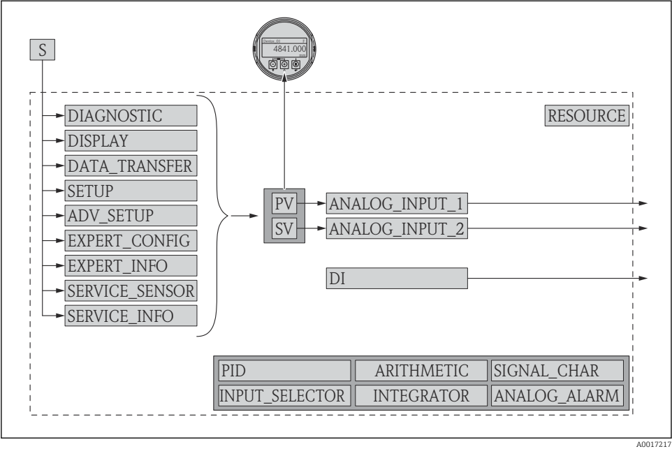
9 Configuration des blocs à la livraison
