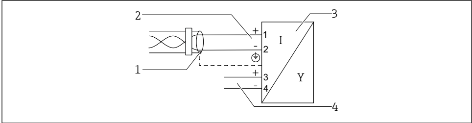
4 Schéma de principe PROFIBUS PA / FOUNDATION Fieldbus
