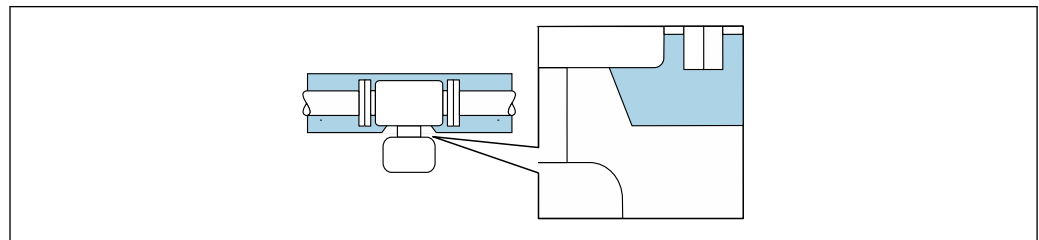
7 Неприменение теплоизоляции удлинительной шейки
