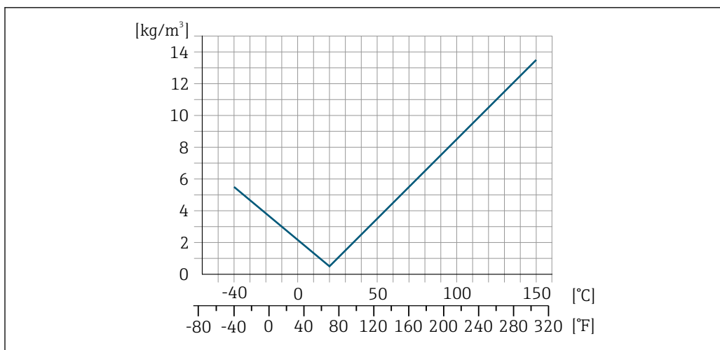
39 Калибровка по плотности на месте эксплуатации, в примере – при температуре +20 °C (+68 °F)
