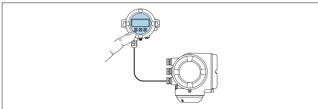
43 Управление с помощью выносного блока управления и дисплея DKX001
