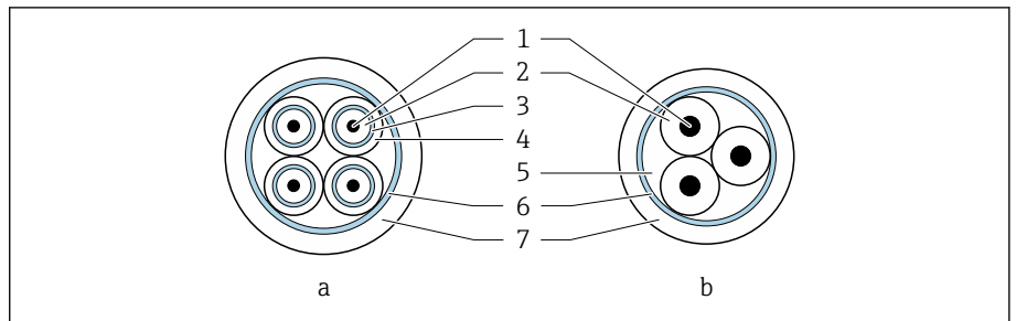
9 Поперечное сечение кабеля
