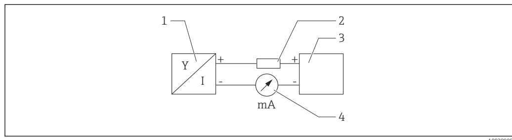
2 Diagrama de bloques de la conexión HART
