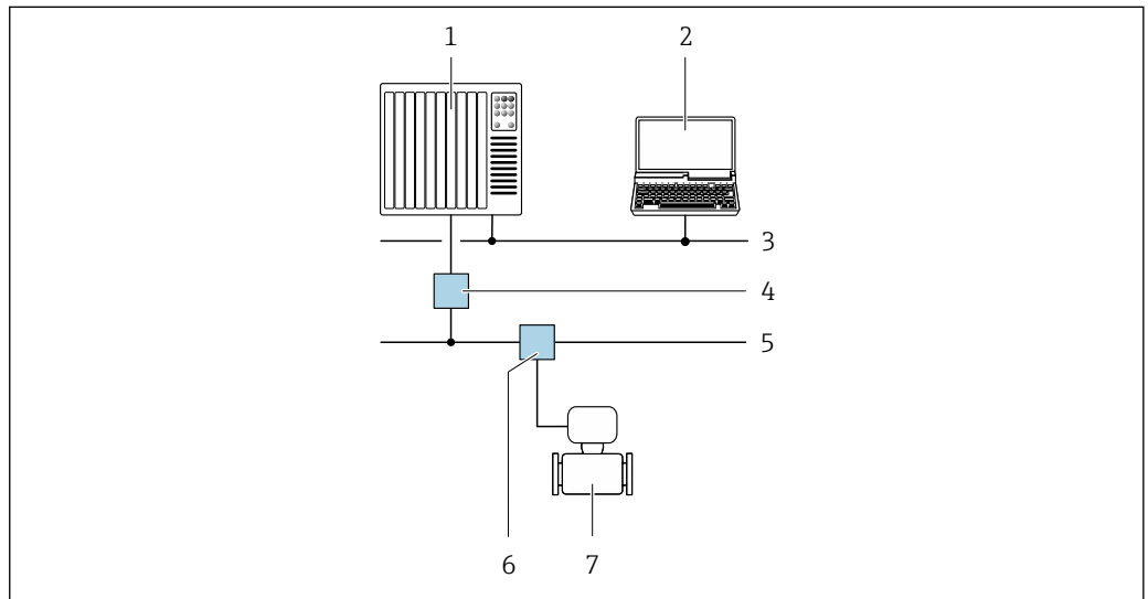
68 Opciones para la configuración a distancia mediante red PROFIBUS PA
