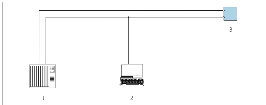
69 Opciones para la configuración a distancia mediante el protocolo Modbus-RS485 (activo)
