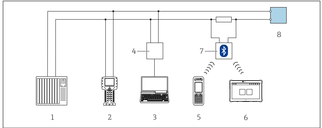
64 Opciones para la configuración a distancia mediante el protocolo HART (activo)
