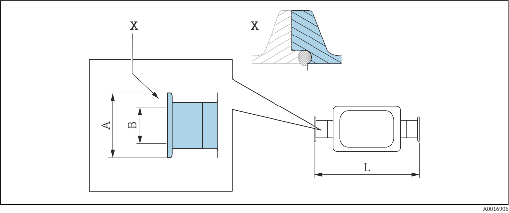
46 Detalle X: conexión a proceso asimétrica; la parte representada en azul la proporciona el proveedor.
