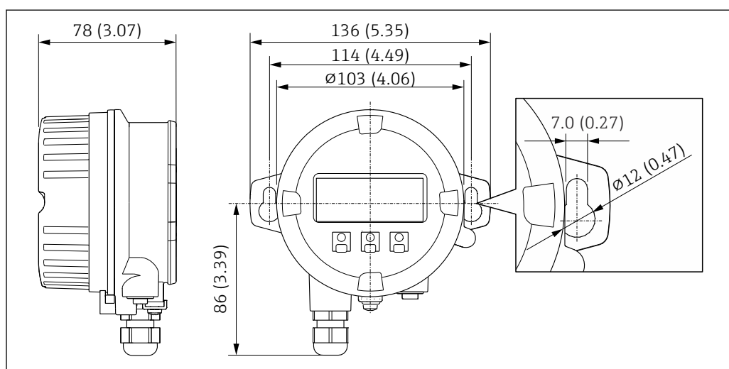
58 Unidad física mm (in)
