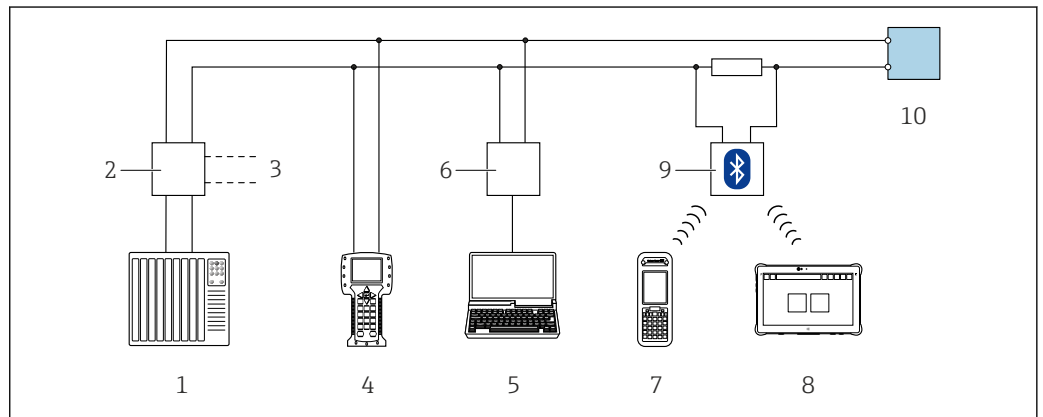
65 Opciones para la configuración a distancia mediante el protocolo HART (pasivo)
