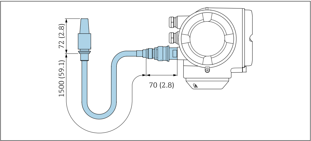
60 Unidad física mm (in)
