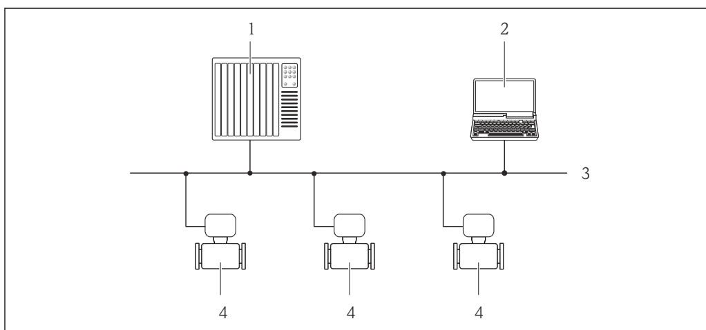
67 Opciones para la configuración a distancia mediante red PROFIBUS DP
