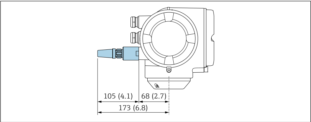
50 Unidad física mm (in)
