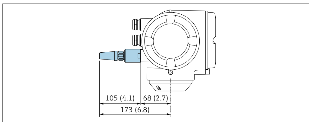
59 Unidad física mm (in)
