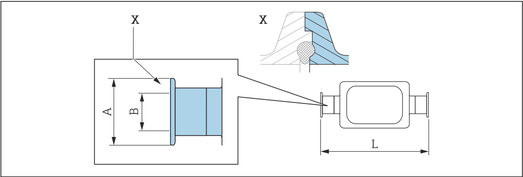
44 Detalle X: conexión a proceso asimétrica; la parte representada en azul la proporciona el proveedor.
