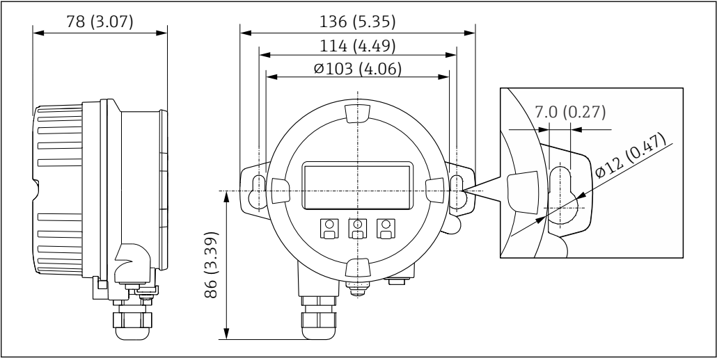
49 Unidad física mm (in)
