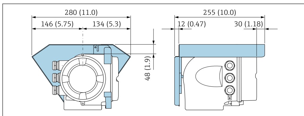
57 Unidad física mm (in)
