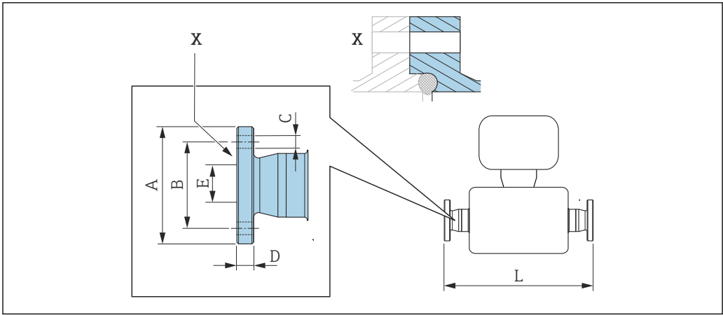
39 Detalle X: conexión a proceso asimétrica; la parte representada en azul la proporciona el proveedor.
