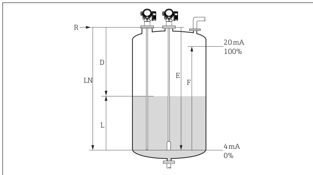
图 28 液位测量时的设置参数
