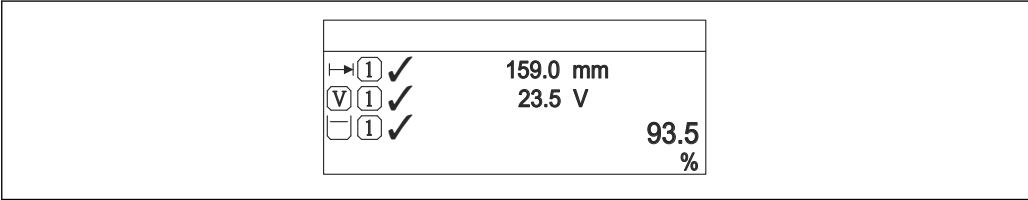
51 「表示形式」 = 「1 つの値はサイズ大 + 2 つの値」
