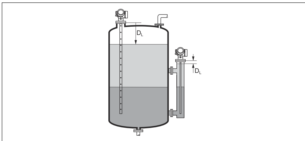
43 界面測定距離
