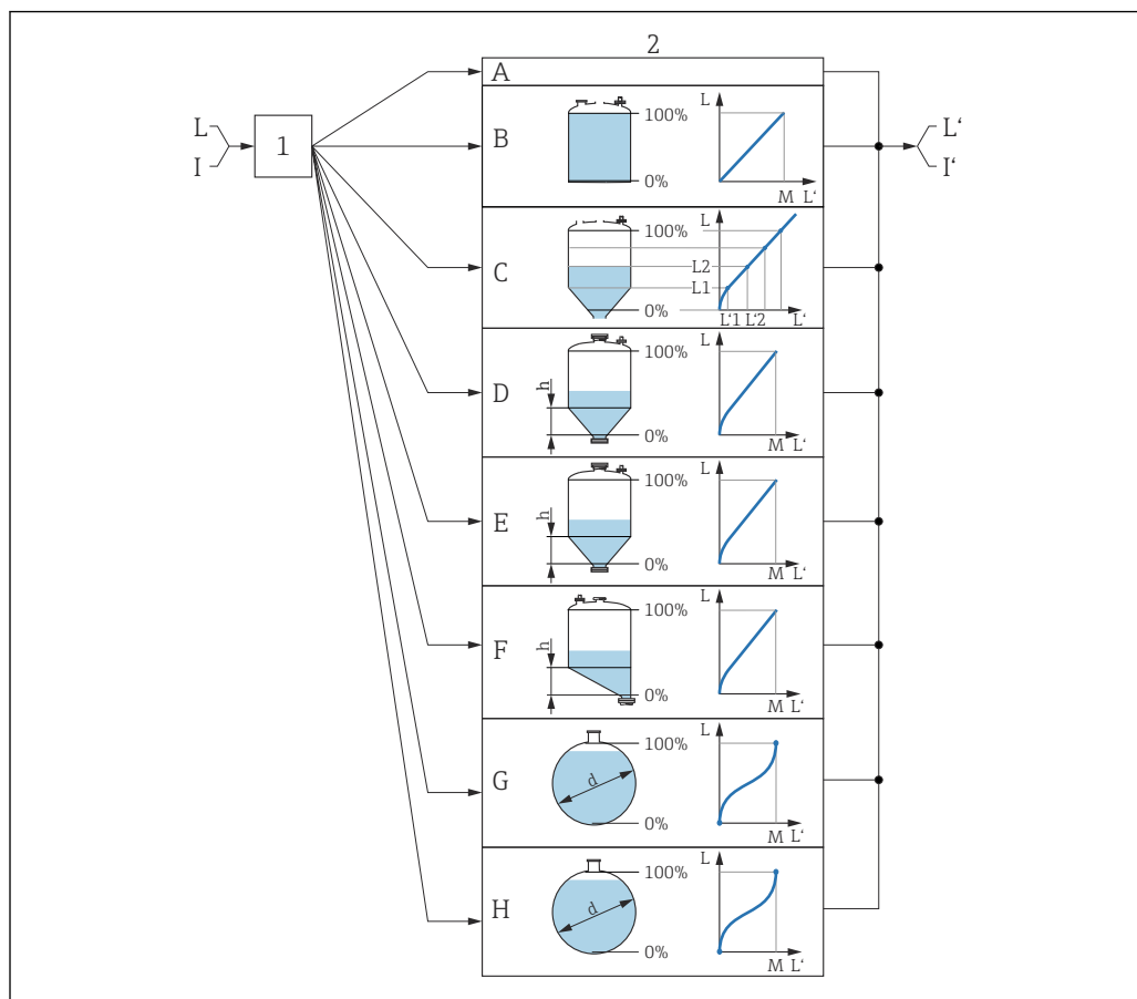
図 45 リニアライゼーション：レベルおよび界面の高さ（該当する場合）を容量または質量に変換します。これは容器の形状に応じて異なります。
