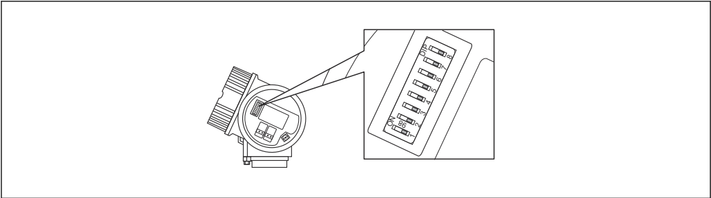
図 24 接続端子室のスイッチのアドレスを指定
