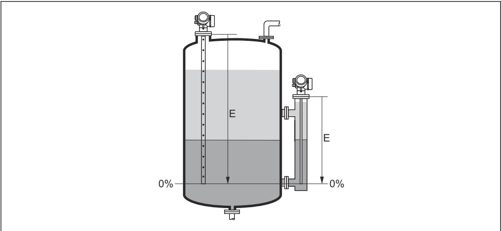
37 界面測定用の空校正 (E)
