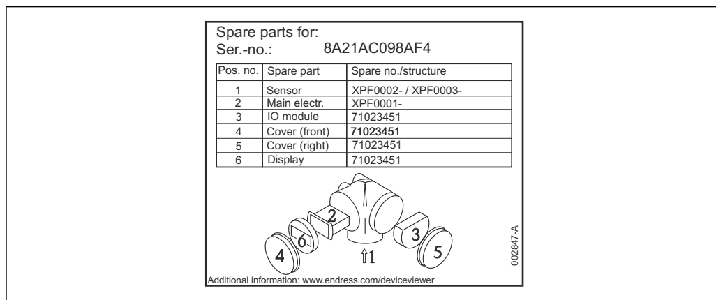
図 32 端子部カバーのスペアパーツ型式銘板の例
