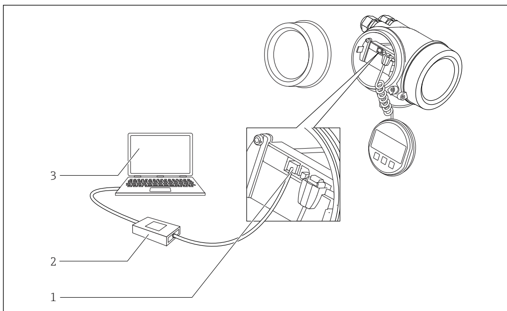
22 サービスインターフェイス（CDI）経由の DeviceCare/FieldCare
