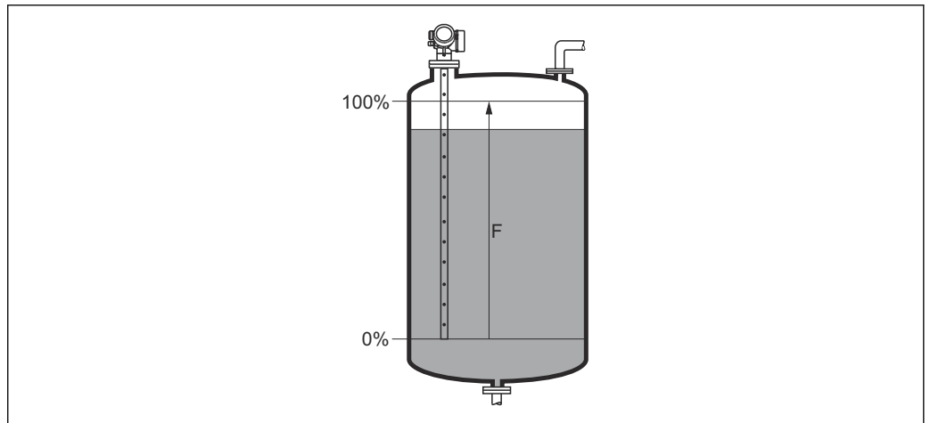
38 液体レベル測定用の満量校正 (F)
