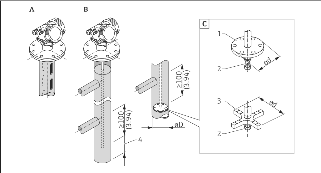
図 6 寸法単位：mm (in)
