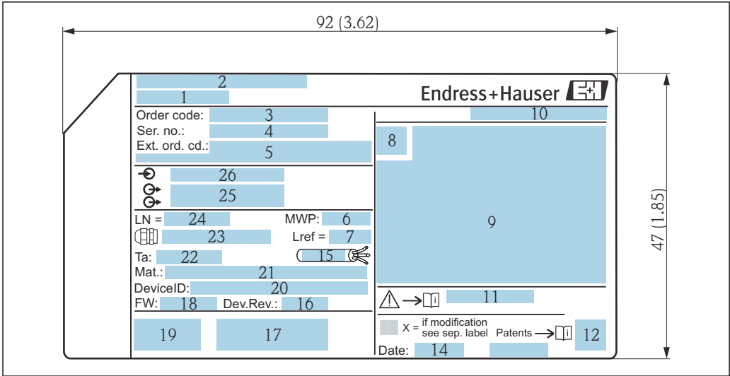
図 3 Levelflex の銘板；寸法単位：mm (in)
