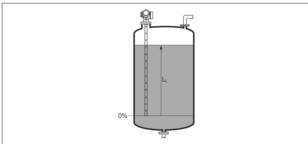
図 40 液体計測時のレベル
