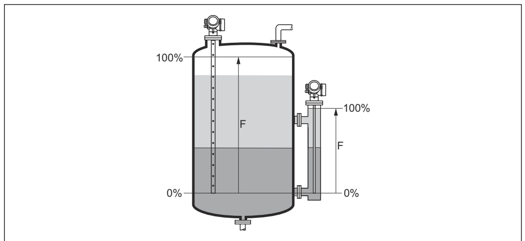
39 界面測定用の満量校正 (F)
