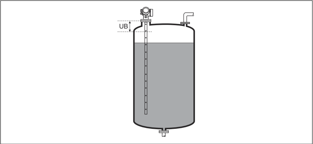
図 44 液体計測の不感知距離 (UB)
