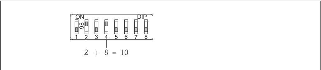
図 25 ハードウェアアドレス指定の例：スイッチ 8 を「オフ」位置にし、スイッチ 1～7 にアドレスを定義します。
