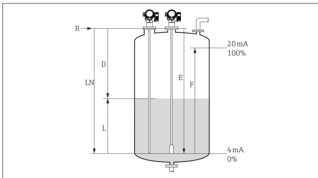
図 28 液体のレベル測定用パラメータの設定
