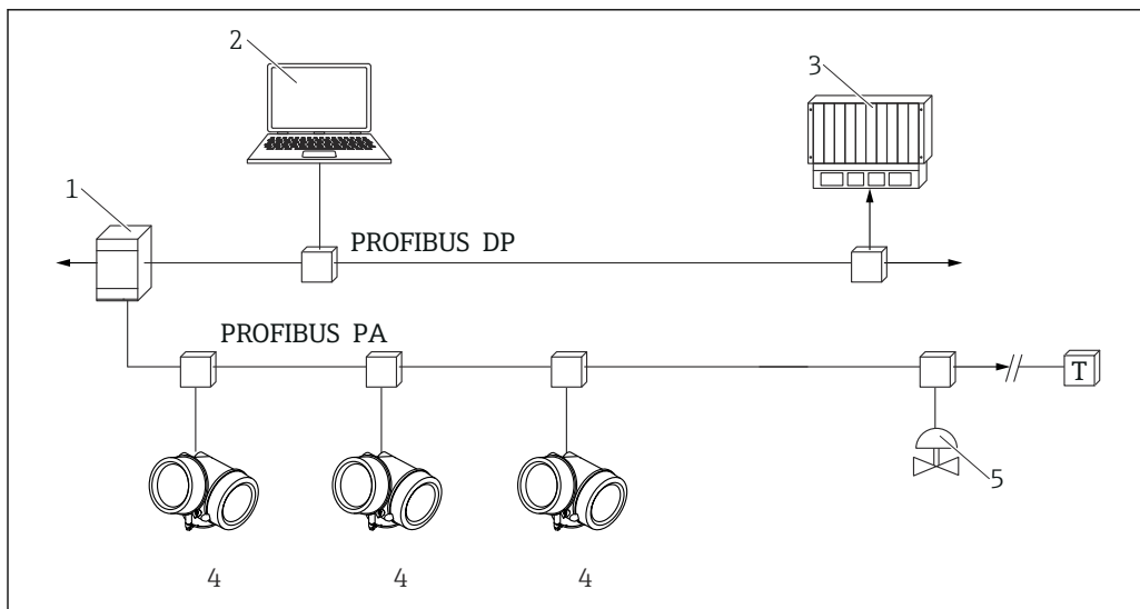
図 21 PROFIBUS PA プロトコルを介したリモート操作のオプション
