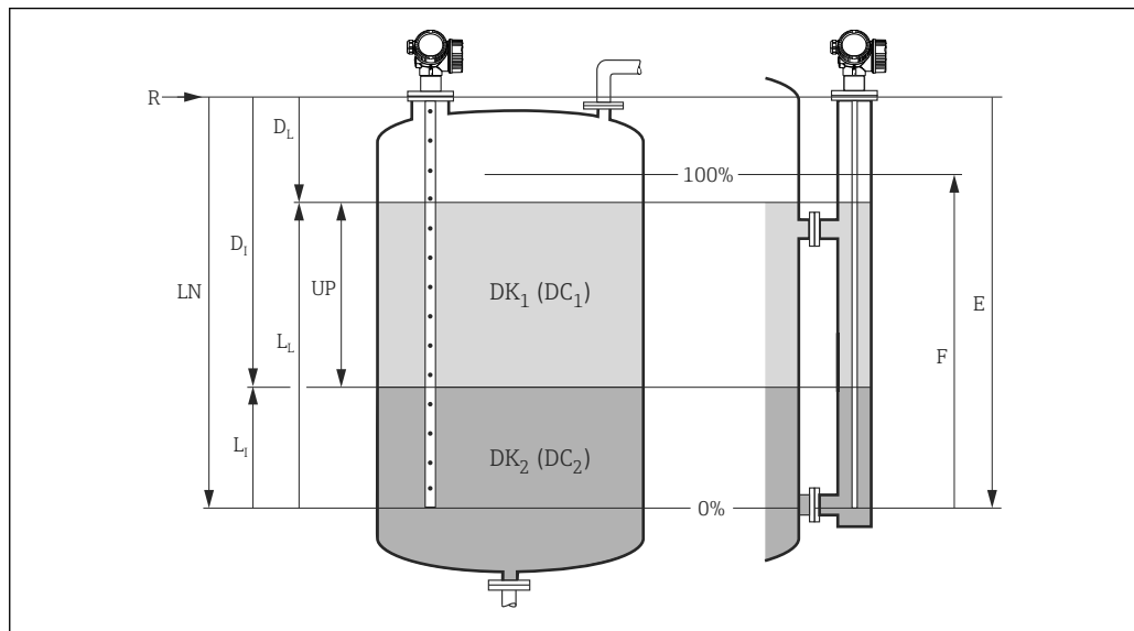
図 29 界面測定用パラメータの設定
