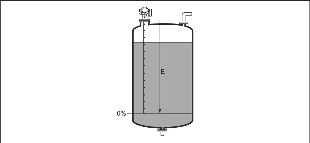
36 液体レベル測定用の空校正 (E)
