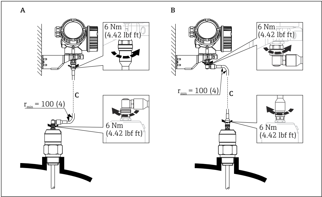
图 7 连接电缆。可选下列方式：
