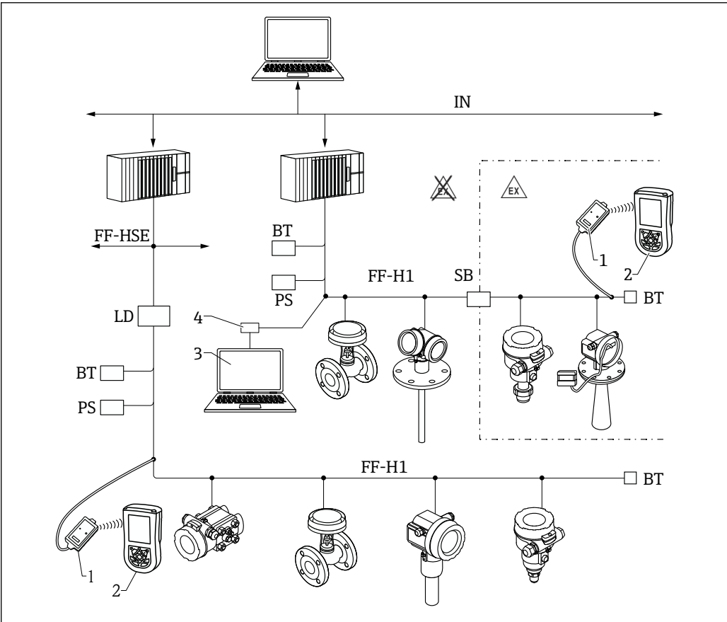
图 16 FOUNDATION Fieldbus 系统架构及其相关部件
