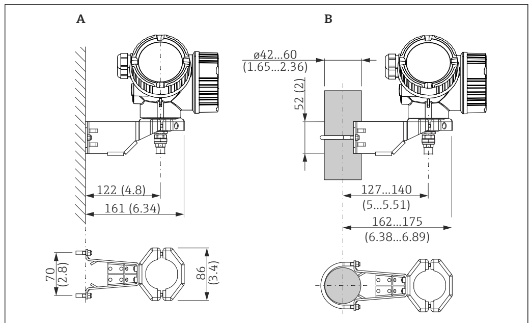
图 6 使用安装支架安装电子腔外壳；单位：mm (in)
