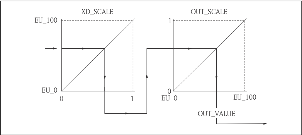
图 24 比例转换 AI 块中的测量值
