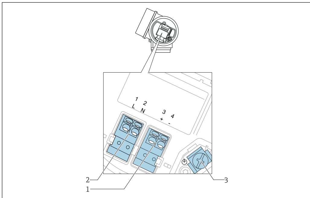
图 8 接线端子分配：四线制；4...20 mA HART (90 ... 253 V AC )
