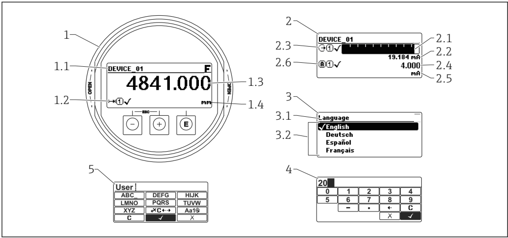
图 18 进行现场操作时显示与操作单元的显示界面
