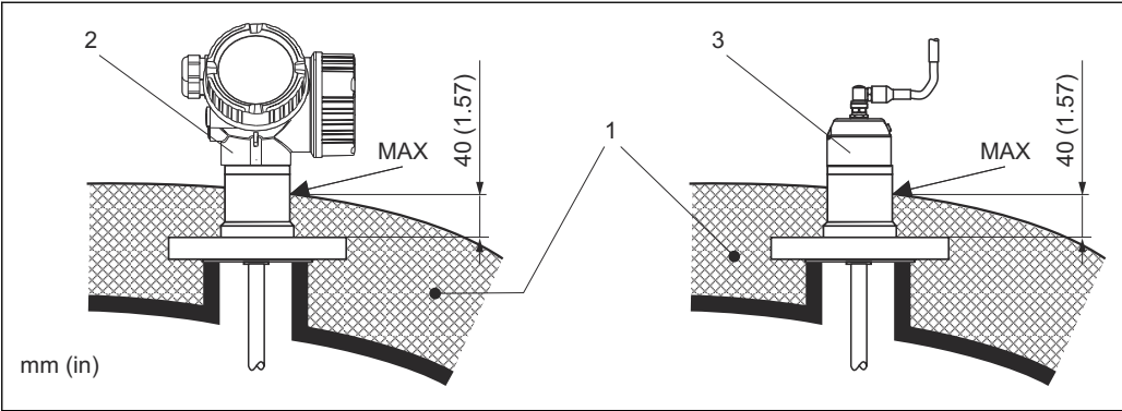
5 带法兰过程连接的 FMP55
