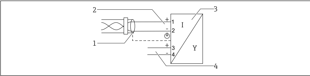
10 接线图: PROFIBUS PA / FOUNDATION Fieldbus
