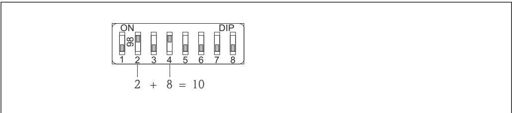
26 Ejemplo de ajuste de dirección mediante hardware: microinterruptor 8 en posición "DESCONECTADO"; los microinterruptores 1 a 7 definen la dirección.
