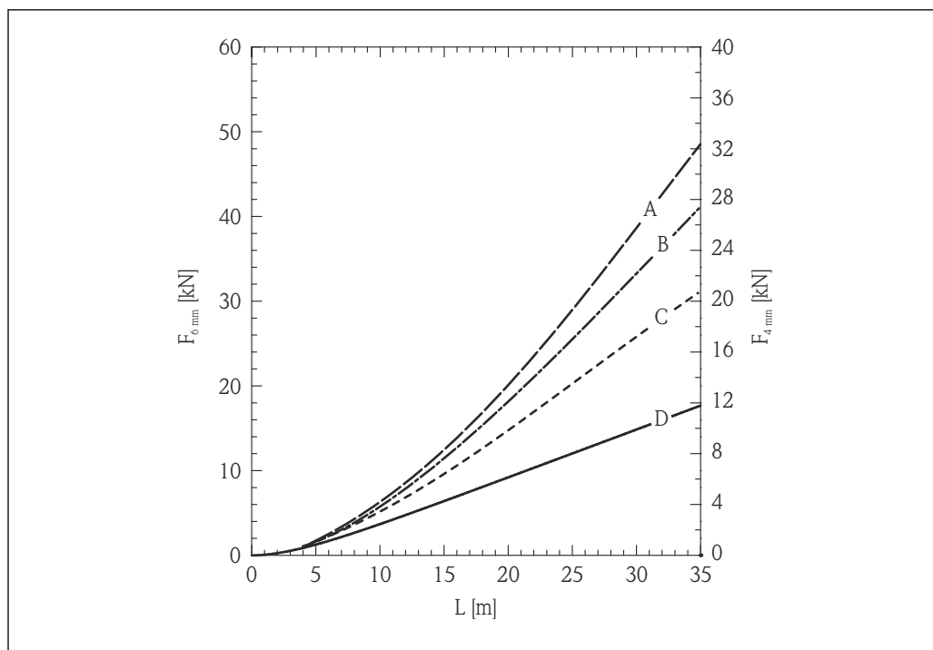
5 Arena de sílice en el silo con paredes metálicas lisas; carga de tracción como función del nivel L para diámetros de cable de 6 mm (0,24 pulgadas) y 4 mm (0,16 pulgadas)
