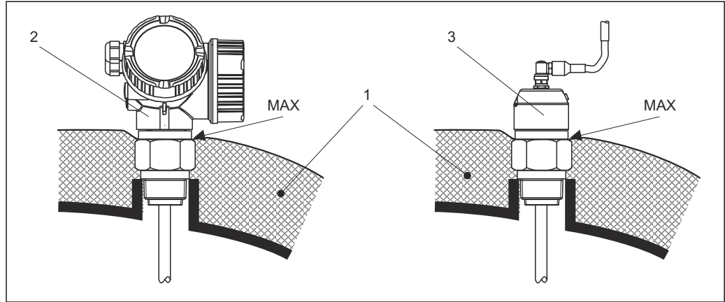
10 Conexión a proceso con rosca - FMP56 y FMP57
