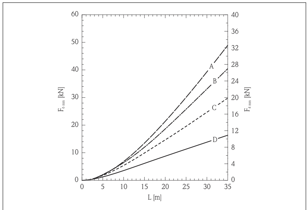
8 Cemento en el silo con paredes metálicas lisas; carga de tracción como función del nivel L para diámetros de cable de 6 mm (0,24 pulgadas) y 4 mm (0,16 pulgadas)
