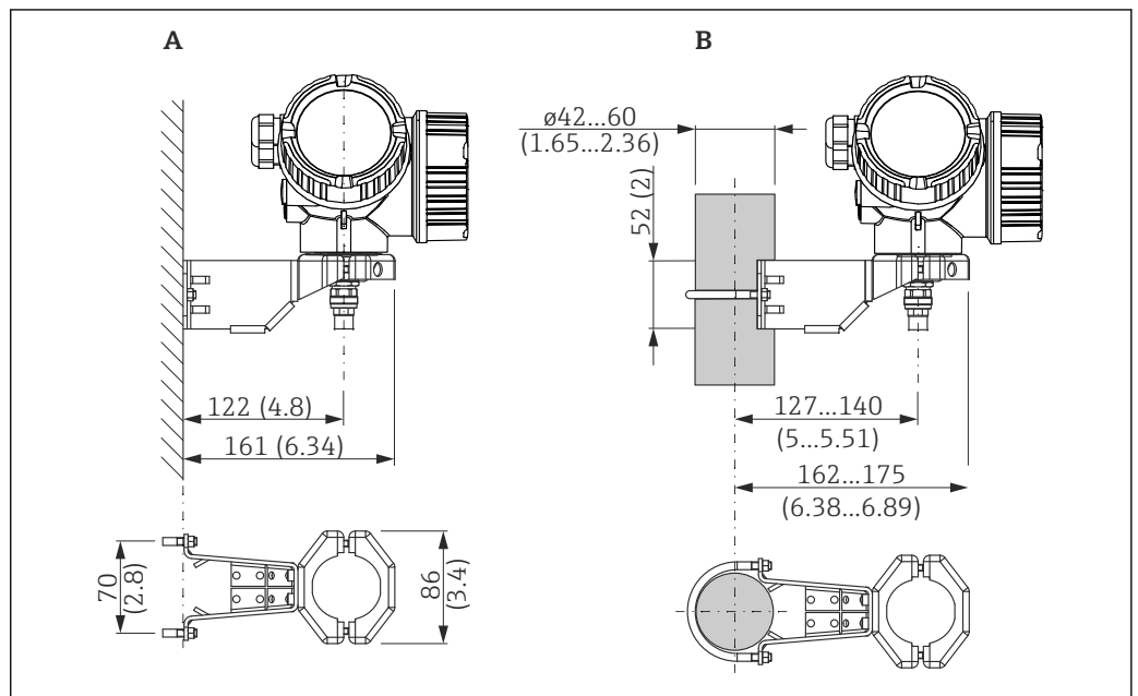
12 Montaje del compartimento de la electrónica con el soporte de montaje; dimensiones: mm (pulgadas)
