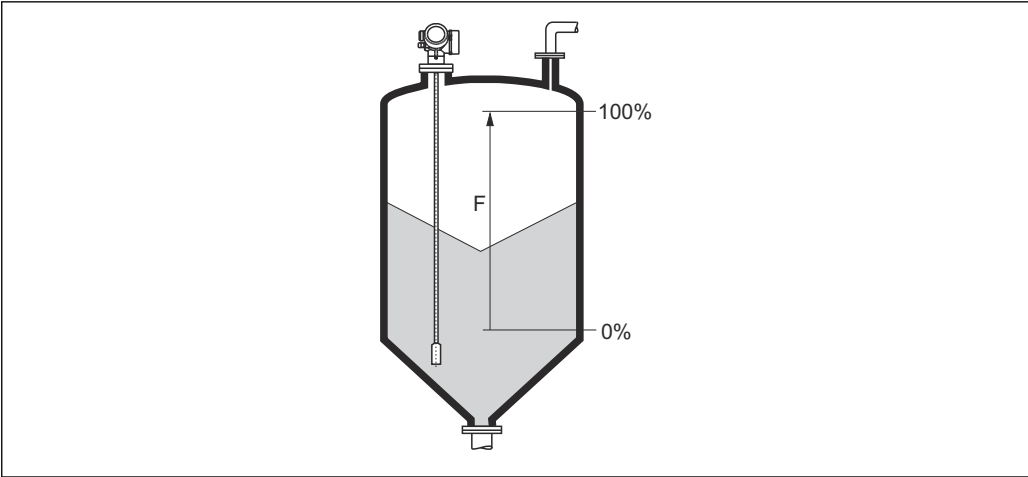
37 Calibración lleno (F) para mediciones de nivel en sólidos granulados
