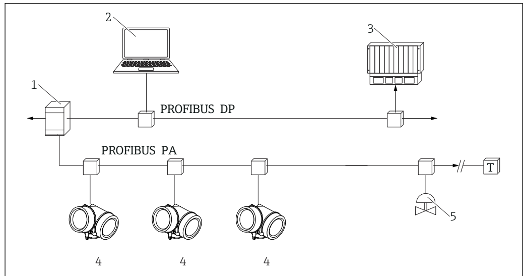
22 Opciones para la configuración a distancia mediante el protocolo de red PROFIBUS PA
