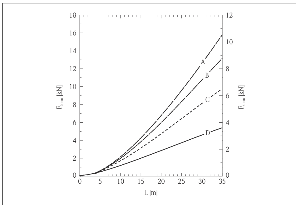
6 Granza de polietileno en el silo con paredes metálicas lisas; carga de tracción como función del nivel L para diámetros de cable de 6 mm (0,24 pulgadas) y 4 mm (0,16 pulgadas)
