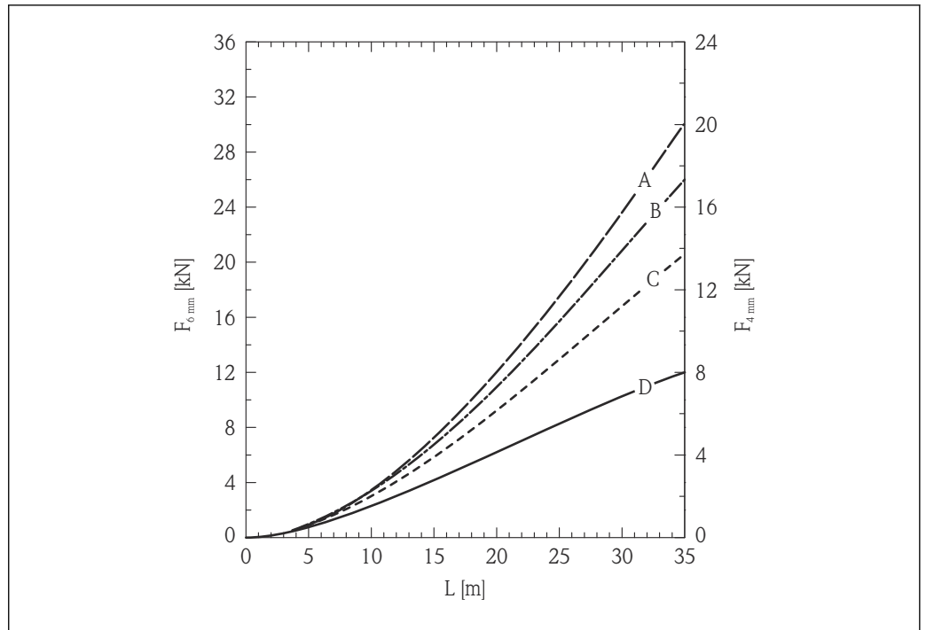
7 Silo de trigo con paredes metálicas lisas; carga de tracción como función del nivel L para diámetros de cable de 6 mm (0,24 pulgadas) y 4 mm (0,16 pulgadas)
