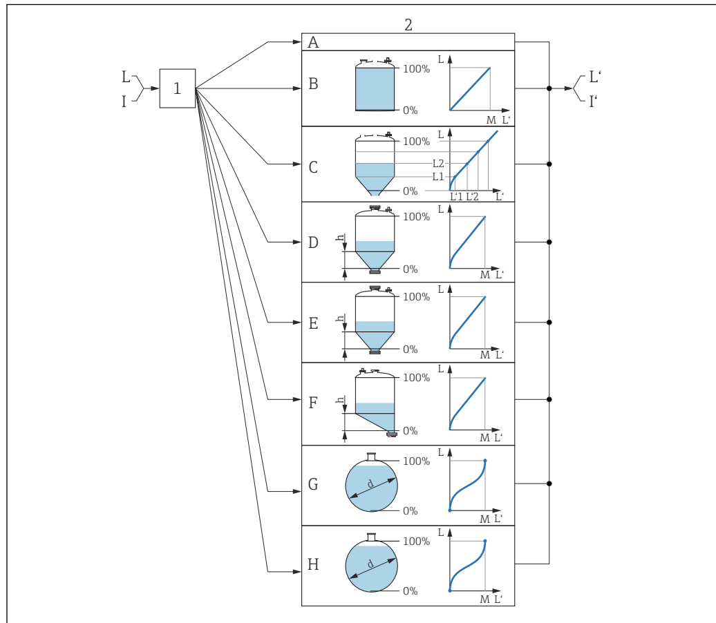
41 Linealización: Transformación del nivel y (si resulta pertinente) de la altura de la interfase en un volumen o peso; la transformación depende de la forma del depósito.
