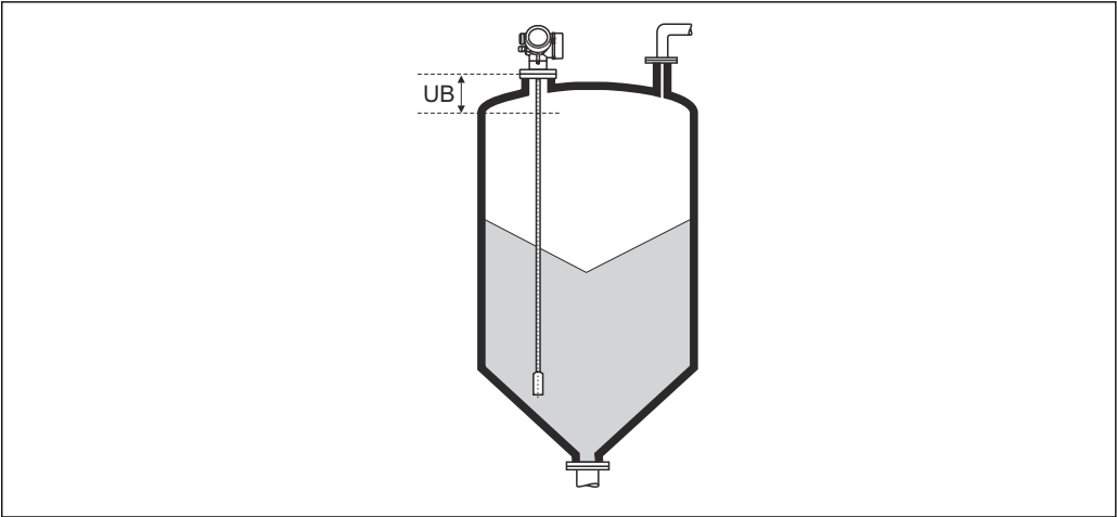
40 Distancia de bloqueo (UB) para mediciones de sólidos granulados
