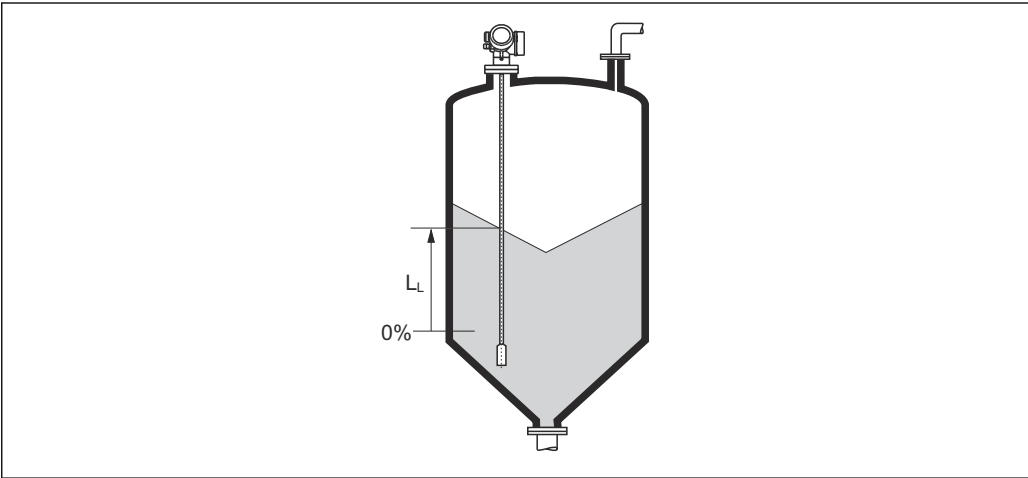
38 Nivel en caso de mediciones de sólidos granulados
