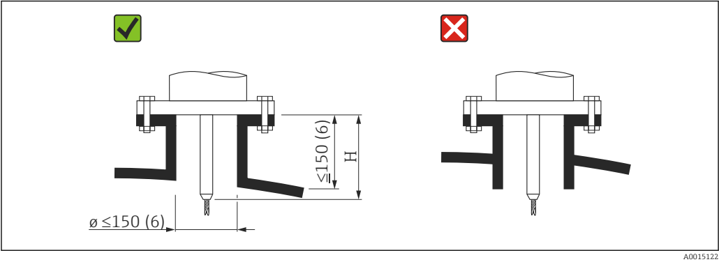
H Longitud de la varilla central o de la parte rígida de la sonda de cable
