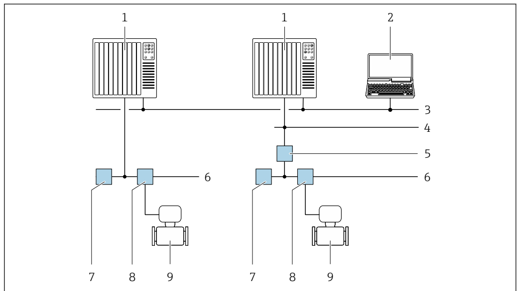
54 Possibilités de configuration à distance via réseau FOUNDATION Fieldbus
