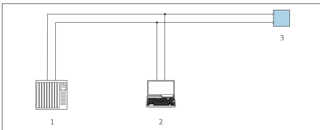
57 Options de configuration à distance via protocole Modbus-RS485 (active)
