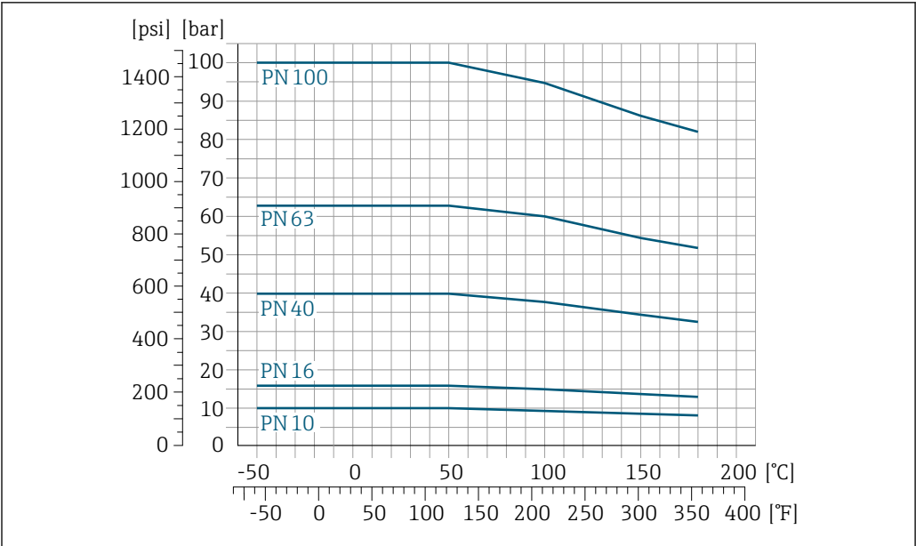
31 Avec matériau de bride 1.4404 (316/316L)
