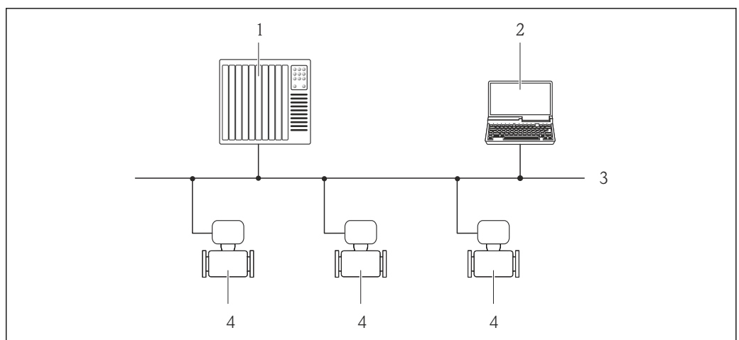
55 Possibilités de configuration à distance via réseau PROFIBUS DP
