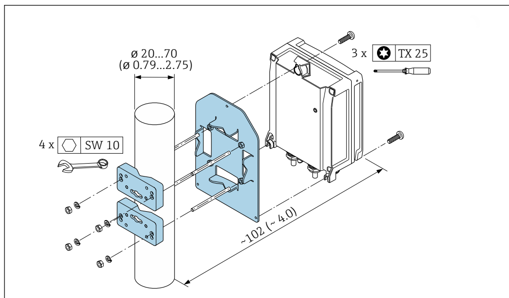
24 Unité de mesure mm (in)
