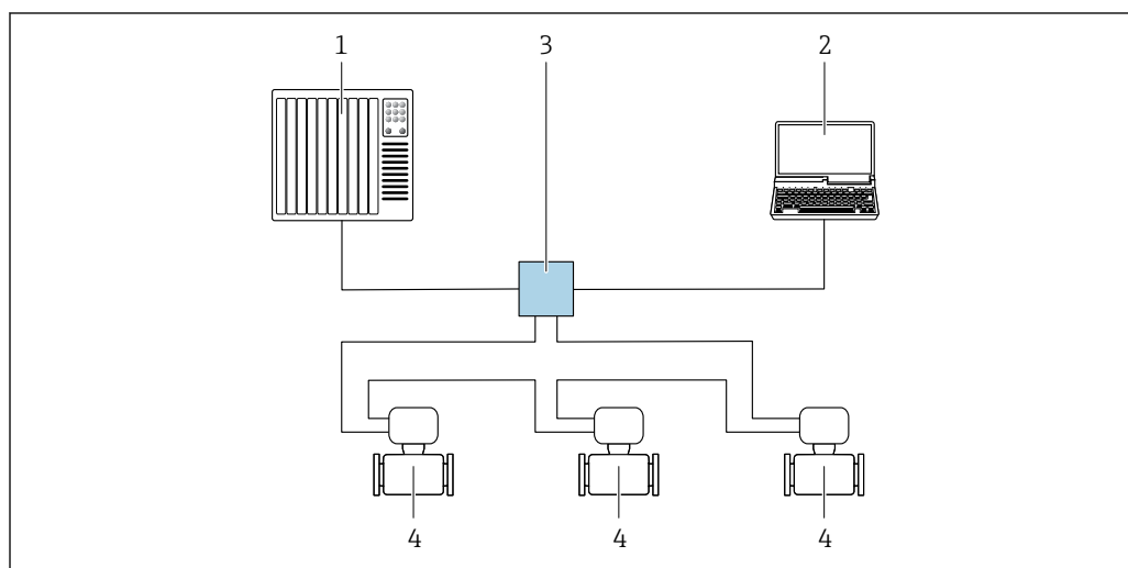
61 Options de configuration à distance via réseau PROFINET : topologie en anneau
