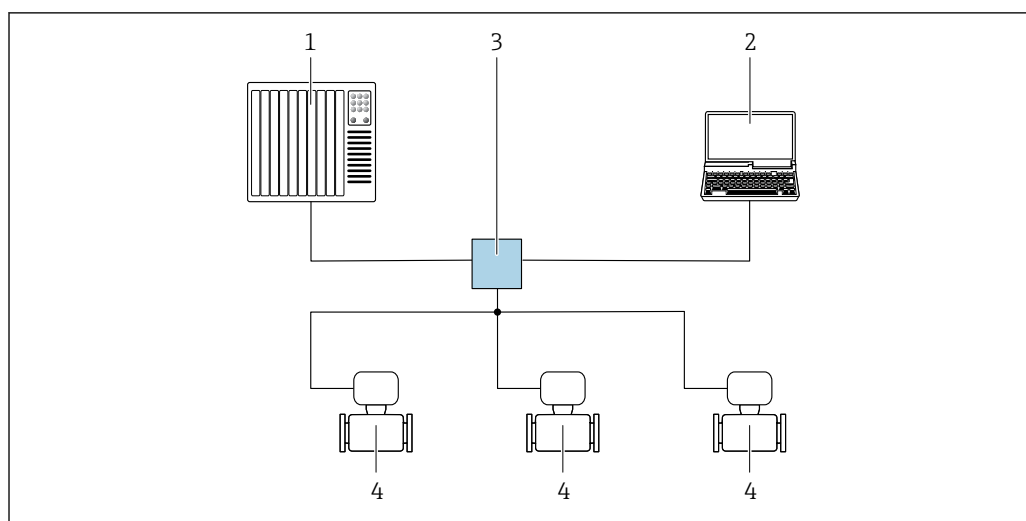
60 Options de configuration à distance via réseau PROFINET : topologie en étoile
