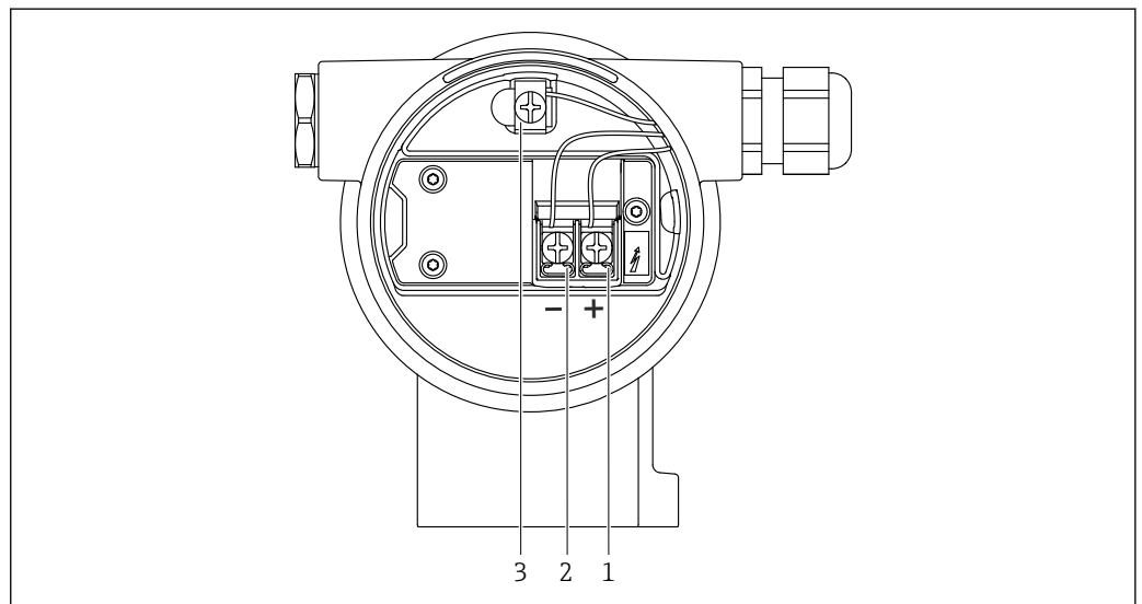
图 4 接线腔内的接线端子和接地端子
