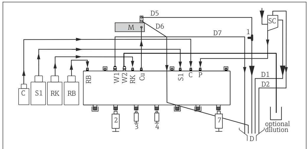
64 Liquiline System CA80CR, Einkanalgerät
