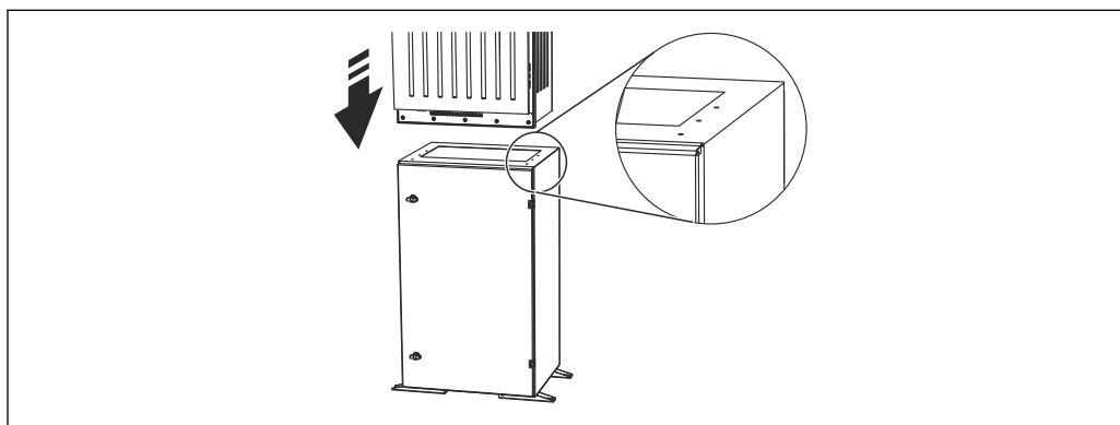
21 Befestigung Sockel
