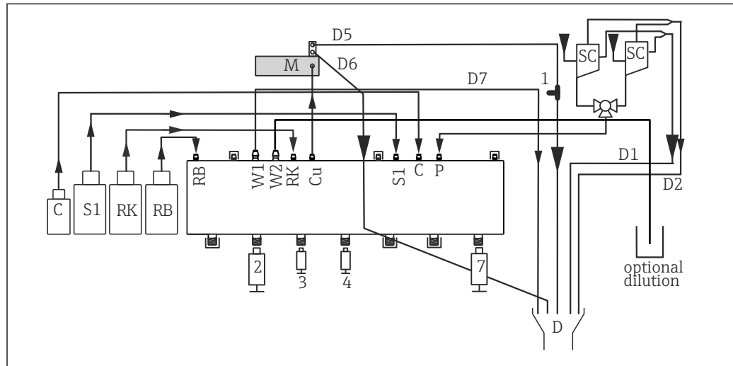
65 Liquiline System CA80CR, Zweikanalgerät
