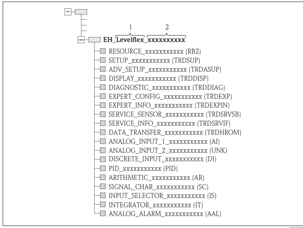
25 Visualización común en un programa de configuración tras establecer la conexión
