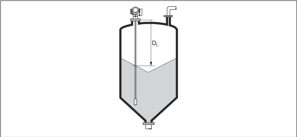
42 Distancia para mediciones de sólidos granulados
