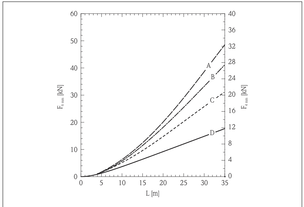
5 Arena de sílice en el silo con paredes metálicas lisas; carga de tracción como función del nivel L para diámetros de cable de 6 mm (0,24 pulgadas) y 4 mm (0,16 pulgadas)
