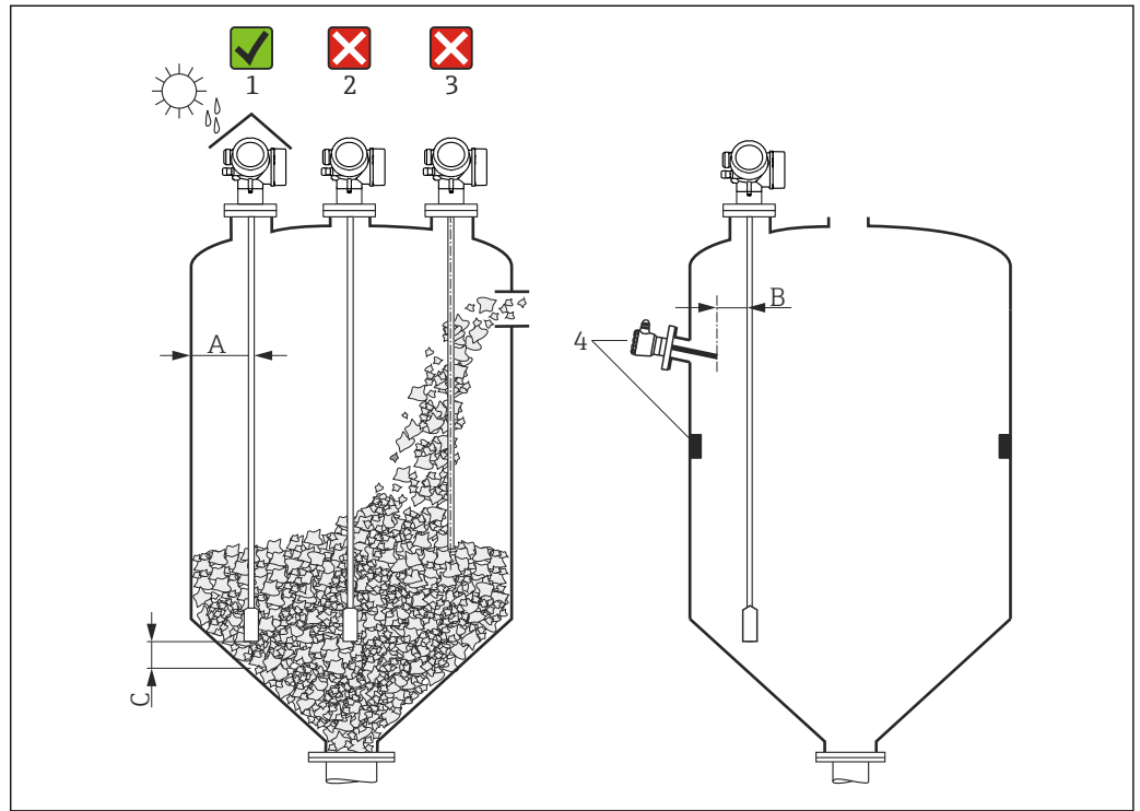
4 Requisitos para el montaje de Levelflex
