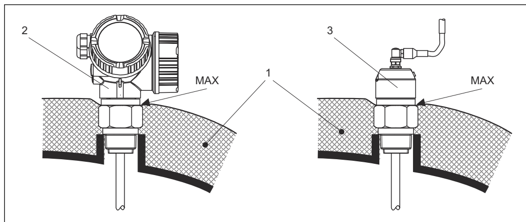
10 Conexión a proceso con rosca - FMP56 y FMP57
