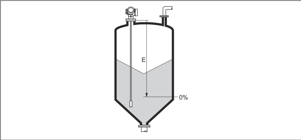
39 Calibración vacío (E) para mediciones de nivel en sólidos granulados.
