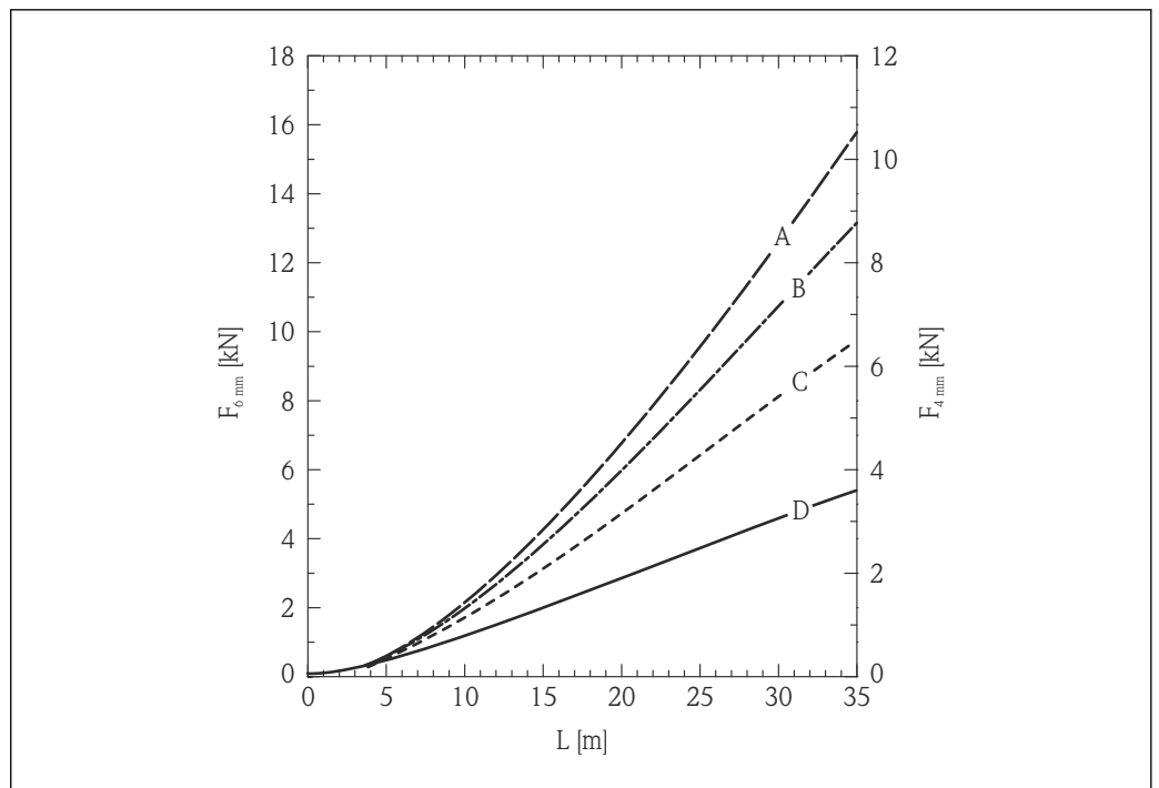
6 Granza de polietileno en el silo con paredes metálicas lisas; carga de tracción como función del nivel L para diámetros de cable de 6 mm (0,24 pulgadas) y 4 mm (0,16 pulgadas)
