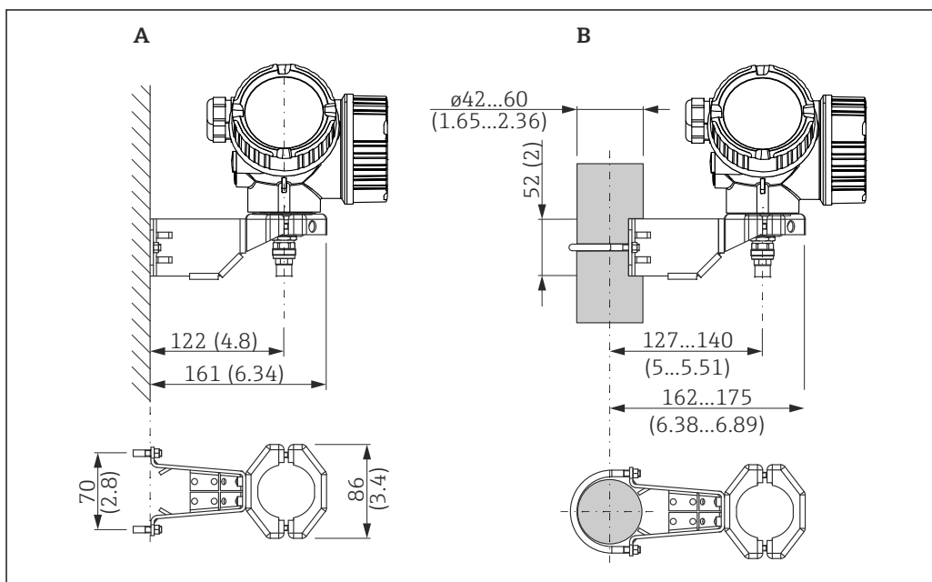
12 Montaje del compartimento de la electrónica con el soporte de montaje; dimensiones: mm (pulgadas)
