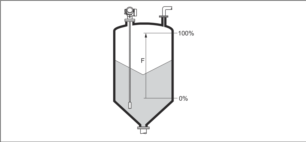
40 Calibración lleno (F) para mediciones de nivel en sólidos granulados
