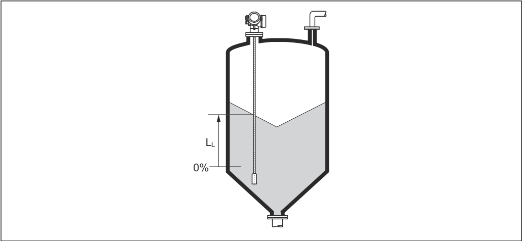
41 Nivel en caso de mediciones de sólidos granulados
