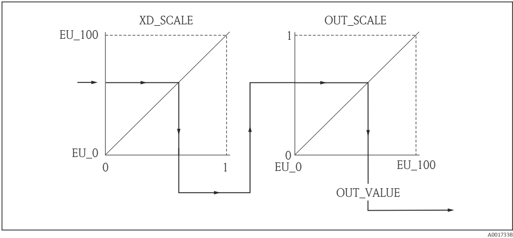
30 Escalado del valor medido en un bloque AI
