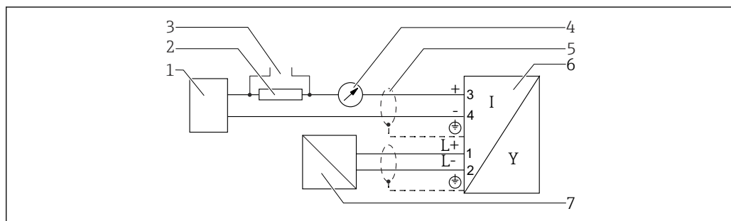
13 Schéma de principe 4 fils : 4-20 mA HART (10,4 ... 48 V DC )
