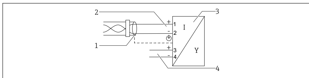
17 Блок-схема: PROFIBUS PA/FOUNDATION Fieldbus
