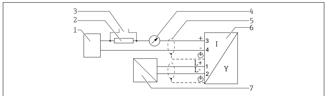
13 Блок-схема 4-проводного подключения: 4–20 мА HART (10,4 до 48 В DC )
