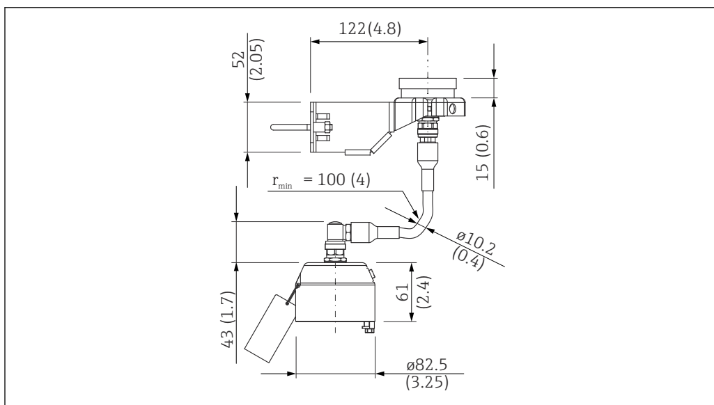
37 Соединительный элемент для дистанционного зонда. Длина соединительного кабеля: согласно заказу. Единица измерения мм (дюйм)
