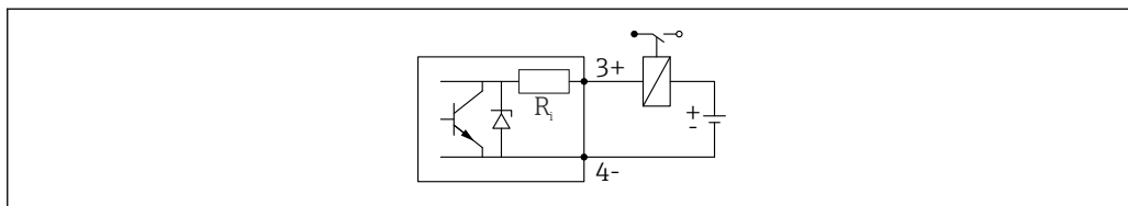
18 Подключение реле
