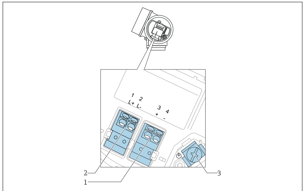
12 Назначение клемм, 4-проводное подключение; 4–20 мА HART (10,4 до 48 В DC )
