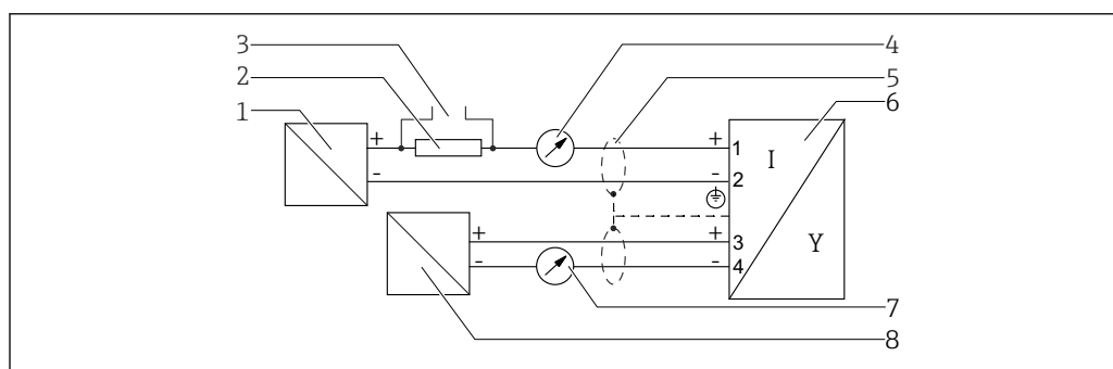
11 Блок-схема 2-проводного подключения: 4–20 мА HART, 4–20 мА
