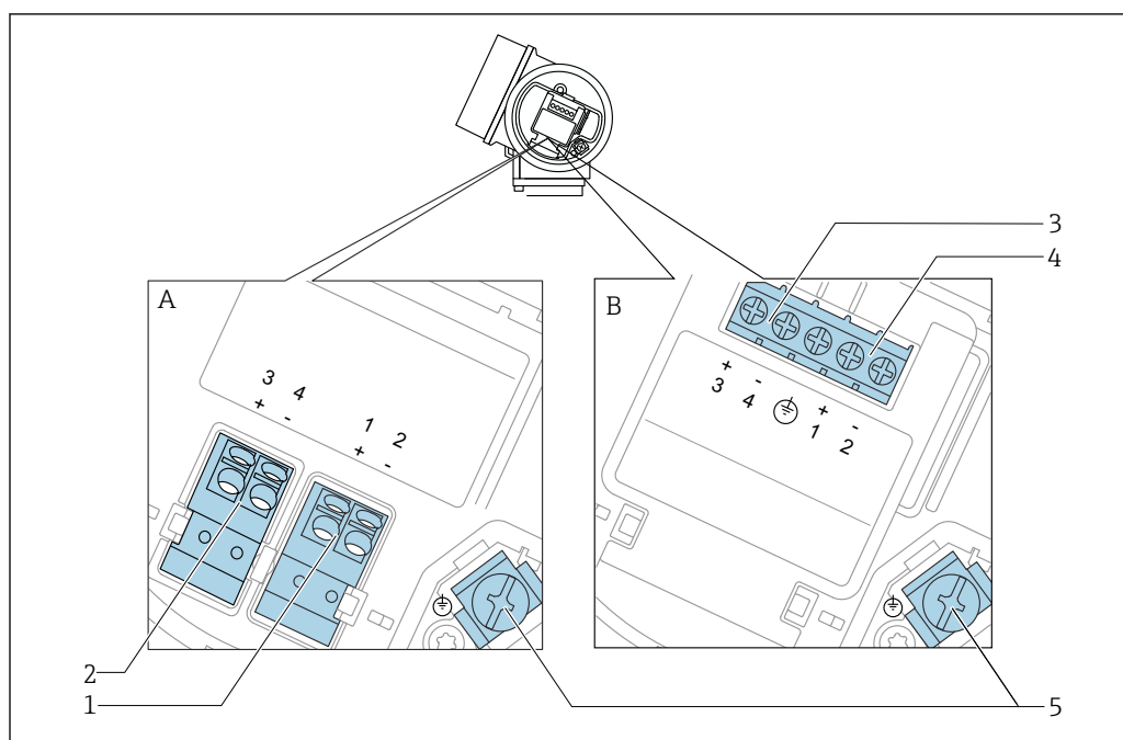
10 Назначение клемм; 2-проводное подключение; 4–20 мА HART, 4–20 мА
