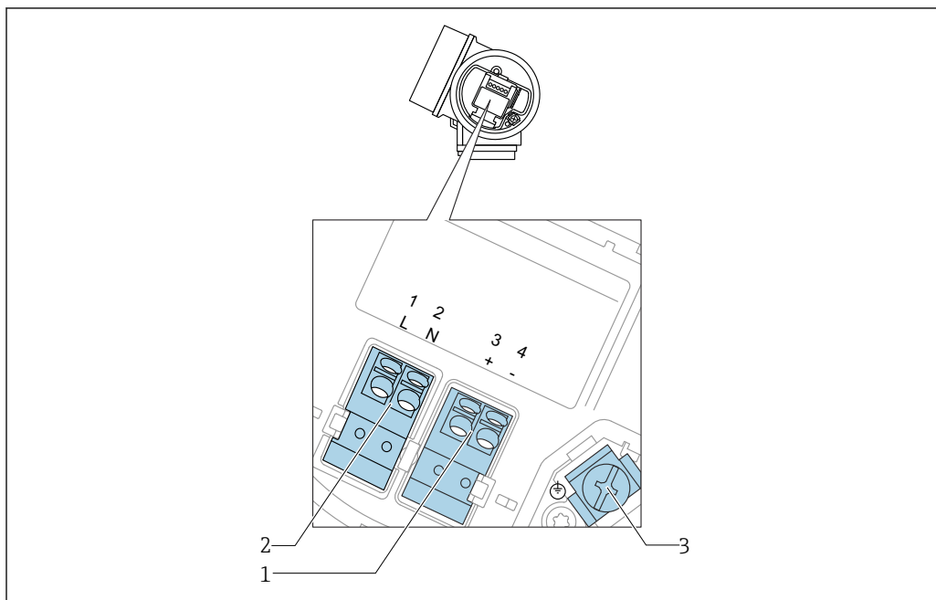
14 Назначение клемм, 4-проводное подключение; 4–20 мА HART (90 до 253 V AC )
