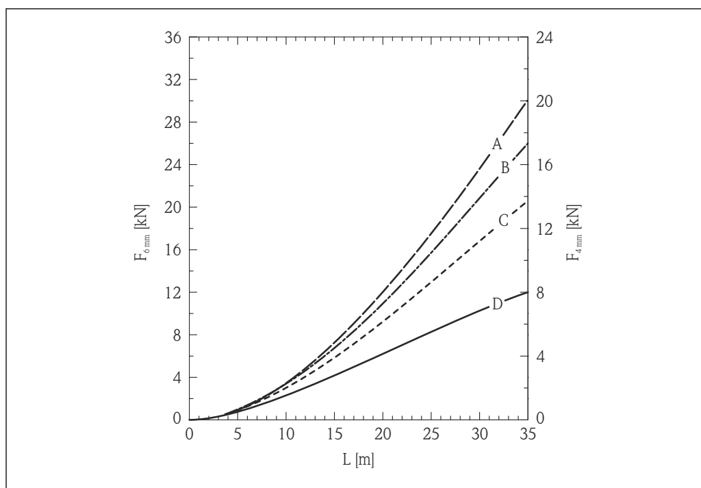
28 Пшеница в металлическом бункере с гладкими стенками; зависимость растягивающей нагрузки от уровня L для диаметров троса 6 мм (0,24 дюйм) и 4 мм (0,16 дюйм)
