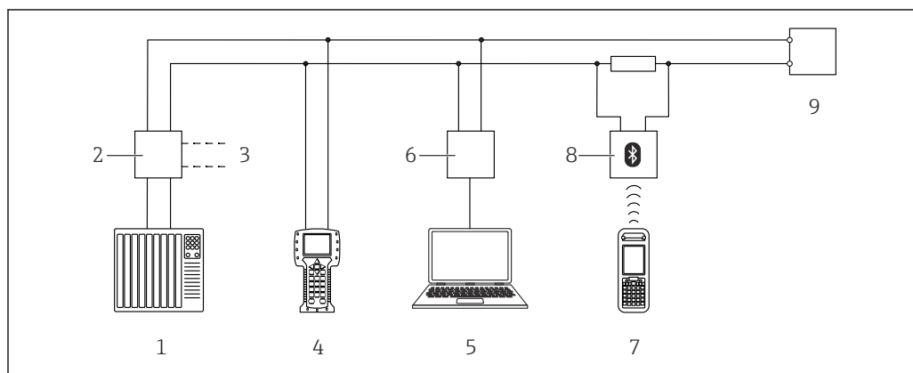
43 Варианты дистанционного управления по протоколу HART
