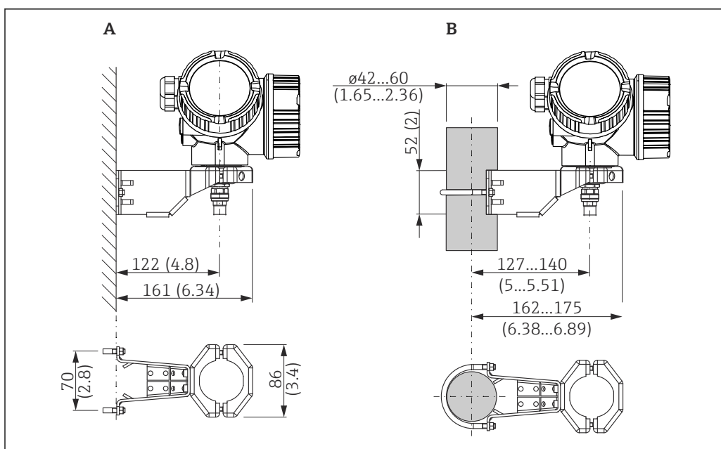
36 Монтажный кронштейн для корпуса электроники. Единица измерения мм (дюйм)
