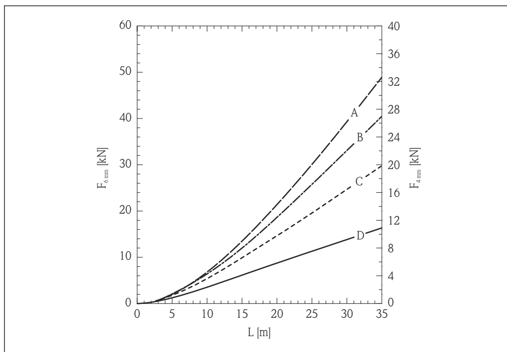
29 Цемент в металлическом бункере с гладкими стенками; зависимость растягивающей нагрузки от уровня L для диаметров троса 6 мм (0,24 дюйм) и 4 мм (0,16 дюйм)
