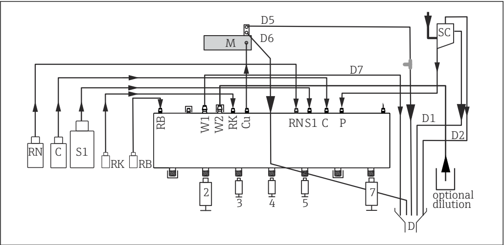
64 Liquiline System CA80AL, dispositivo a un canale
