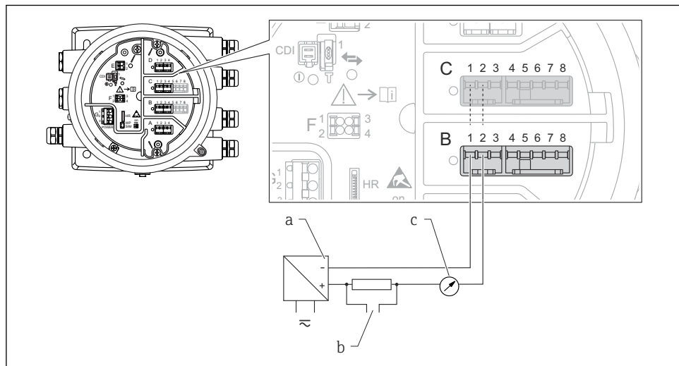
12 Uso pasivo del módulo de E/S analógica en el modo de salida
