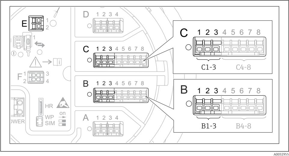
29 Terminales posibles para circuitos HART
