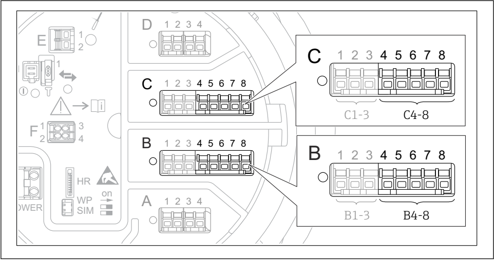
32 Ubicaciones posibles de los módulos E/S analógicos, a los que se puede conectar una RTD. Los módulos que están realmente presentes dependen del código de producto del equipo.
