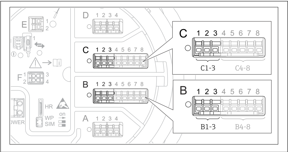
35 Ubicaciones posibles de los módulos E/S analógicos, que pueden utilizarse como salida 4-20 mA. Los módulos que están realmente presentes dependen del código de producto del equipo.
