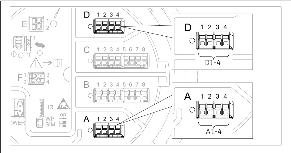
36 Ubicaciones posibles de los módulos Modbus (ejemplos); en función de la versión del equipo, estos módulos también pueden ocupar las ranuras B o C → 34.
