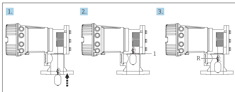
27 Secuencia de calibración de referencia
