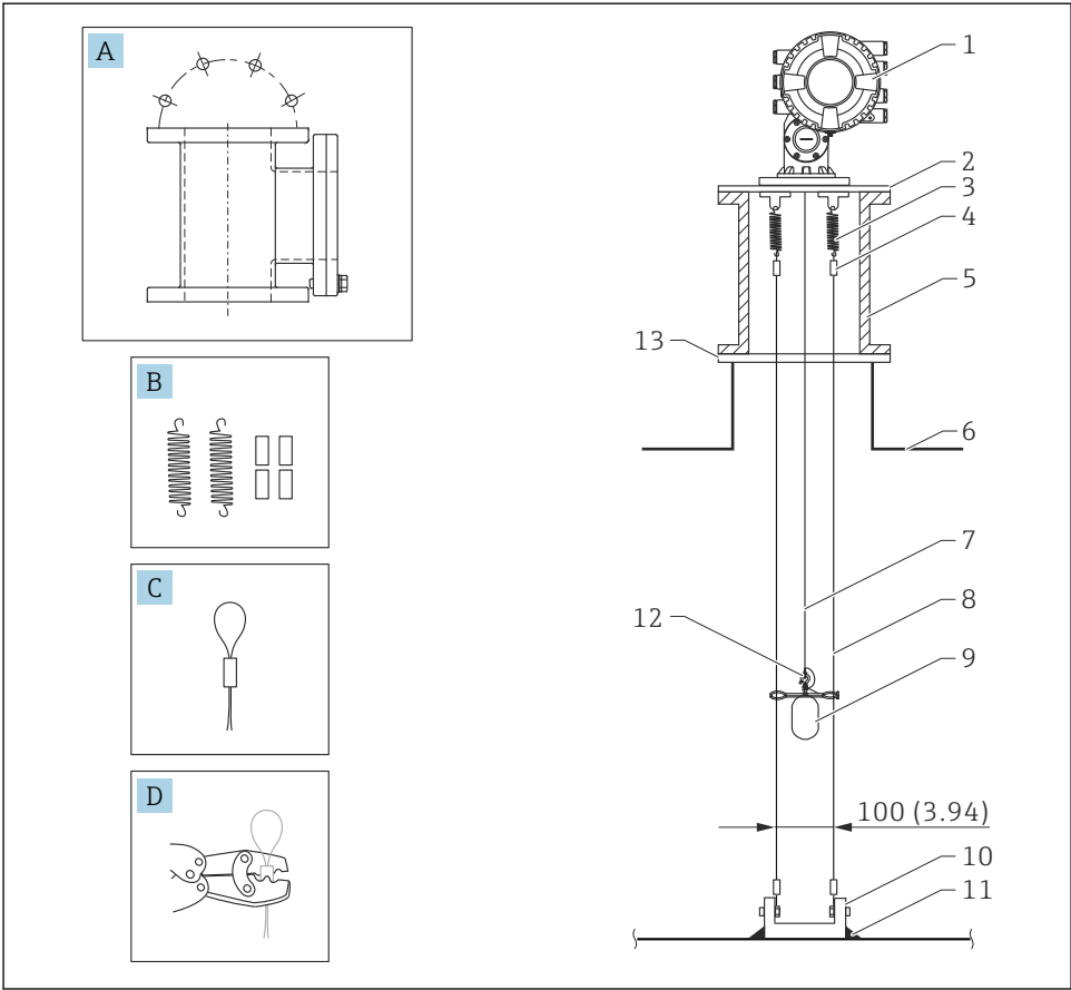
3 Cable guía; dimensiones en mm (in)
