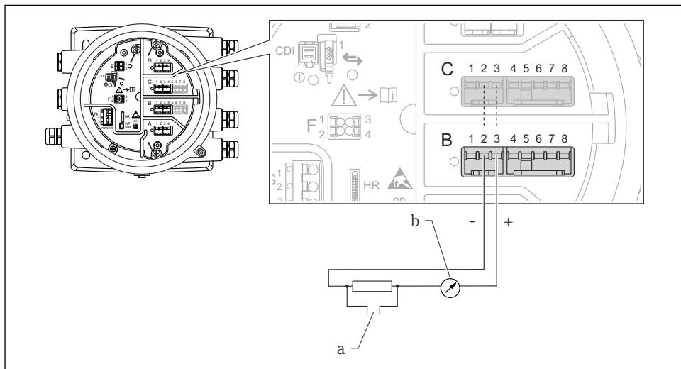
15 Uso activo del módulo de E/S analógica en el modo de salida
