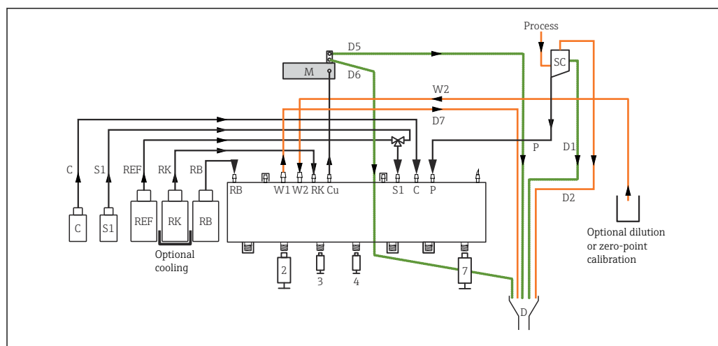
64 Liquiline System CA80AM, dispositivo a un canale
