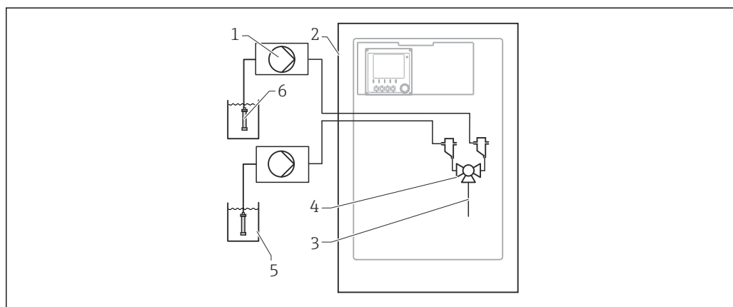
7 Ensemble de mesure avec 2x Liquiline System CAT820
