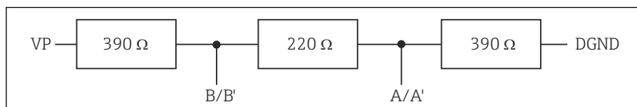
54 Structure de la terminaison interne
