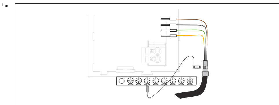
35 Morsettiera
