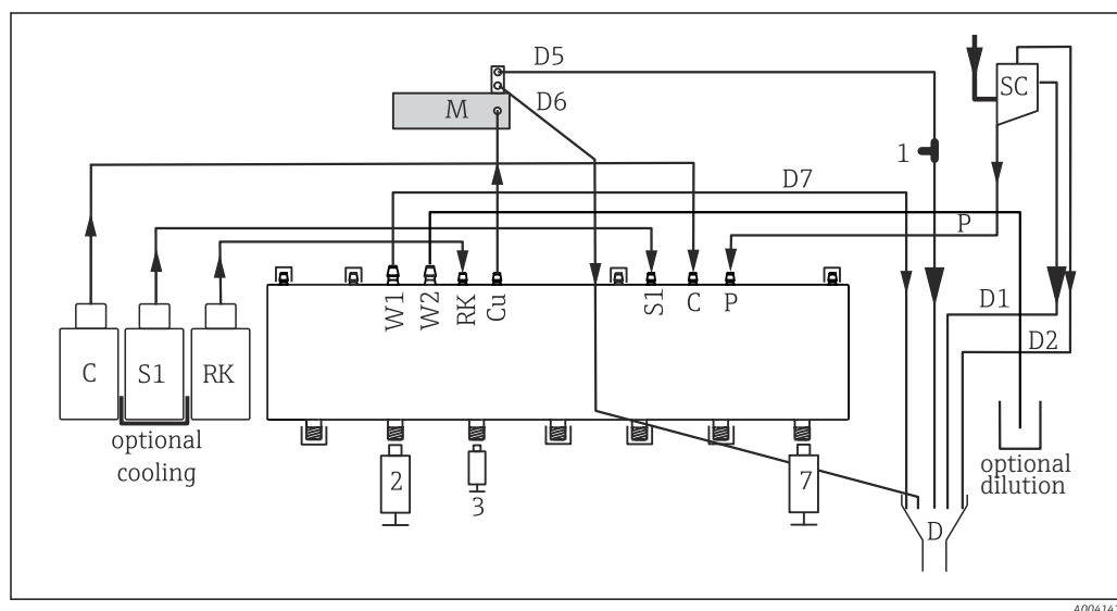
64 Liquiline System CA80NO, dispositivo a un canale
