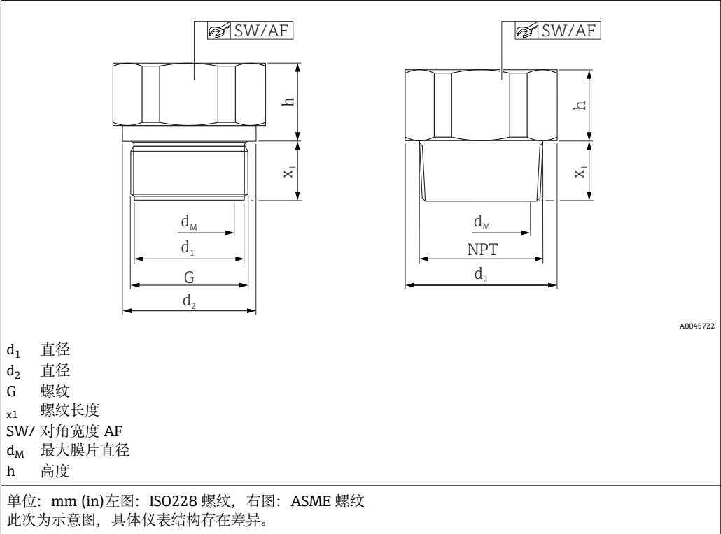
ISO228 螺纹、ASME 螺纹、齐平膜片、隔膜密封系统、TempC 膜片
