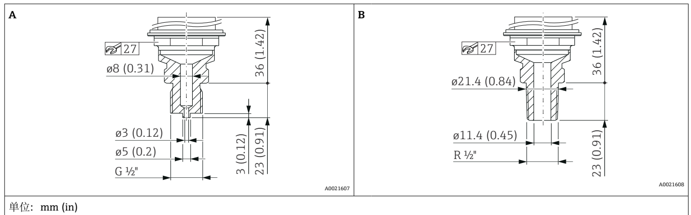
JIS 螺纹过程连接, 内置膜片 (不带隔膜密封系统的标准型仪表)
