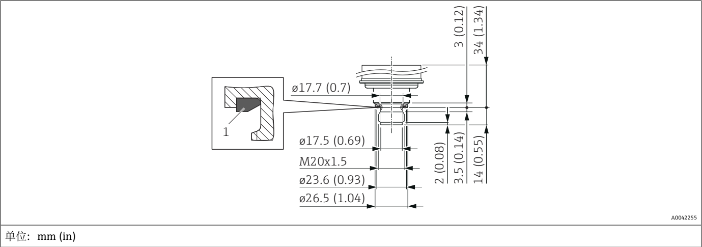
DIN 螺纹过程连接，齐平安装膜片（不带隔膜密封系统的标准型仪表）
