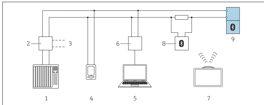
図 8 HART 経由のリモート操作用オプション
