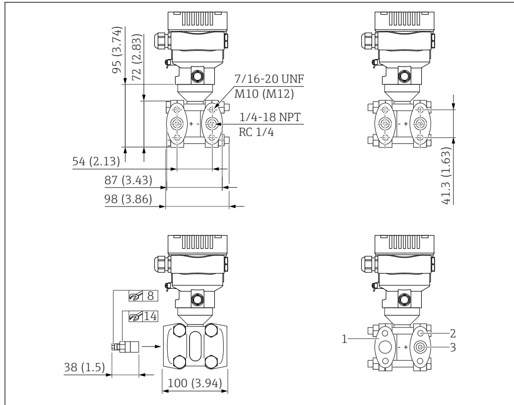
图 6 正视图、左视图、右视图。测量单位 mm (in)
