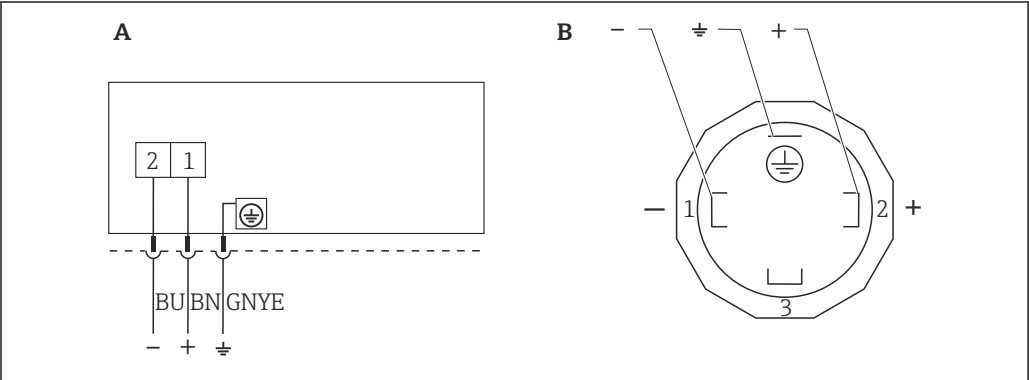
2 BN = 棕色, BU = 蓝色, GNYE = 绿/黄相间 A 带霍斯曼插头的仪表的电气连接 B 仪表上的连接插头
