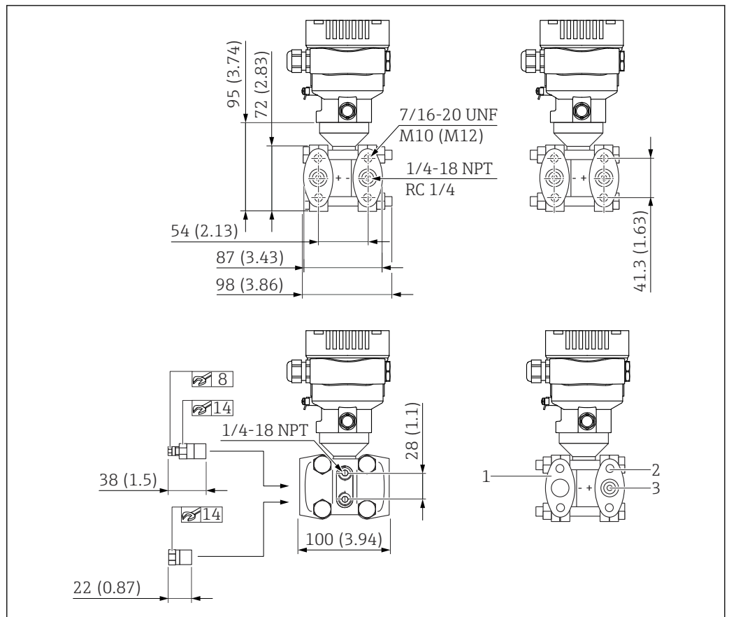
图 7 正视图、左视图、右视图。螺母始终安装在负压侧。测量单位 mm (in)
