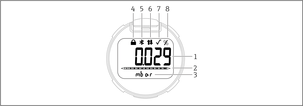
图 8 段码显示屏
