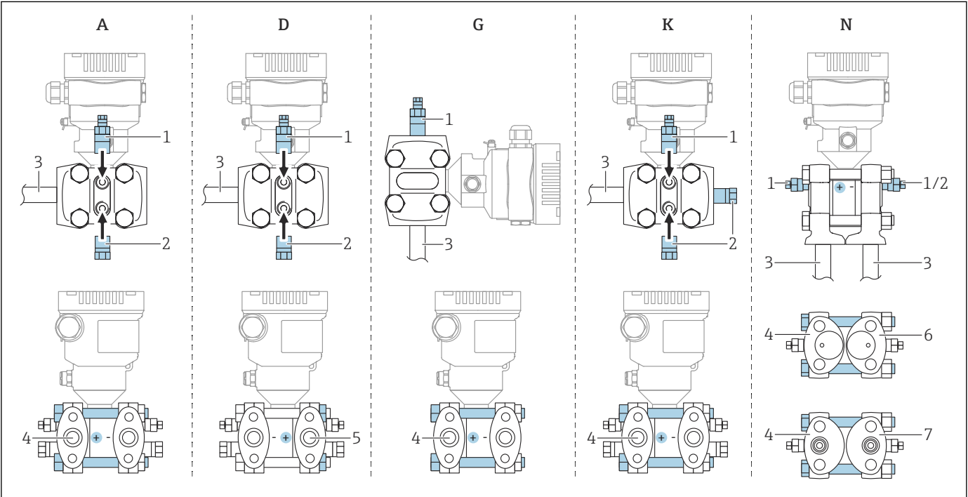
图 4 选型代号: A、D、G、K、N
