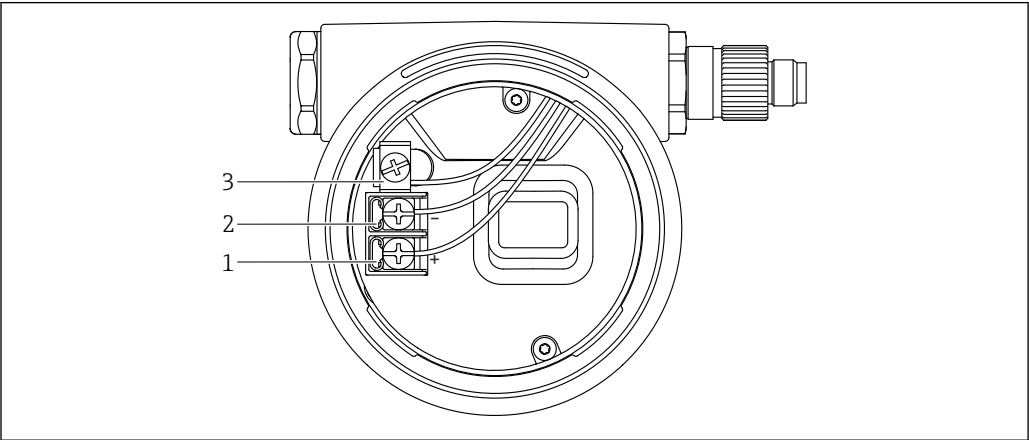
1 接线腔内的接线端子和接地端子 1 “+”接线端 2 “-”接线端 3 内部接地端
