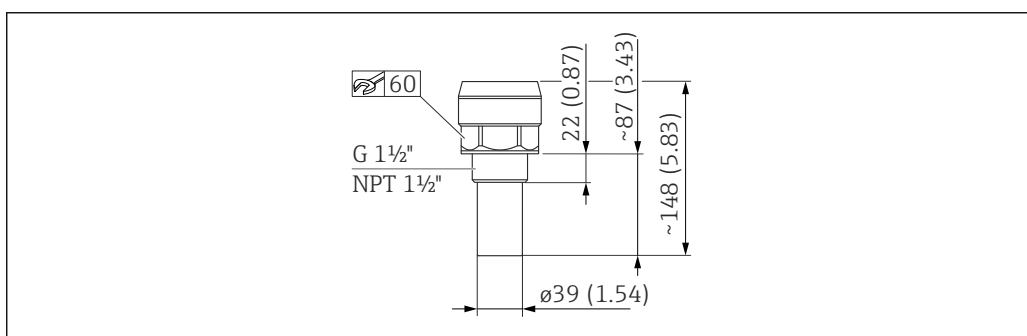
図 19 FMU40 センサの寸法。測定単位 mm (in)
