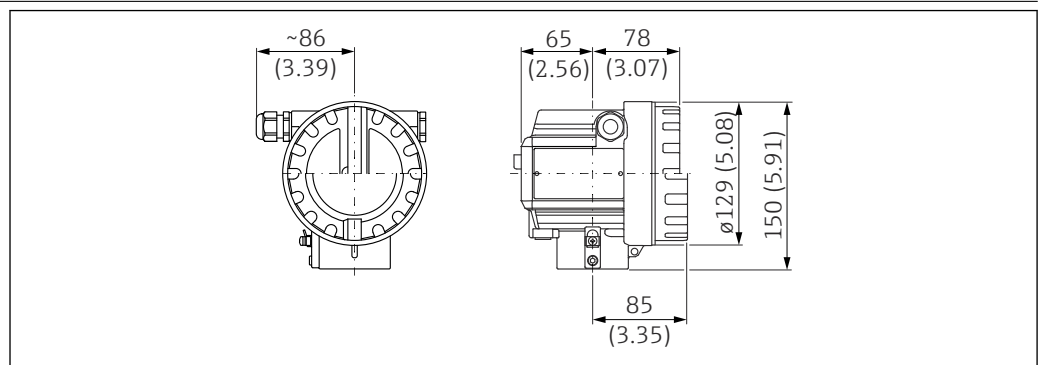
図 17 F12 ハウジングの寸法。測定単位 mm (in)
