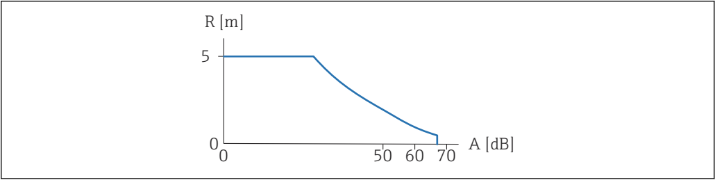
4 Diagramme de la gamme
