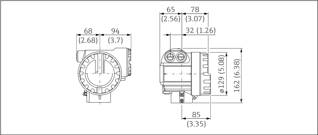
18 Dimensions du boîtier T12. Unité de mesure mm (in)
