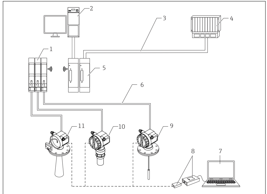
22 Intégration système via Rackbus Endress+Hauser
