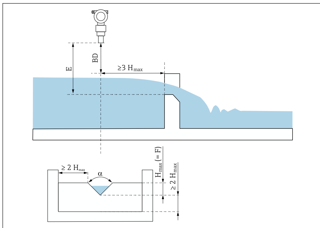
11 Déversoir triangulaire (exemple)
