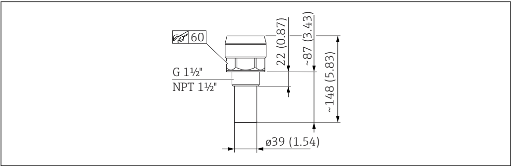
19 Dimensions du capteur FMU40. Unité de mesure mm (in)
