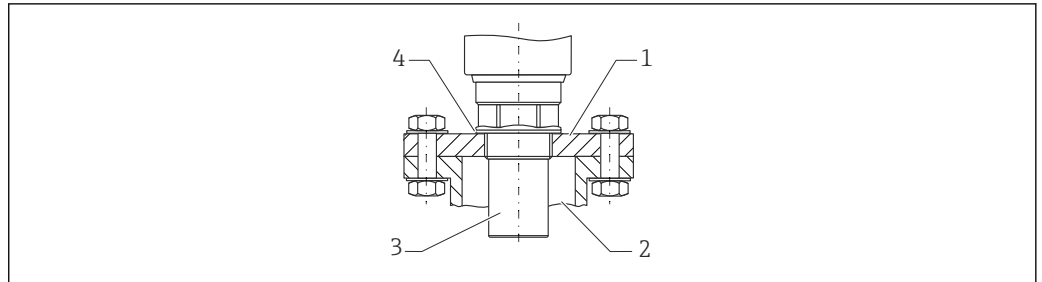
28 Bride à visser FAX50
