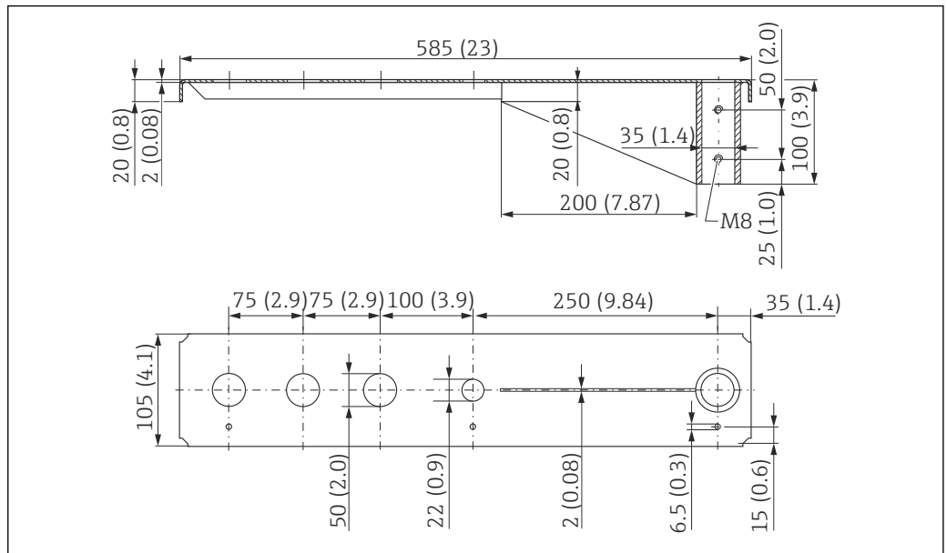
32 Dimensions. Unité de mesure mm (in)
