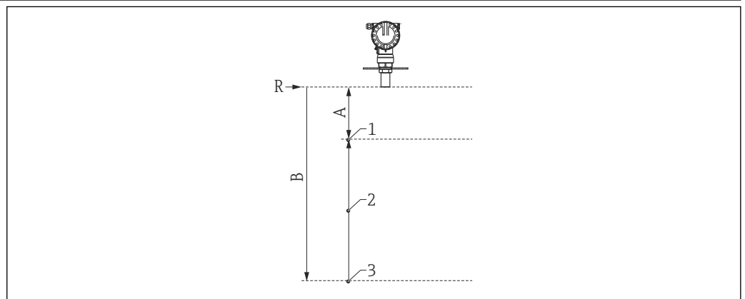
25 Exemple de protocole de linéarité en 3 points
