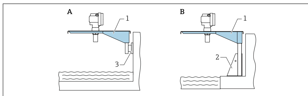
34 Bras de montage avec support de montage ou support mural
