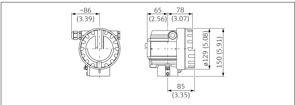
17 Dimensions du boîtier F12. Unité de mesure mm (in)
