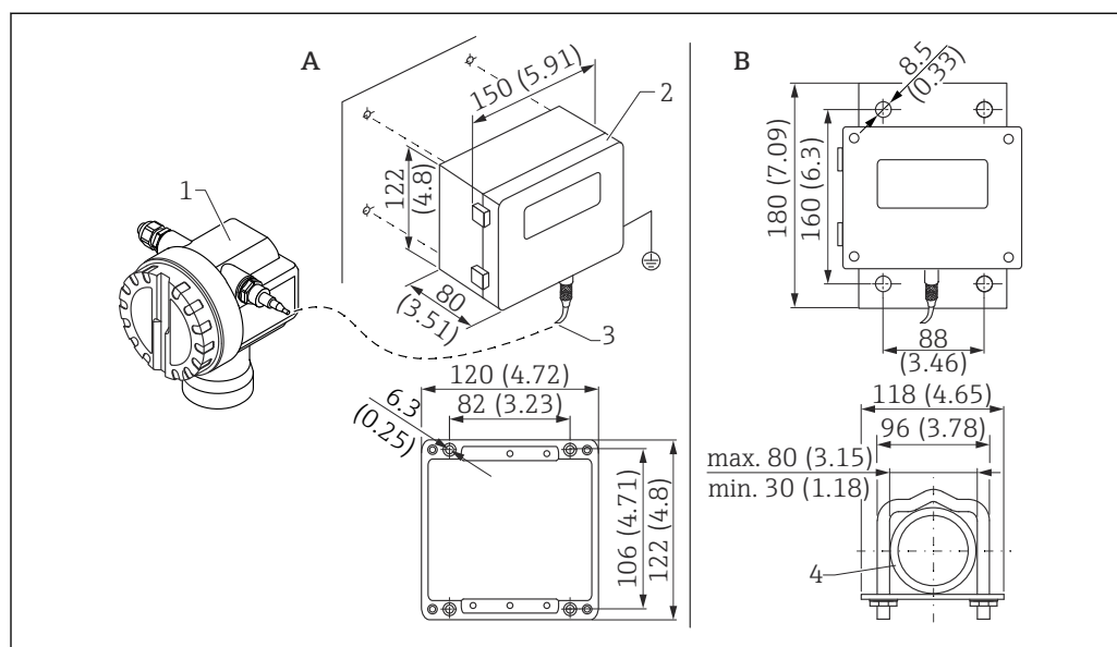
35 Afficheur séparé. Unité de mesure mm (in)
