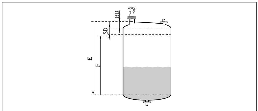
15 Paramètres pour le fonctionnement correct de l'appareil
