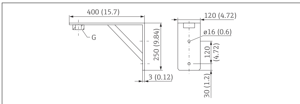
27 Dimensions de l'étrier de montage. Unité de mesure mm (in)
