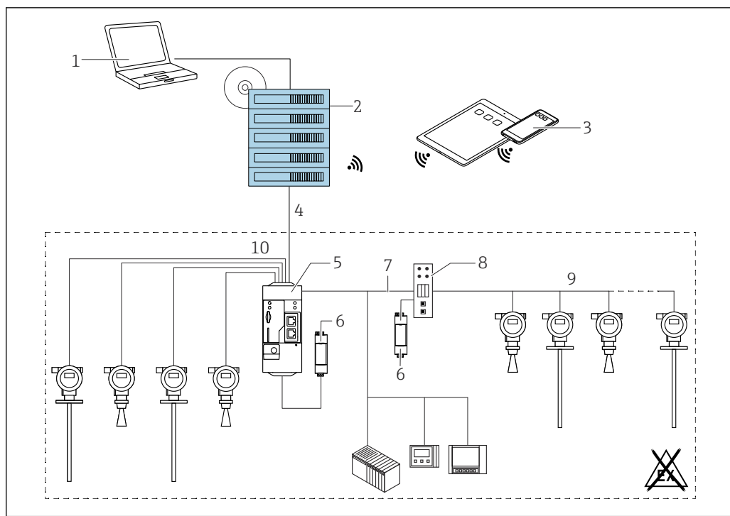
23 Exemple de plateforme de gestion des stocks avec SupplyCare Enterprise SCE30B
