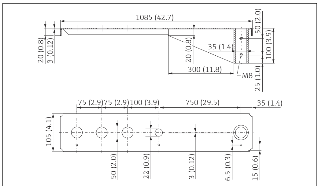
33 Dimensions. Unité de mesure mm (in)
