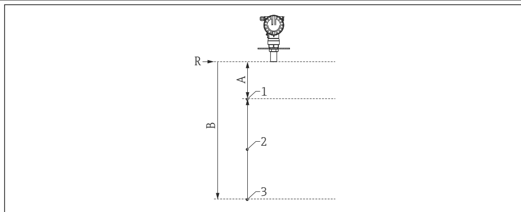
28 Exemplo de protocolo de linearidade de 3 pontos
