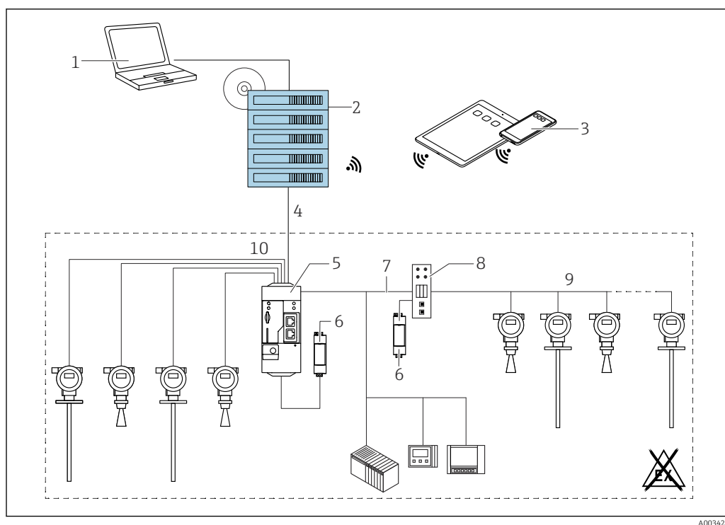
26 Exemplo de plataforma de gerenciamento de inventário com a SupplyCare Enterprise SCE30B
