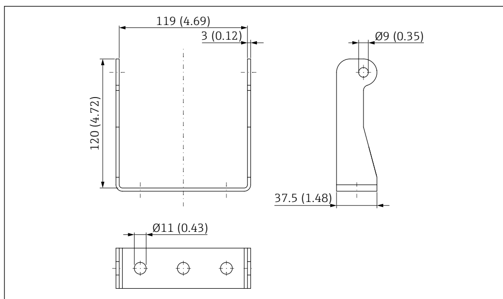
20 Suporte de montagem. Unidade de medida mm (in)
