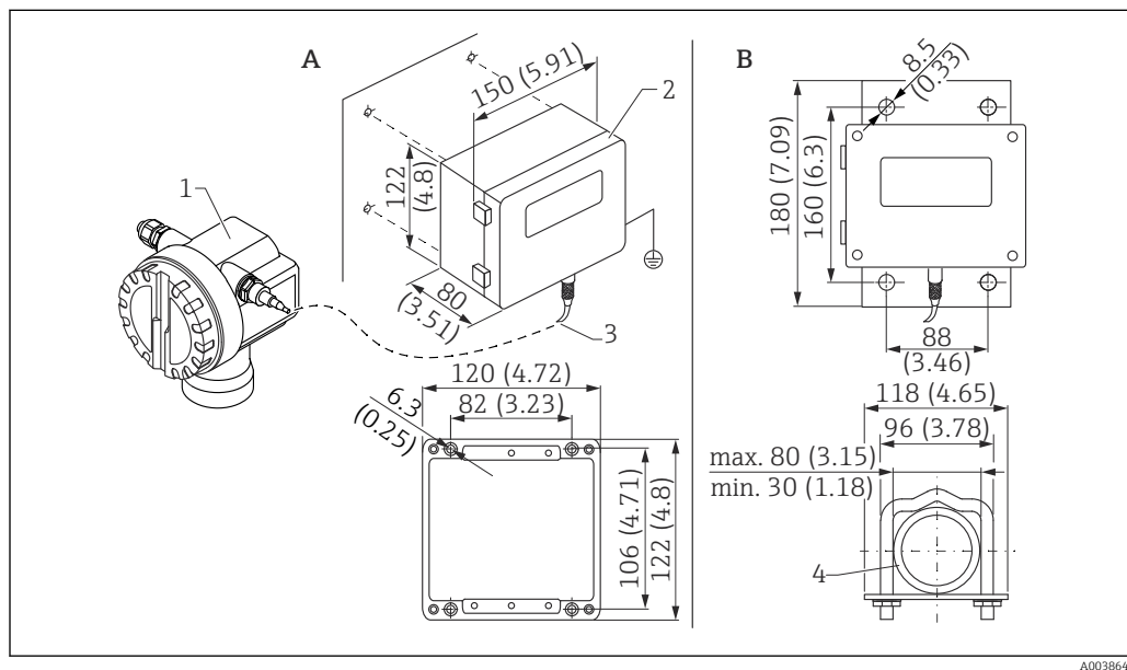
29 Indicador remoto. Unidad de medida mm (in)
