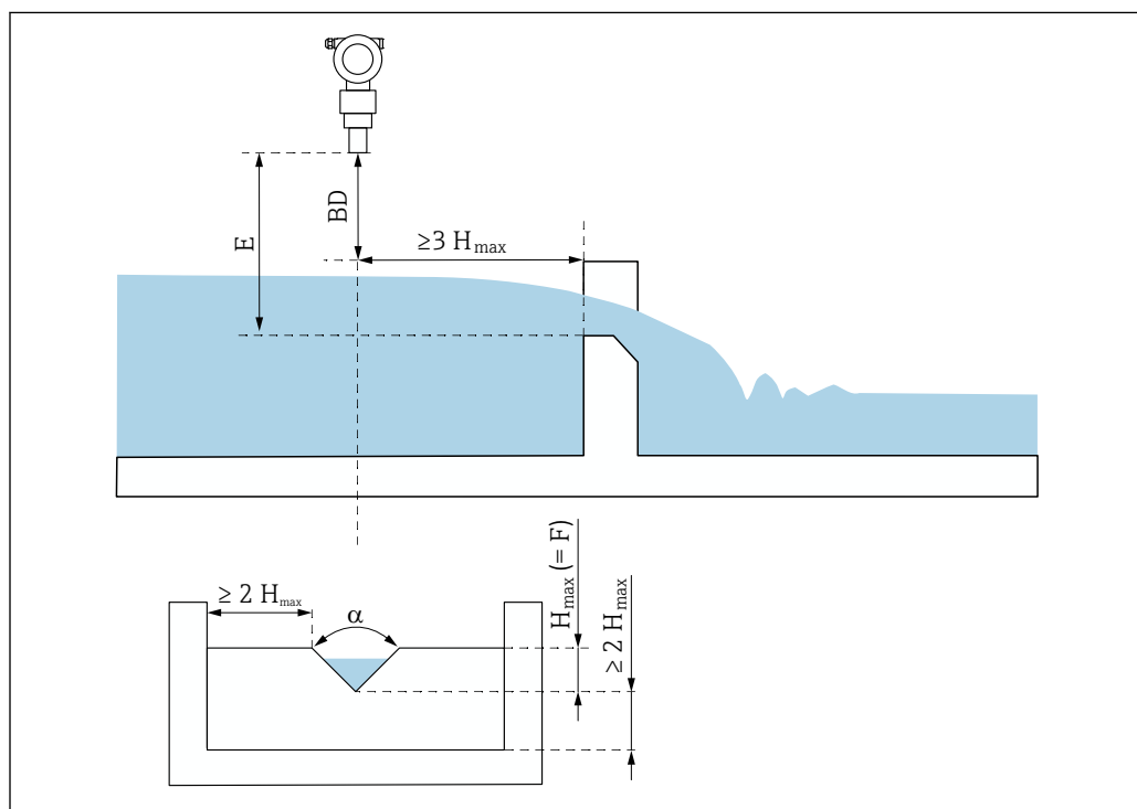
8 Vertedero triangular (ejemplo)
