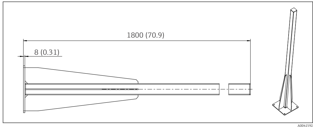
12 Palina (accessorio) per versione "outdoor", dimensioni in mm (inch)
