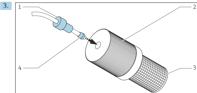
56 Montaggio del filtro di aspirazione (fornito) sul tubo flessibile di prelievo
