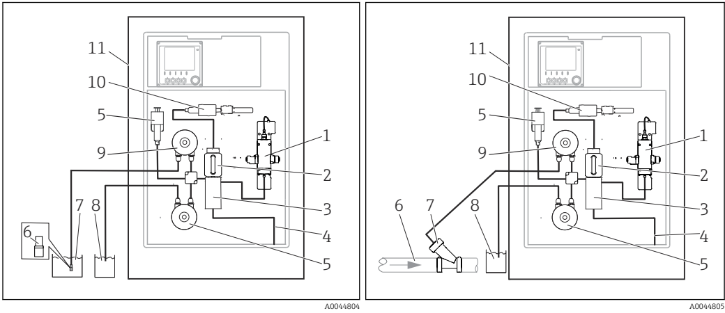
2 Sistema di misura con Liquiline System CA80COD e filtro di aspirazione
