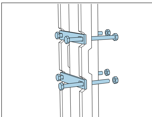
19 Analizzatore montato su palina (vista frontale)
