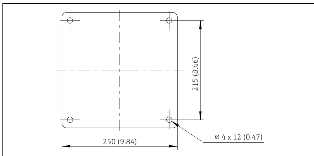
18 Piano di fondazione, dimensioni in mm (in)
