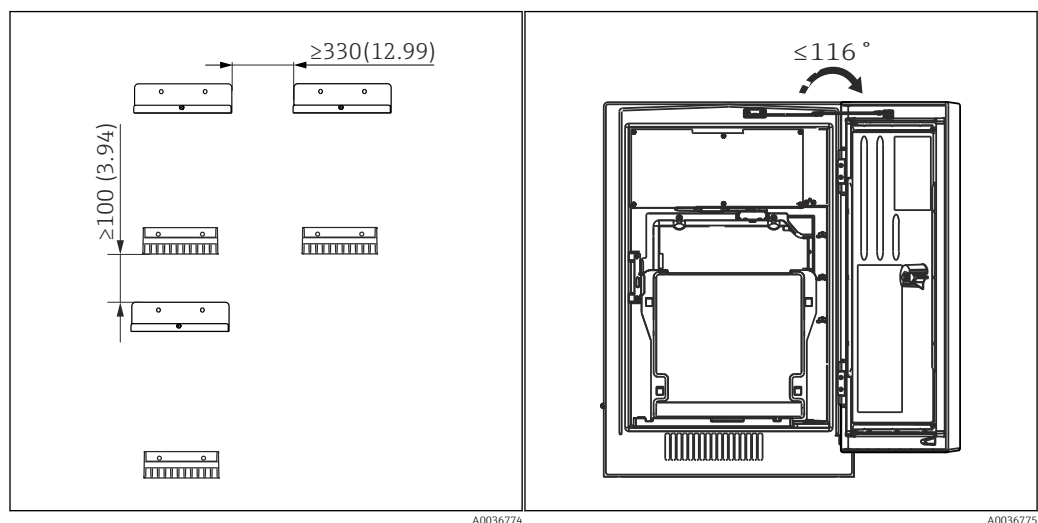
13 Spaziatura minima richiesta per il montaggio. Unità ingegneristica mm (in). 14 Angolo di apertura massimo
