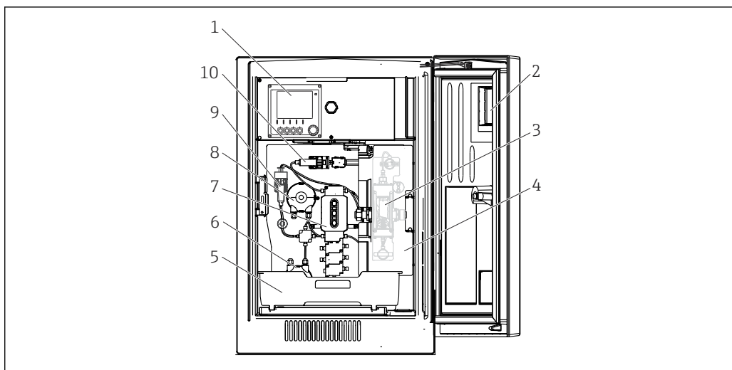
1 Esempio di Liquiline System CA80
