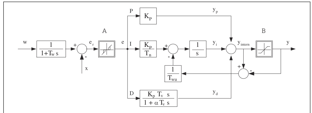
67 Diagramma a blocchi della struttura del controllore
