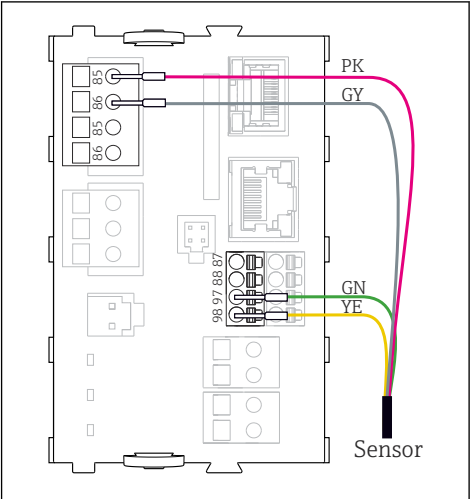
11 传感器，连接附加电源
