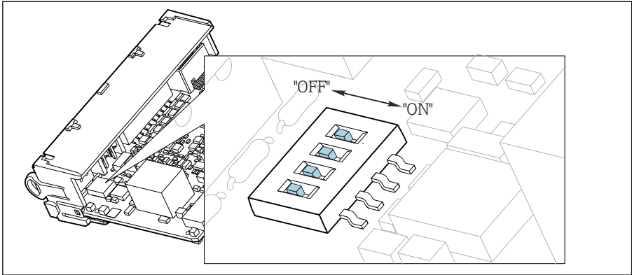
图 30 内部端接的 DIP 开关
