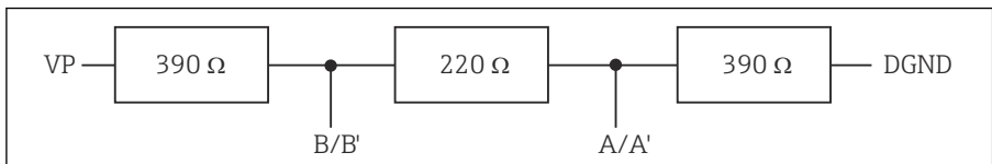
图 31 内部端接示意图
