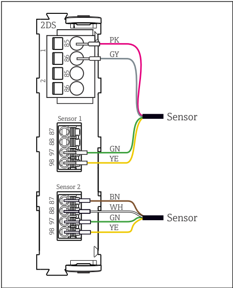
12 传感器，连接/不连接传感器模块 2DS 处的附加电源
