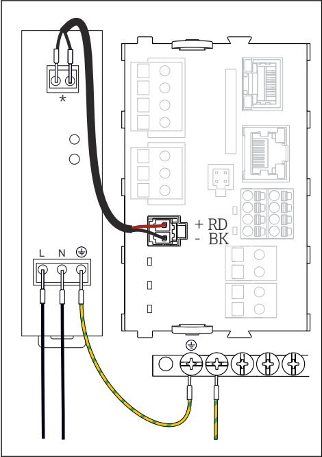
图 7 BASE2-E 模块的电源接线示意图
