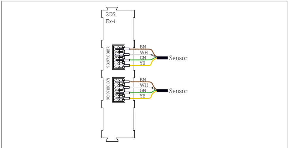
图 13 传感器和本安 Ex-i 型传感器通信模块 2DS，不带附加电源
