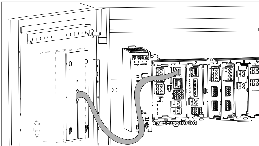
图 4 安装到位的显示单元
