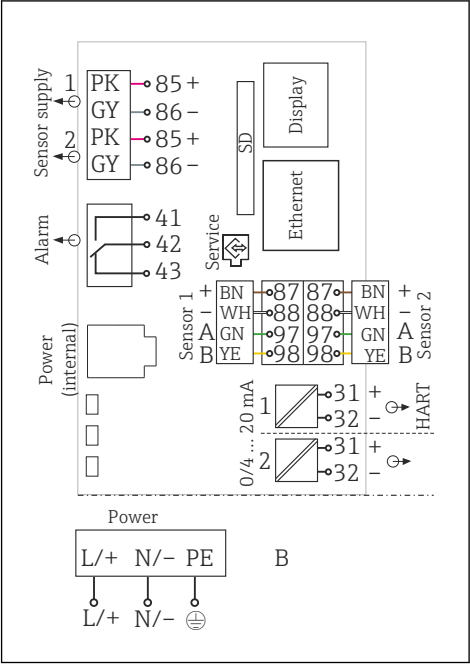
图 8 BASE2-E 模块和外接供电单元 (B) 的完整接线图
