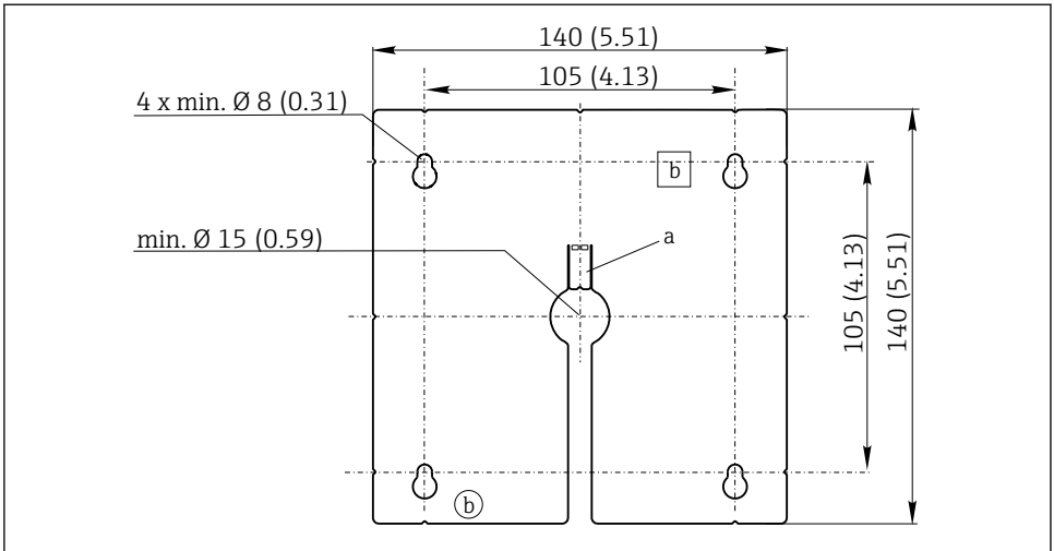
图 3 外接显示单元的安裝背板的外形尺寸；单位：mm (in)
