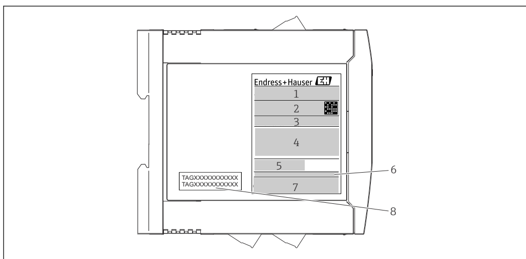
2 Etiqueta de identificação do transmissor do trilho DIN (exemplo, versão Ex)
