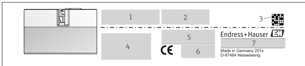
1 Etiqueta de identificação do transmissor compacto (exemplo, versão Ex)
