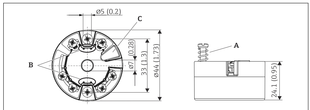
20 Versão com terminais de parafuso
