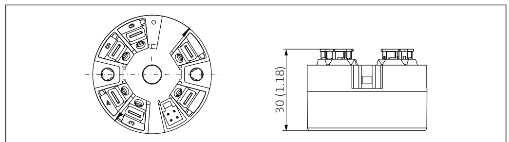
21 Versão com terminais push-in. Dimensões são idênticas à versão com terminais de parafuso, com exceção da altura do invólucro.
