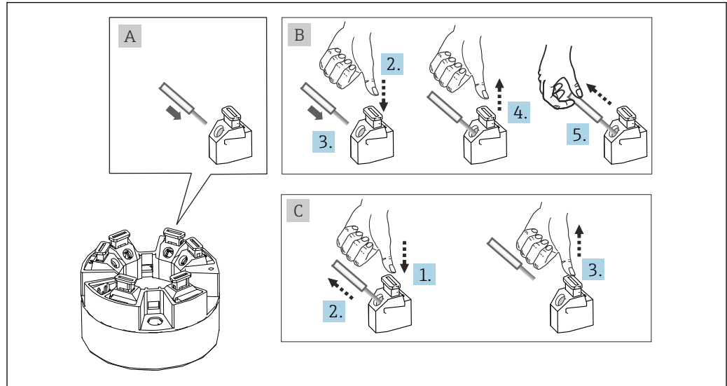
11 Conexão ao terminal de mola, usando o exemplo de um transmissor compacto
