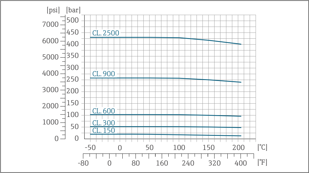
29 法兰材质: C22 2.4602 (UNS N06022) 合金
