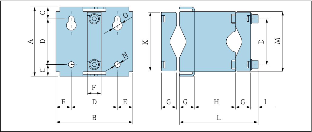
传感器安装支座
