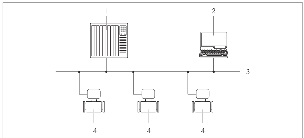
图 51 通过 PROFIBUS DP 网络进行远程操作
