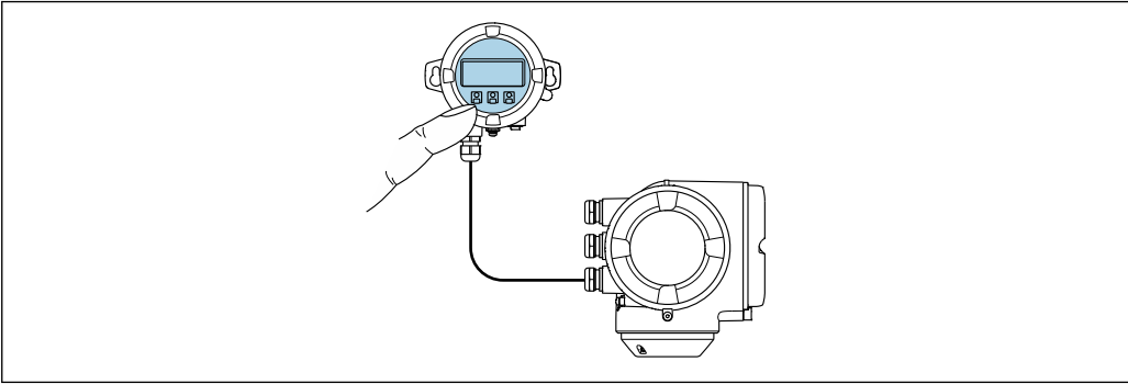
47 通过远传显示单元 DKX001 操作
