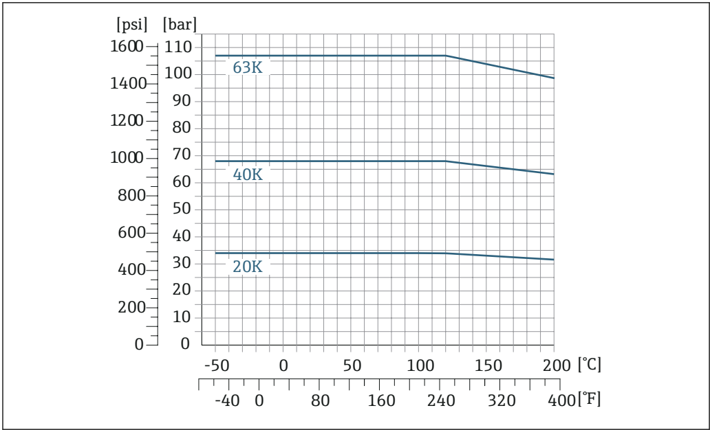
图 31 法兰材质: 1.4404 (316/316L) 、C22 2.4602 (UNS N06022) 合金
