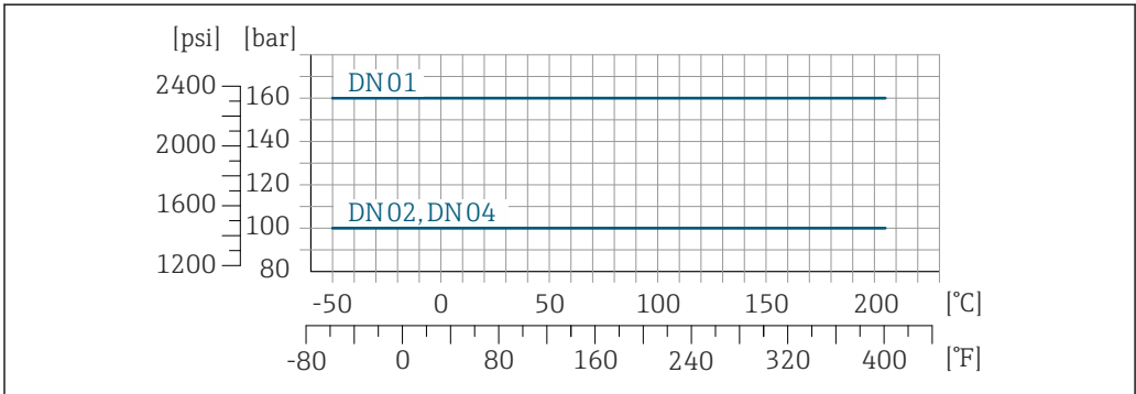
图 33 法兰材质: 1.4404 (316/316L)
