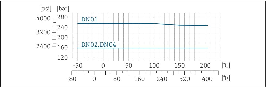
34 法兰材质: C22 2.4602 (UNS N06022) 合金
