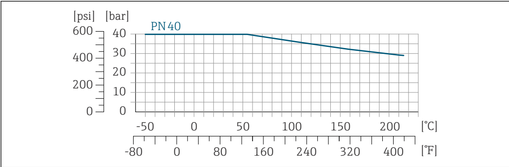
27 松套法兰材质: 1.4301 (F304) ; 接液部件材质: C22 2.4602 (UNS N06022) 合金
