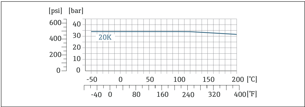
图 32 松套法兰材质: 1.4301 (F304) ; 接液部件材质: C22 2.4602 (UNS N06022) 合金
