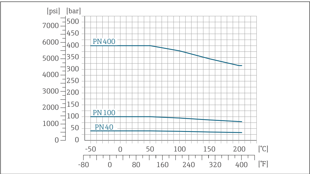
图 25 法兰材质: 1.4404 (316/316L)
