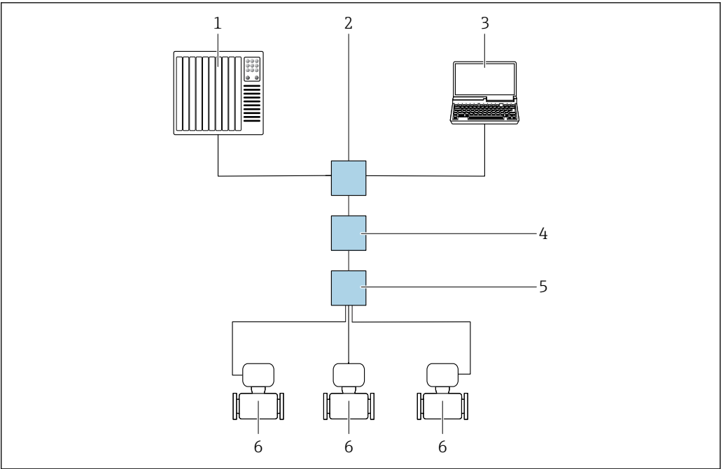
图 58 通过 APL 网络进行远程操作
