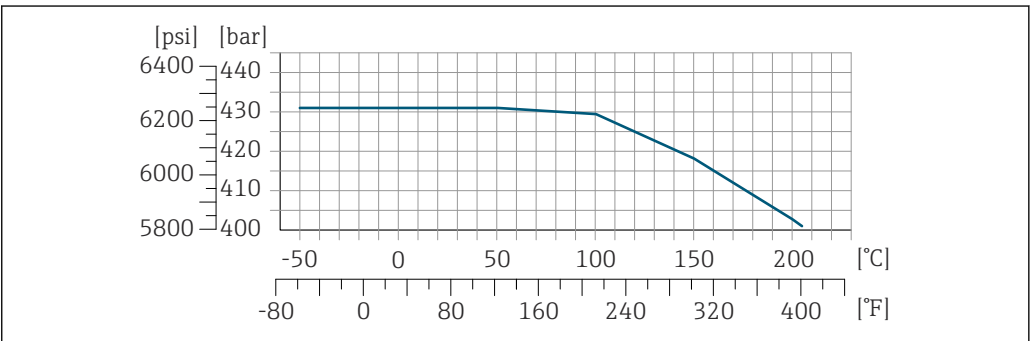
35 法兰材质: C22 2.4602 (UNS N06022) 合金; 订购选项“测量管材质; 接液部件表面”, 选型代号 HB
