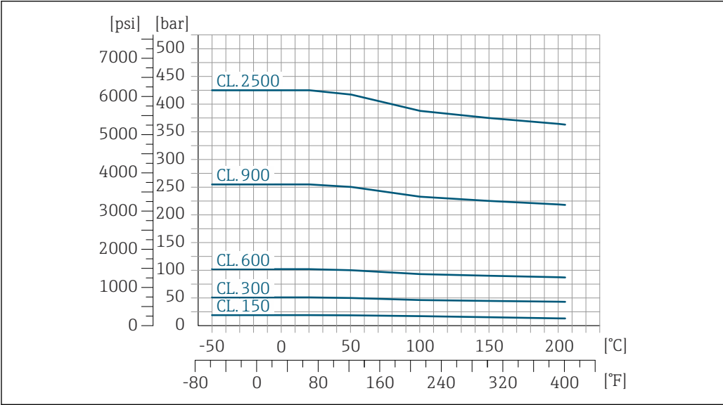
28 法兰材质: 1.4404 (316/316L)
