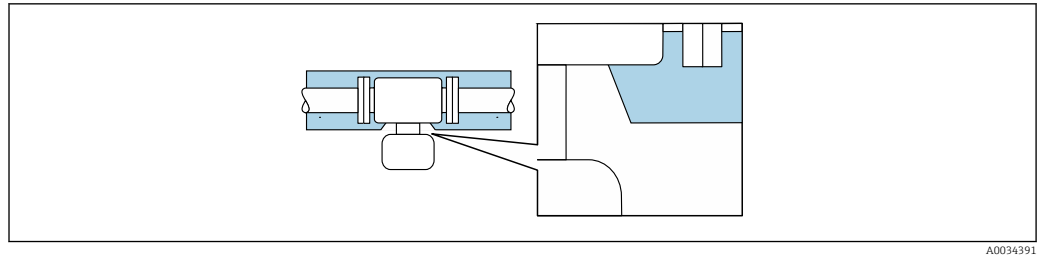
6 Isolamento térmico com pescoço de extensão não isolado
