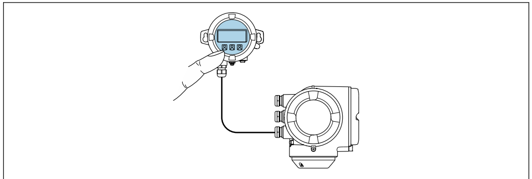
41 Operação através do display remoto e do módulo de operação DKX001
