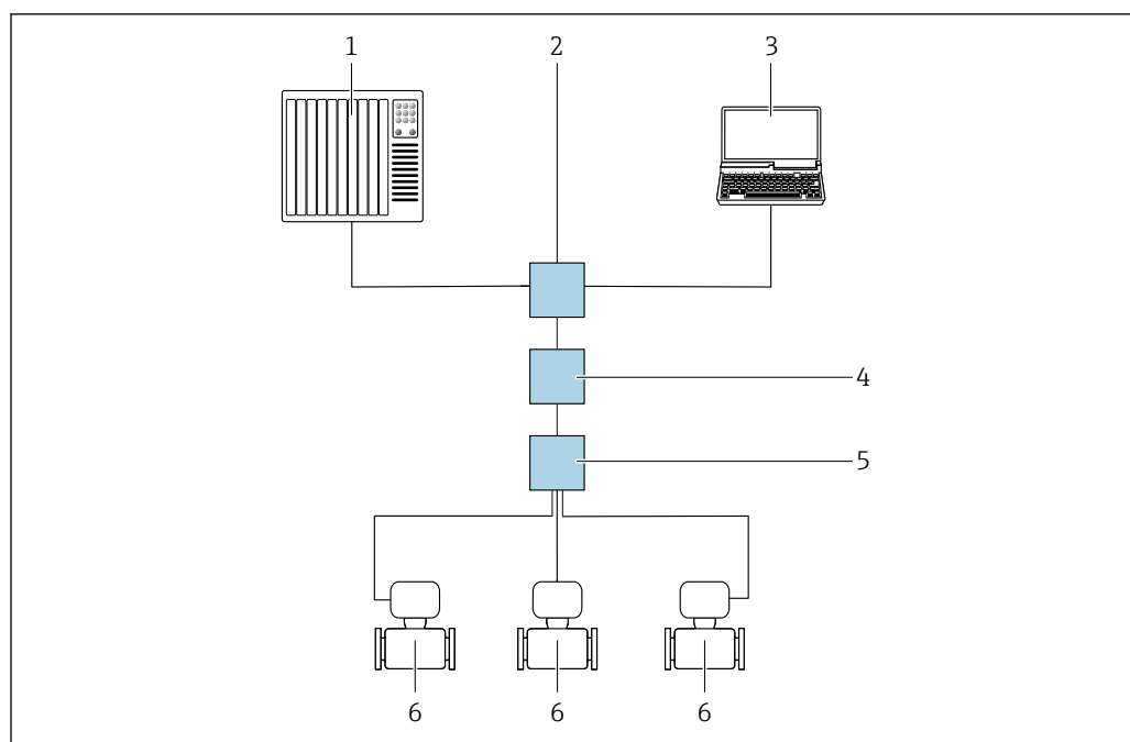
图 62 通过 APL 网络进行远程操作
