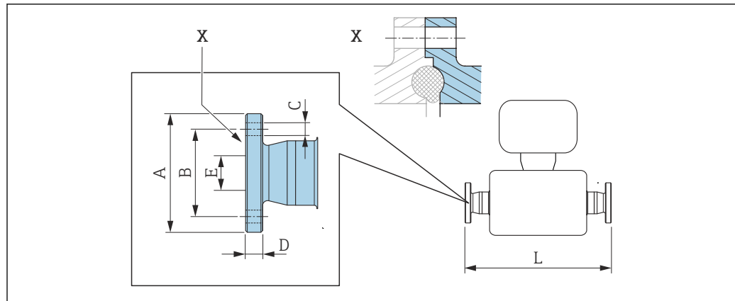
图 39 视图 X: 非对称过程连接; 蓝色部分由供应商提供。
