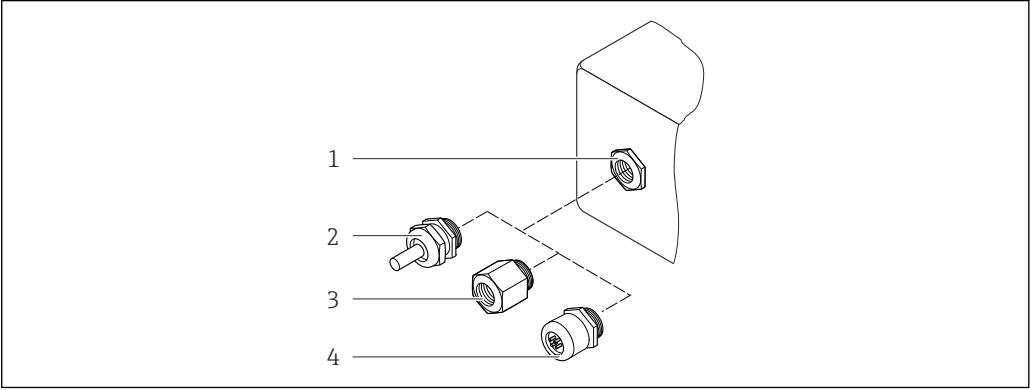
图 49 允许的电缆入口/缆塞
