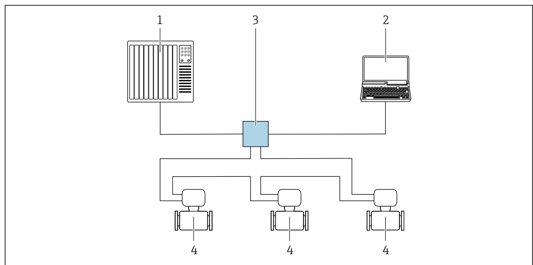
图 50 通过 PROFINET 网络进行远程操作：环形拓扑结构
