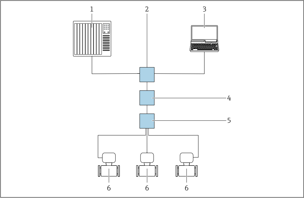
51 通过 APL 网络进行远程操作
