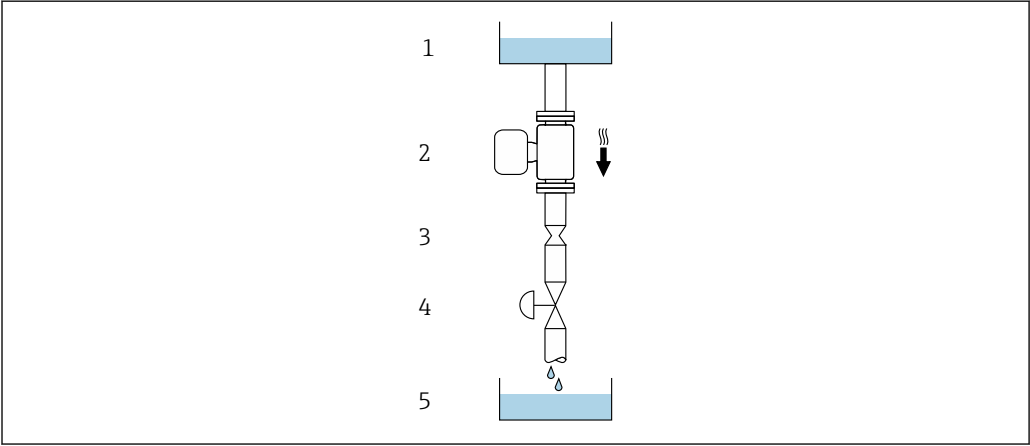
22 安装在竖直向下管道中（例如批处理应用）
