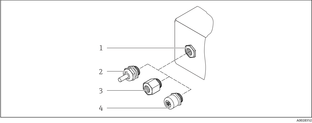
图 38 允许的电缆入口/缆塞 1 内螺纹 M20 × 1.5 2 缆塞 M20 × 1.5 3 转接头，适用 G ½"或 NPT ½"内螺纹电缆入口 4 设备插头
