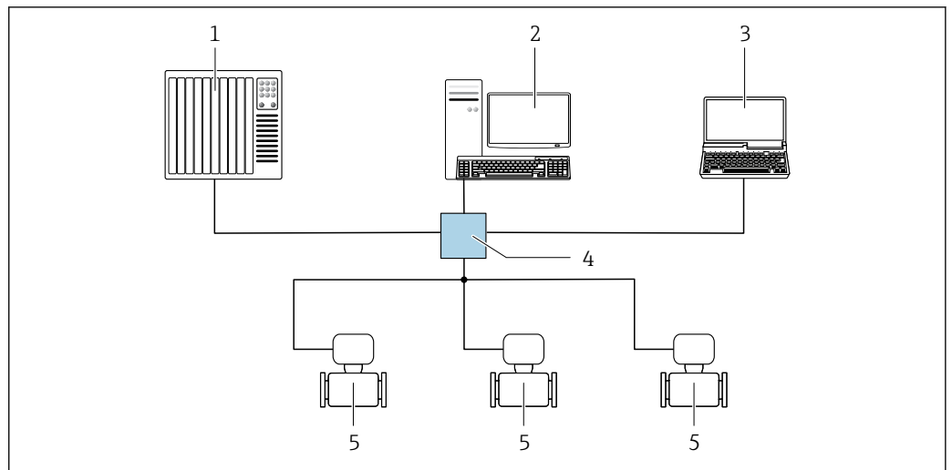
图 47 通过 EtherNet/IP 网络进行远程操作：星形拓扑结构
