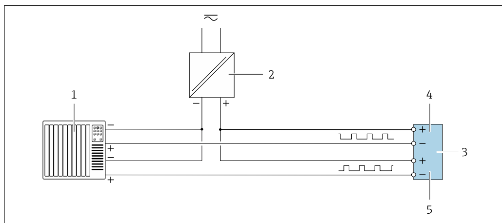
18 接线实例：双脉冲输出（无源信号）
