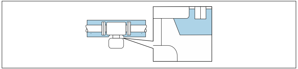
图 29 保温层延长颈裸露
