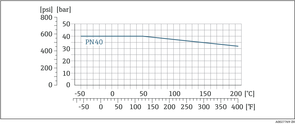
图 26 法兰材质: 1.4301 (304) ; 接液部件材质: 锆 702、钽
