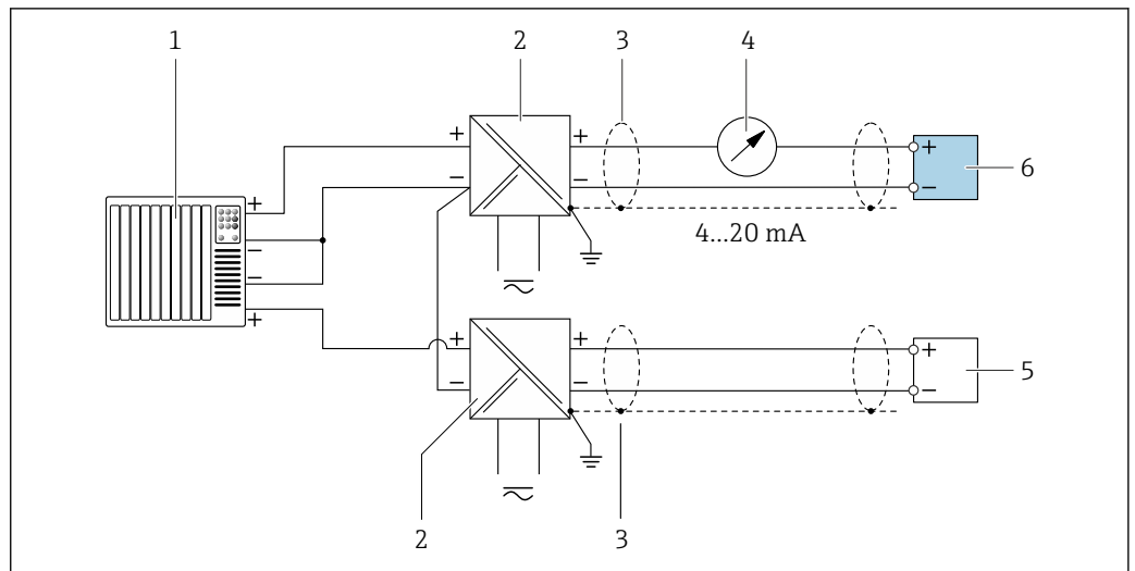
4 接线实例：HART 输入，公共端接负极（无源信号）
