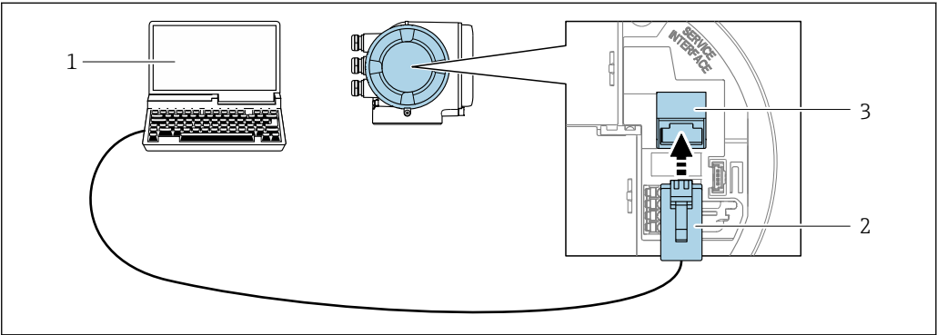
52 通过服务接口（CDI-RJ45）连接
